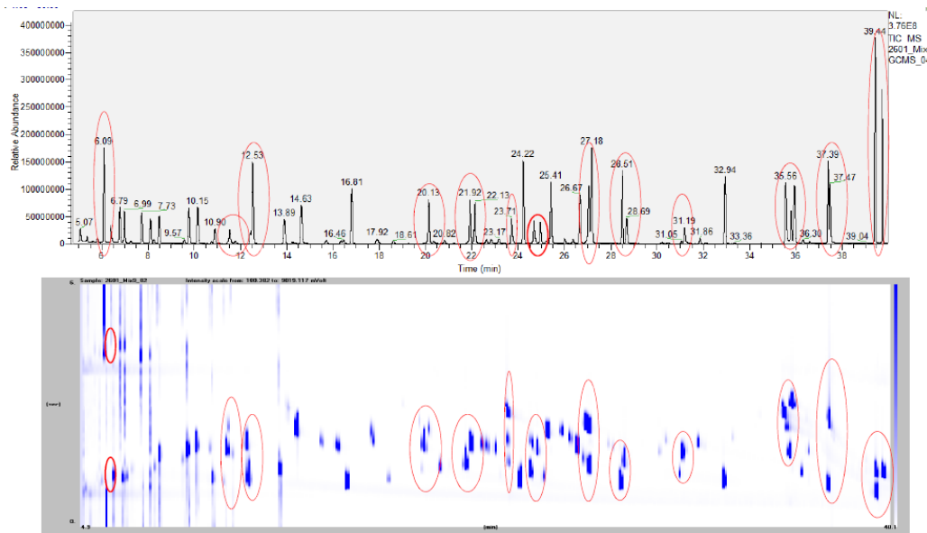
Abbildung 31 GC- (oben) und 2xGC-Chromatogramme (unten) derselben Gasprobe. Von 18 Spitzen des GC-Fragmentierungsmusters können 14 mit der zweiten Dimension des 2xGC (in der Abbildung rot hervorgehoben) fragmentiert werden. Nach (Vial et al., 2016).
