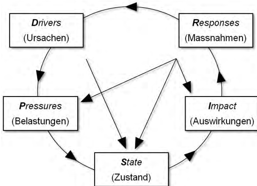
Abb. 3: Das DPSIR-Modell.
