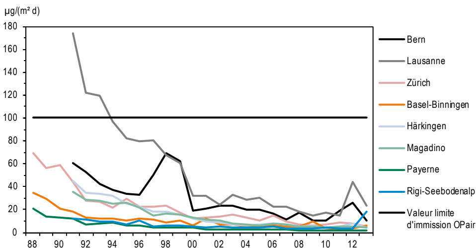
Figure 41 > Plomb dans les retombées de poussières, moyennes annuelles de 1988 à 2013
