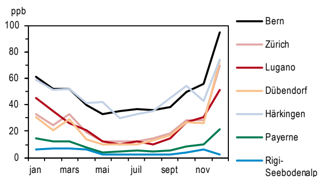
Figure 12 > Oxydes d'azote (NO x ), moyennes mensuelles par type de station, 2013
