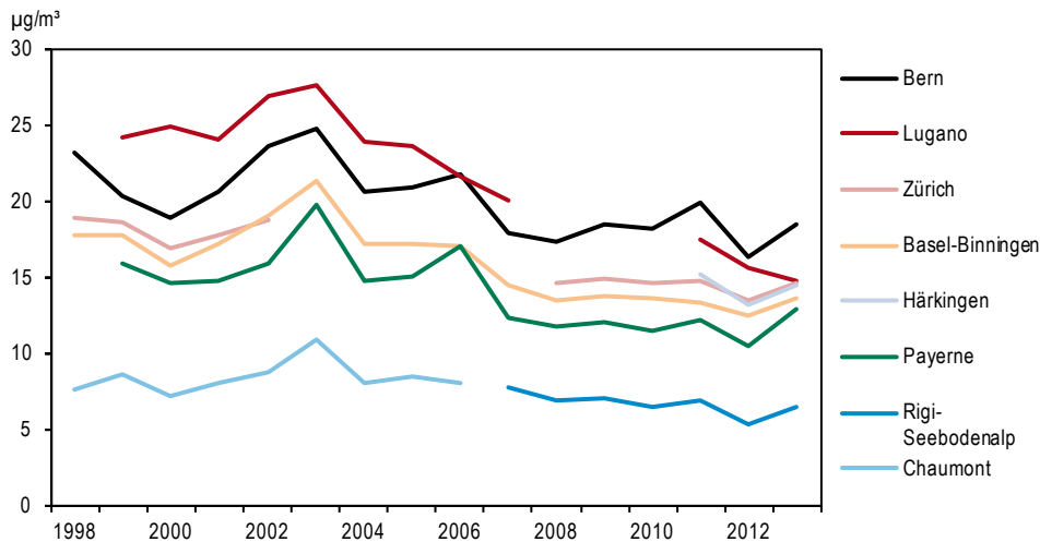
Figure 17 > Poussières fines (PM 2,5 ), moyennes annuelles 1991–2013
