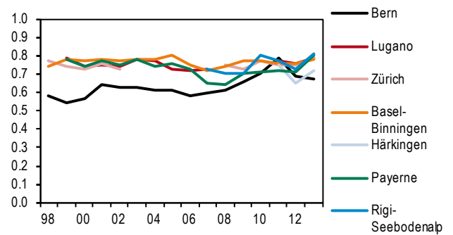
Figure 19 > Verhältnis der Jahresmittel PM 2,5 /PM 10 1998–2013
