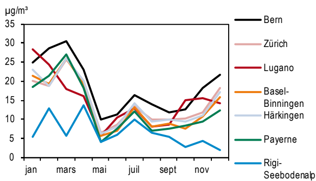
Figure 18 > Poussières fines (PM 2,5 ), moyennes mensuelles, 2013
