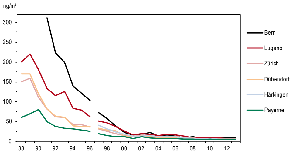
Figure 40 > Plomb dans les poussières fines (PM10, avant 1997, TSP), moyennes annuelles de 1988 à 2013 (valeur limite d'immission OPair: 500 ng/m 3 )
