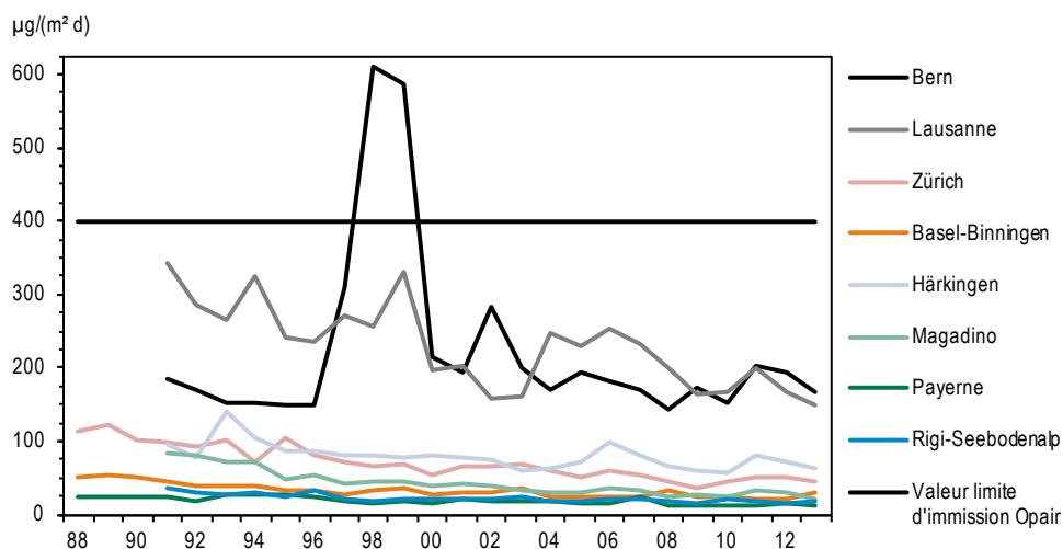
Figure 44 > Zinc dans les retombées de poussières, moyennes annuelles de 1988 à 2013
