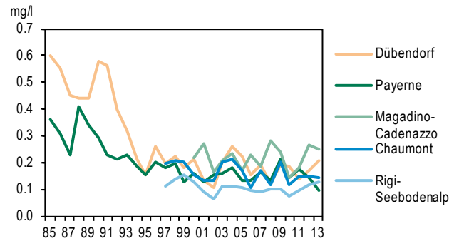
Figure 48 > Chlorure (Cl - ) des eaux de pluie, moyennes annuelles de 1985 à 2013
