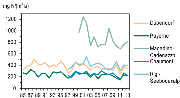
Figure 53 > Nitrate ( \text{NO}_3^-\text{-N} ), moyennes annuelles des charges de 1985 à 2013
