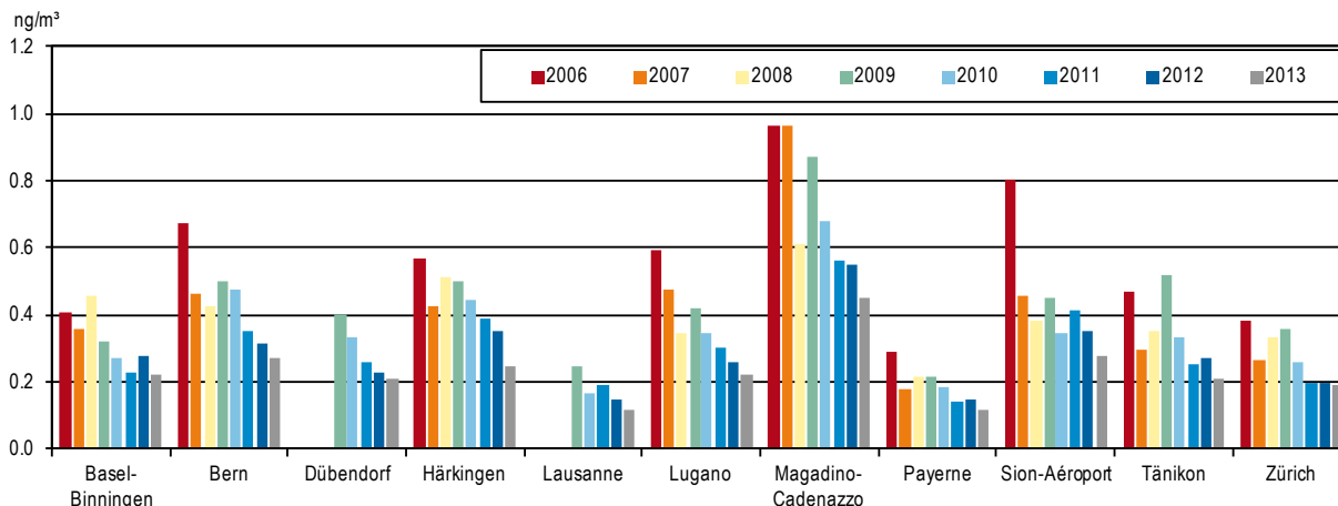
Figure 22 > Moyennes annuelles des concentrations de benzo(a)pyrène dans les PM10
