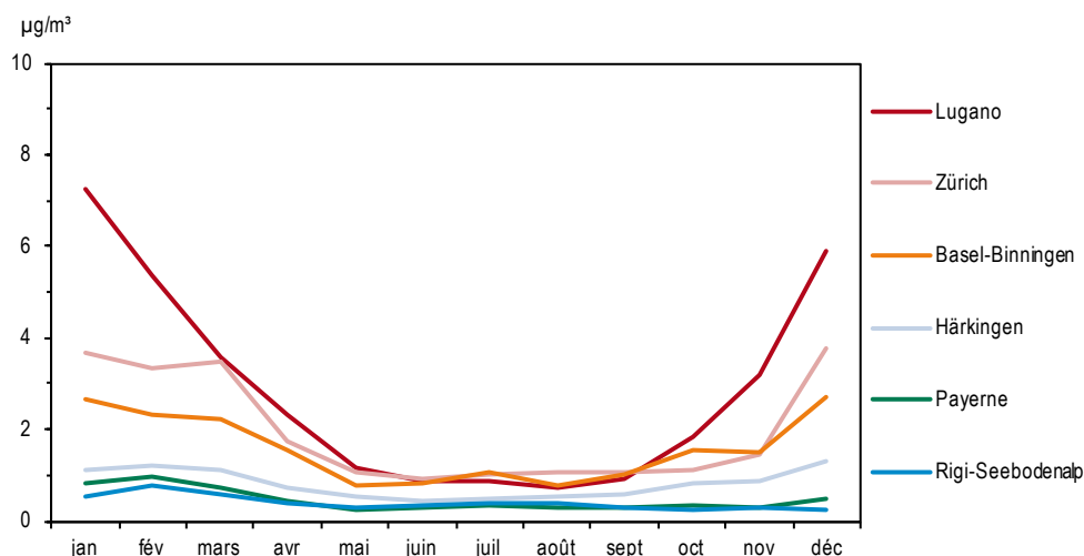
Figure 35 > Dioxyde de soufre (SO 2 ), moyennes mensuelles 2013
