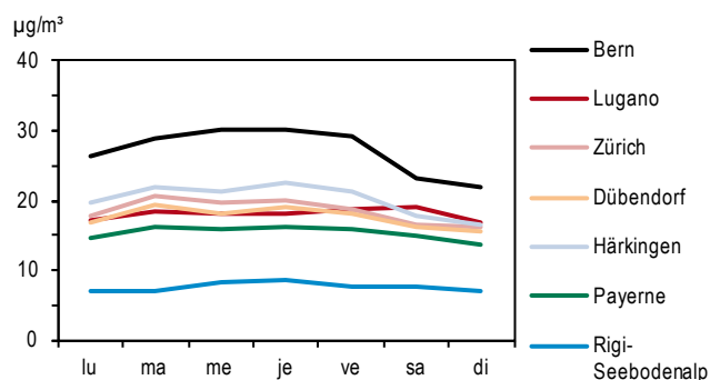
Figure 16 > Fluctuations hebdomadaires moy. des PM10 en 2013
