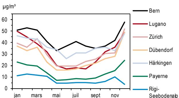
Figure 10 > Dioxyde d'azote (NO 2 ), moyennes mensuelles, 2013
