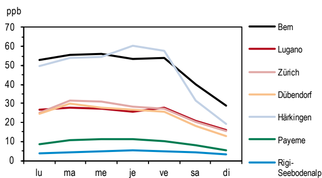
Figure 13 > Oxydes d'azote (NO x ), fluctuations hebdomadaires, 2013
