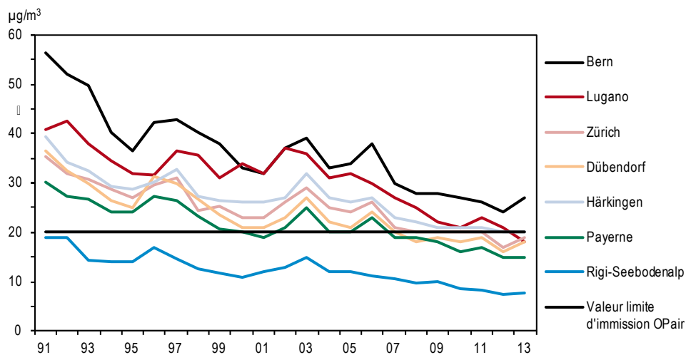
Figure 14 > Poussières fines (PM10), moyennes annuelles 1991–2013
