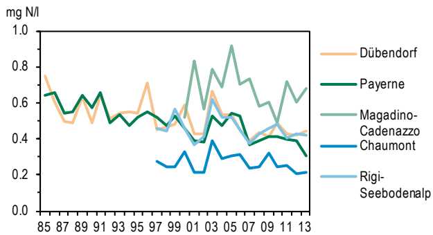
Figure 49 > Ammonium (NH 4 + -N) des eaux de pluie, moyennes annuelles de 1985 à 2013
