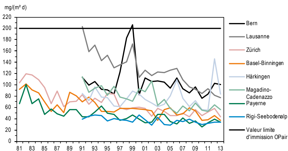
Figure 39 > Retombées de poussières, moyennes annuelles de 1981 à 2013
