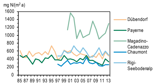
Figure 54 > Ammonium ( \text{NH}_4^+\text{-N} ), moyennes annuelles des charges de 1985 à 2013
