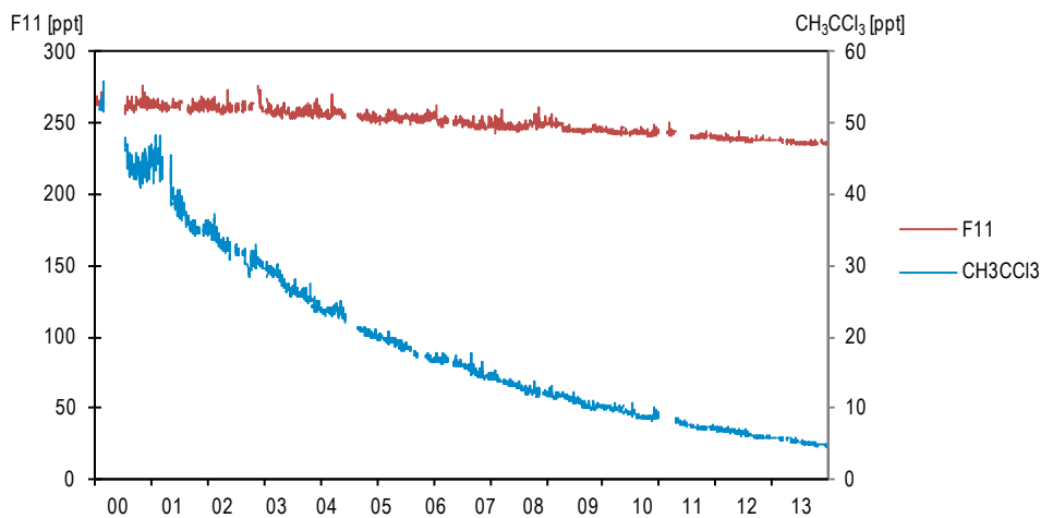
Figure 33 > 1,1,1-Trichloréthane et F11: moyennes journalières de 2000 à 2013 sur la Jungfraujoch
