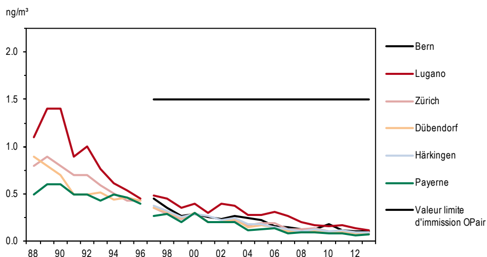
Figure 42 > Cadmium dans les poussières fines (PM10, avant 1997, TSP), moyennes annuelles de 1988 à 2013
