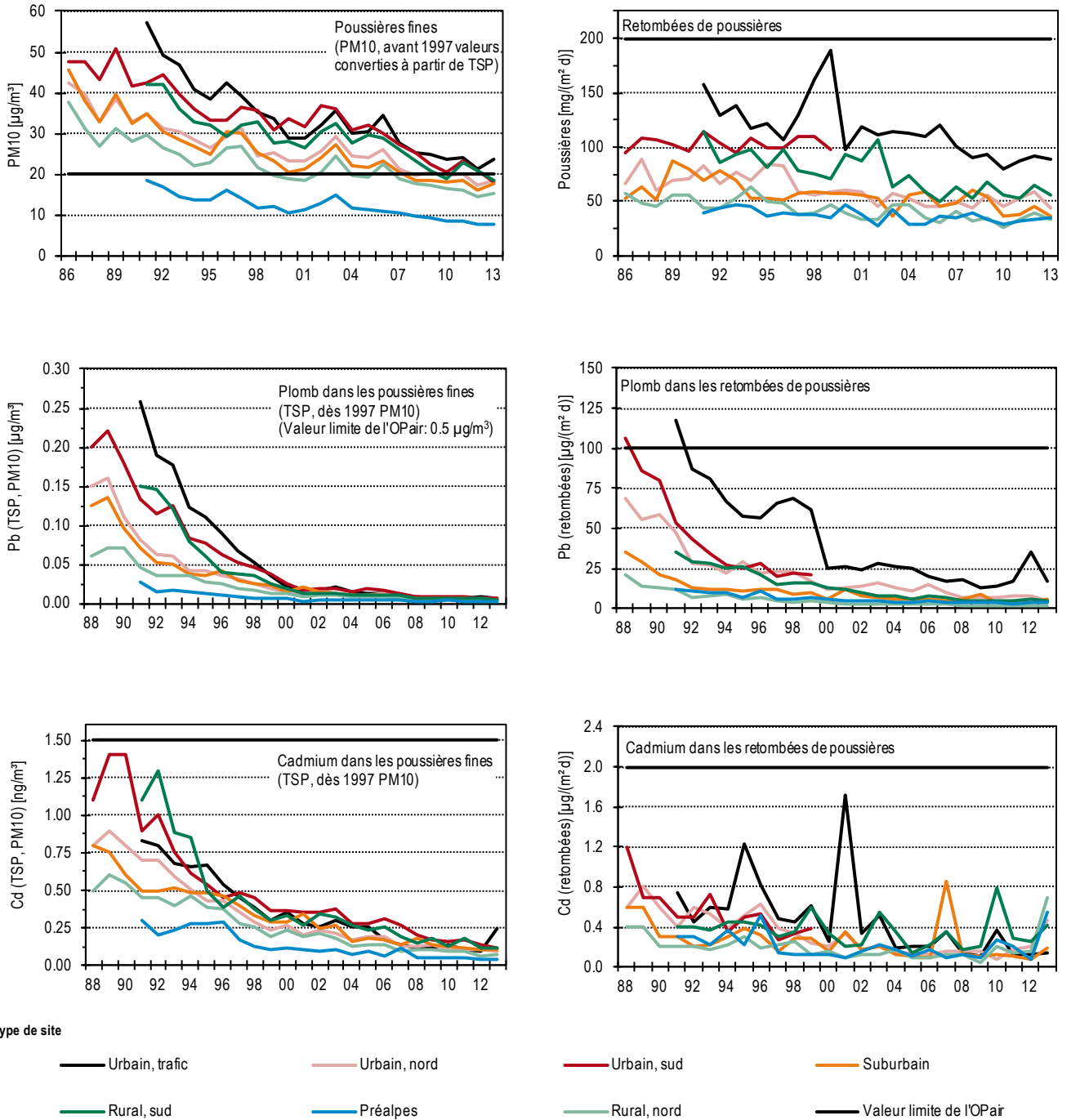
Figure 2 > Evolution de 1986 à 2013 des polluants suivants (moyennes annuelles): poussières fines (PM10; valeurs avant 1997 converties à partir de mesures TSP), retombées de poussières, plomb et cadmium (dans les poussières fines et les retombées de poussières) en différents emplacements
