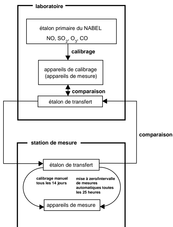
Figure 6 > Traçabilité pour quatre substances: SO 2 , NO, O 3 et CO
