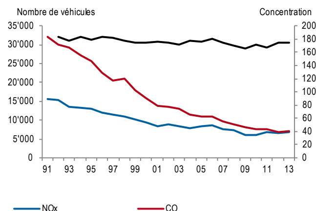
Figure 60 > volume de trafic et concentration de polluants, 1991 – 2013, Lausanne-César-Roux
