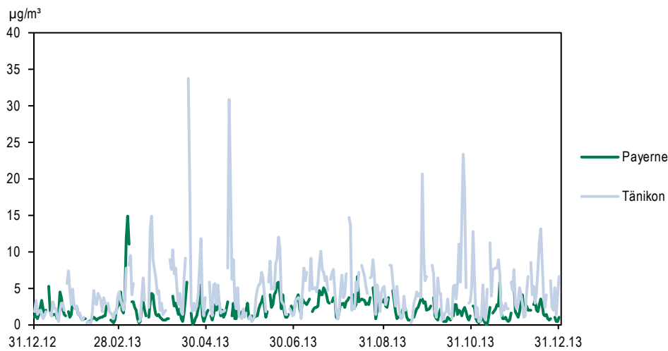
Figure 57 > Valeurs moyennes journalières des concentrations d'ammoniac, 2013
