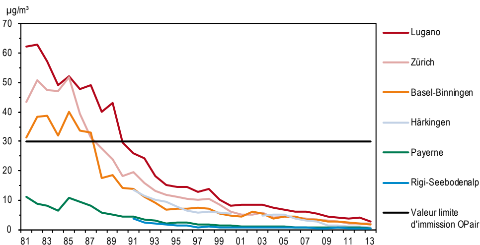
Figure 34 > Dioxyde de soufre ( \text{SO}_2 ), moyennes annuelles de 1981 à 2013
