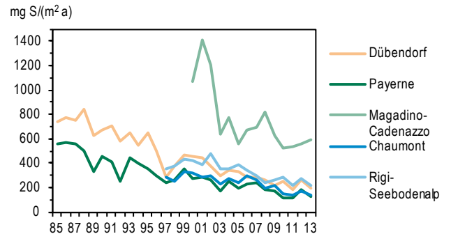
Figure 52 > Sulfate ( \text{SO}_4^{2-}\text{-S} ), moyennes annuelles des charges de 1985 à 2013
