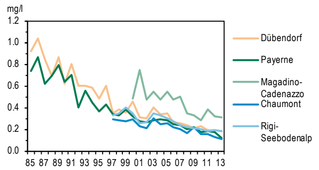
Figure 46 > Sulfate (SO 4 2- -S) des eaux de pluie, moyennes annuelles de 1985 à 2013
