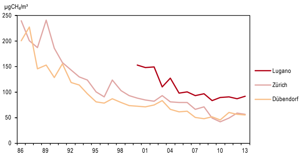
Figure 29 > COV non méthaniques (exprimés en équivalent méthane), moyennes annuelles de 1986 à 2013
