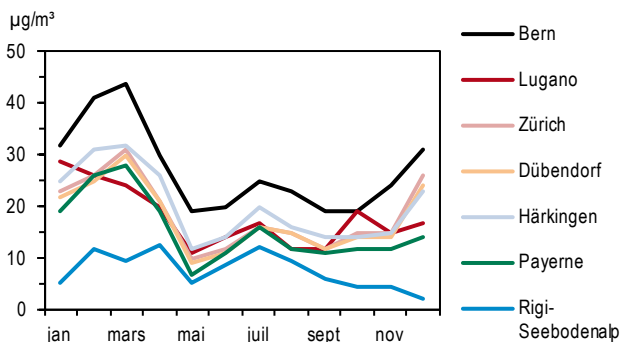
Figure 15 > Poussières fines (PM10), moyennes mensuelles, 2013
