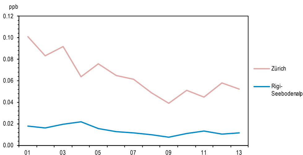
Figure 31 &gt; 1,3-butadiène, moyennes annuelles de 2001 à 2013
