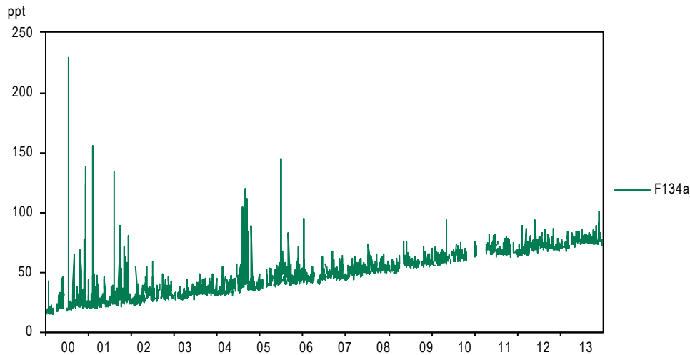
Figure 32 > F134a, moyennes journalières de 2000 à 2013 sur la Jungfraujoch
