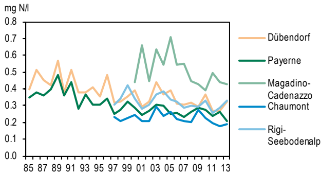
Figure 47 > Nitrate (NO 3 - -N) des eaux de pluie, moyennes annuelles de 1985 à 2013
