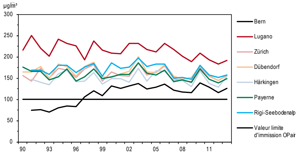
Figure 25 > Ozone, valeur 98 % du mois d'été le plus chargé en ozone, de 1990 à 2013
