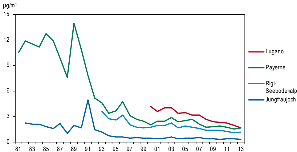
Figure 21 > Sulfate dans les PM10, valeurs moyennes annuelles 1981–2013
