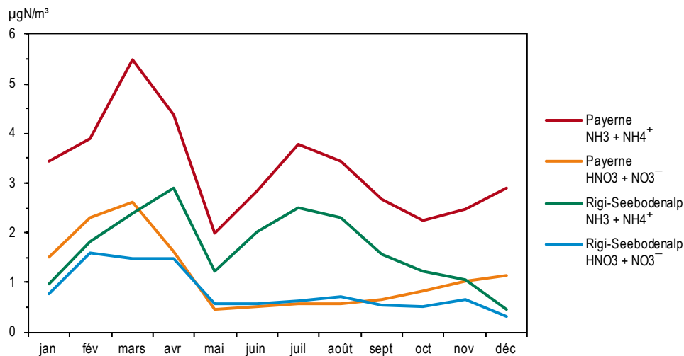
Figure 56 > Quantité totale de composés azotés, moyennes mensuelles 2013 (Payerne et Rigi-Seebodenalp)
