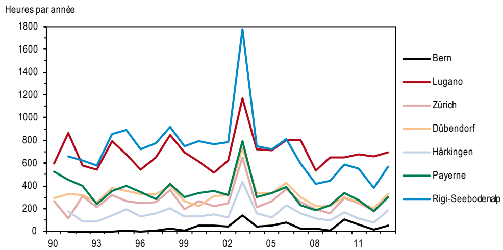
Figure 26 > Ozone, nombre de dépassements de la valeur limite horaire d'immission, de 1990 à 2013
