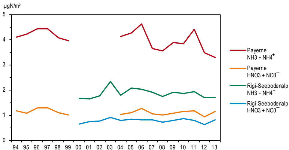
Figure 55 > Quantité totale de composés azotés, moyennes annuelles de 1994 à 1999 et de 2004 à 2013 (Payerne) et de 2000 à 2013 (Rigi-Seebodenalp)
