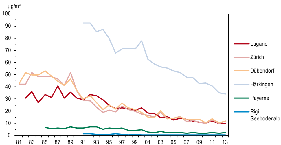
Figure 8 > Monoxyde d'azote (NO), moyennes annuelles de 1981 à 2013
