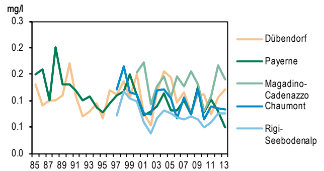
Figure 50 > Sodium (Na + ) des eaux de pluie, moyennes annuelles de 1985 à 2013
