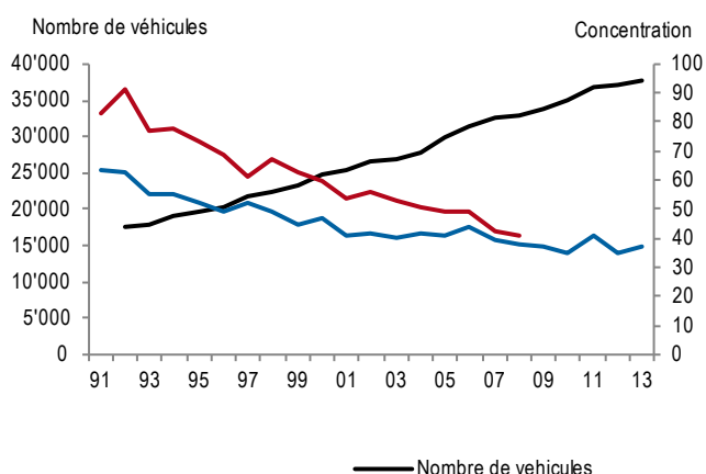
Figure 59 > volume de trafic et concentration de polluants, 1991 – 2013, Sion-Aéroport
