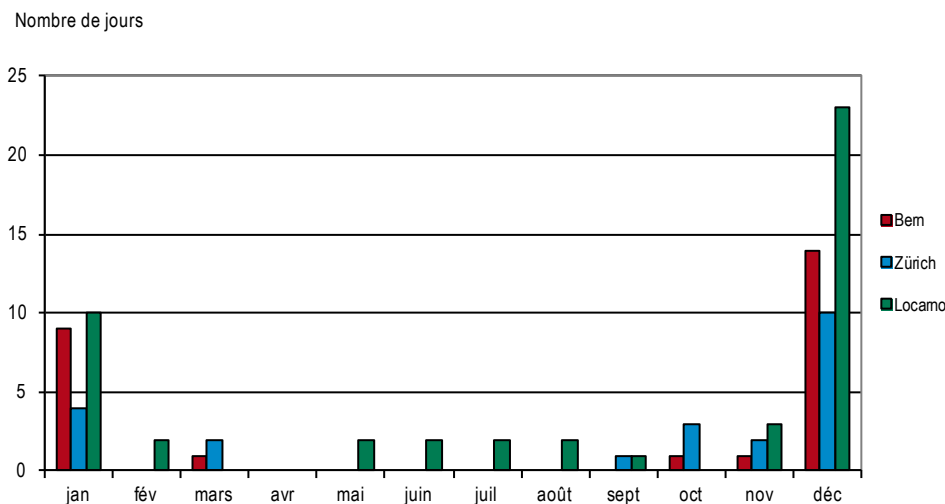
Figure 58 > Nombre de jours par mois avec inversion de la température entre 12 et 14 h HEC (soit au minimum une isothermie, c'est-à-dire la même température pour la station de montagne et celle de plaine)
