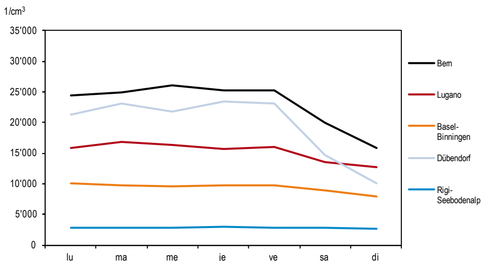
Figure 20 > Concentration en nombre de particules, fluctuations hebdomadaires moyennes, 2013
