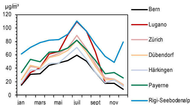
Figure 27 > Ozone, moyennes mensuelles par type de station, 2013
