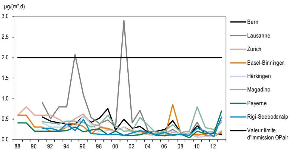
Figure 43 > Cadmium dans les retombées de poussières, moyennes annuelles de 1988 à 2013
