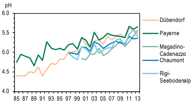
Figure 45 > Valeur de pH des eaux de pluie, moyennes annuelles de 1985 à 2013
