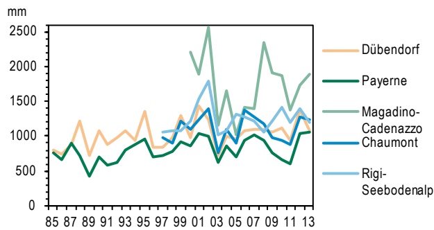
Figure 51 > Taux de précipitations analysé, somme des années 1985 à 2013
