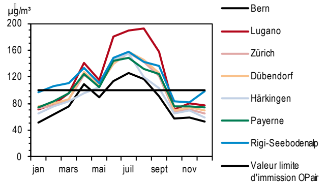
Figure 28 > Ozone, valeurs 98 % mensuelles par type de station, 2013
