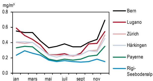
Figure 37 > Monoxyde de carbone (CO), moyennes mensuelles, 2013
