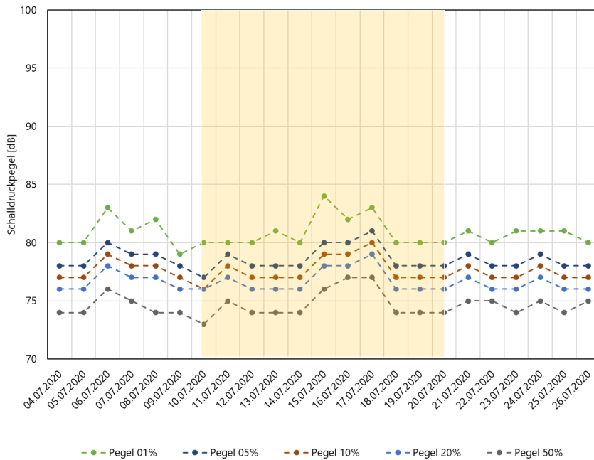
Abbildung 16: Tageweise ausgewertete Schalldruckpegelperzentilwerte für die PW-Ereignisse am Messpunkt 2. Gelb unterlegt ist die Periode mit eingeschaltetem Display.
