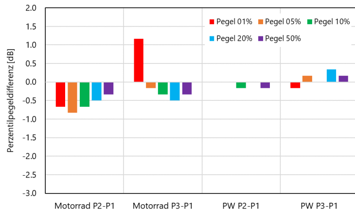
Abbildung 25: Perzentilpegeldifferenzen (1, 5, 10, 20, 50%) am Messpunkt 1 für die beiden Kategorien Motorräder und PW. P2-P1 steht für Phase 2 minus Phase 1, P3-P1 ist Phase 3 minus Phase1.
