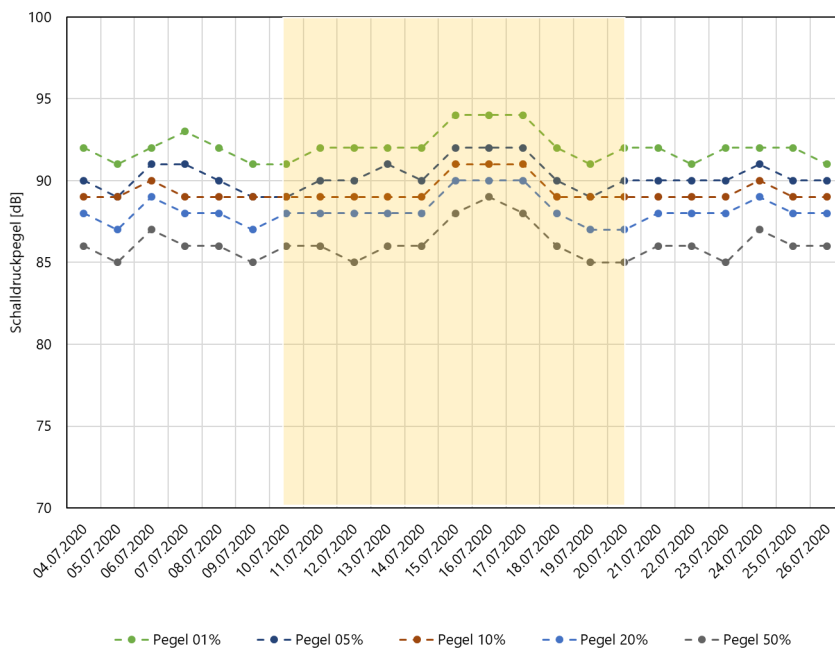
Abbildung 14: Tageweise ausgewertete Schalldruckpegelperzentilwerte für die PW-Ereignisse am Messpunkt 1. Gelb unterlegt ist die Periode mit eingeschaltetem Display.
