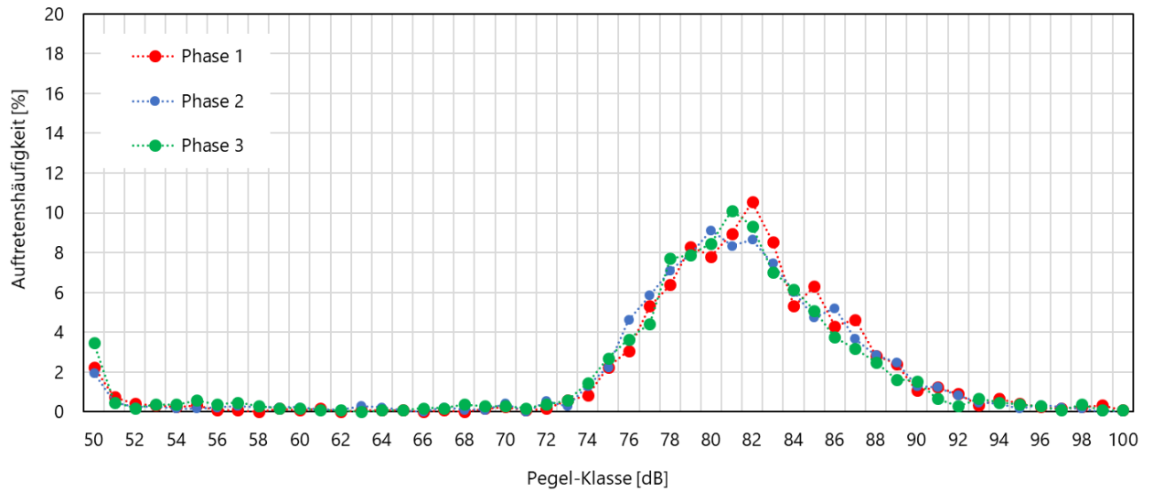
Abbildung 23: Phasenaufgeschlüsselte Pegelverteilung der Motorradereignisse am Messpunkt 3.
