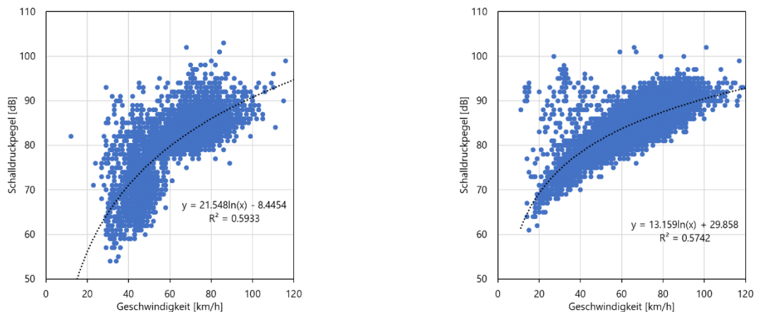
Abbildung 28: X-Y Darstellung der Geschwindigkeits/Schalldruckpegel-Paare am Messpunkt 1 für die Motorräder (links) und PW (rechts).
