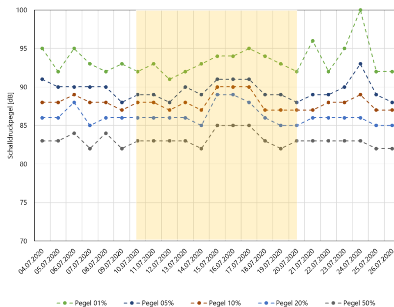
Abbildung 8: Tageweise ausgewertete Schalldruckpegelperzentilwerte für die Motorrad-Ereignisse am Messpunkt 1. Gelb unterlegt ist die Periode mit eingeschaltetem Display. Lesebeispiel: die leisesten 50% der Motorräder erzeugen einen Schalldruckpegel von weniger als 85 dB, die 1% lautesten erzeugen mehr als 92 dB.
