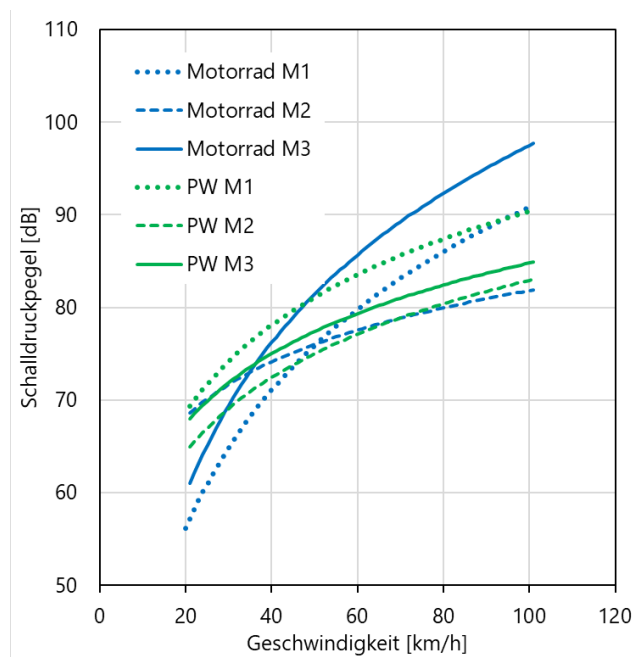
Abbildung 31: Zusammenstellung der Motorrad- und PW-Geschwindigkeitsmodelle an allen drei Messpunkten M1 bis M3.
