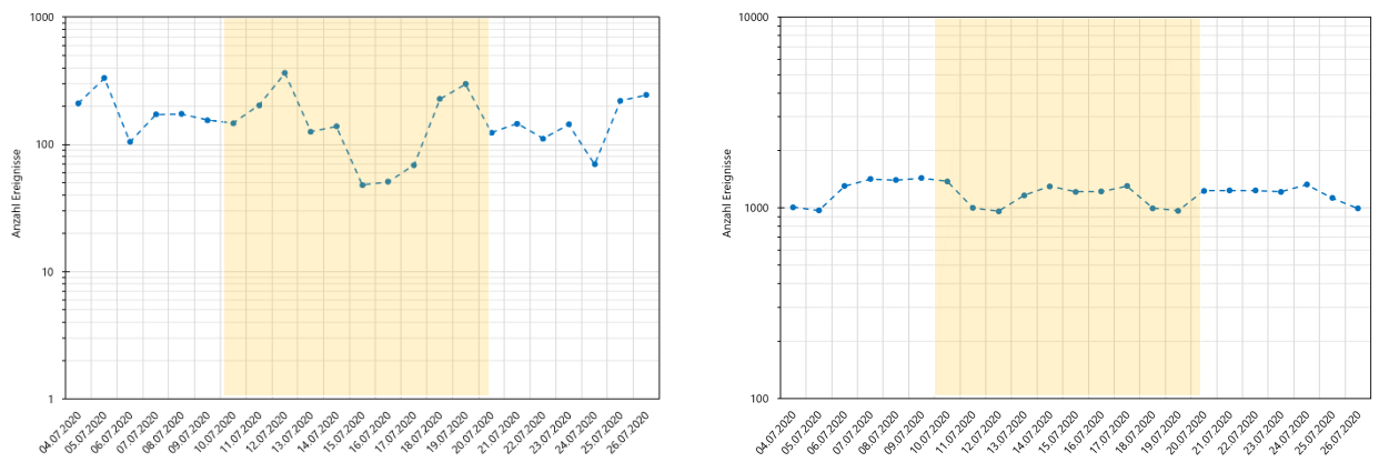
Abbildung 5: Erfasste Tages-Fahrzeugmengen am Messpunkt 2 (links: Motorräder, rechts: Personenwagen).
