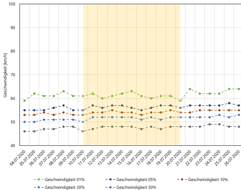
Abbildung 15: Tageweise ausgewertete Geschwindigkeitsperzentilwerte für die PW-Ereignisse am Messpunkt 2. Gelb unterlegt ist die Periode mit eingeschaltetem Display.
