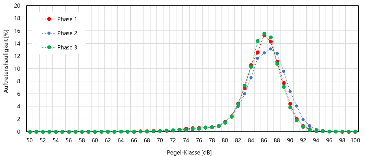
Abbildung 20: Phasenaufgeschlüsselte Pegelverteilung der PW-Ereignisse am Messpunkt 1.
