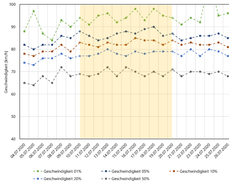
Abbildung 7: Tageweise ausgewertete Geschwindigkeitsperzentilwerte für die Motorrad-Ereignisse am Messpunkt 1. Gelb unterlegt ist die Periode mit eingeschaltetem Display. Lesebeispiel: die langsamsten 50% der Motorräder fahren mit höchstens 70 km/h, die 1% schnellsten sind mit mehr als 90 km/h unterwegs.
