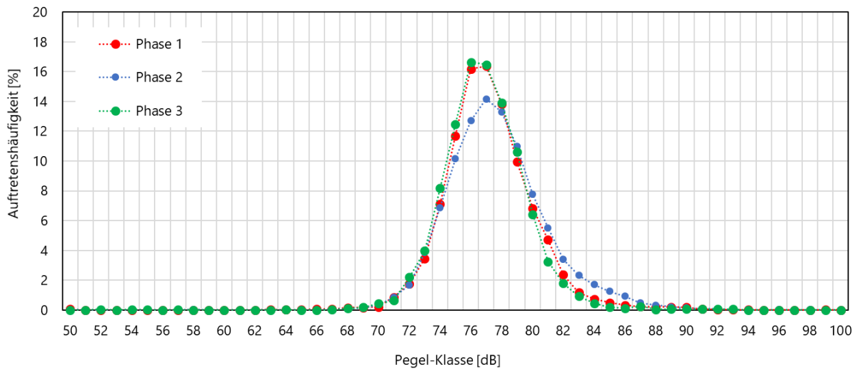
Abbildung 24: Phasenaufgeschlüsselte Pegelverteilung der PW-Ereignisse am Messpunkt 3.
