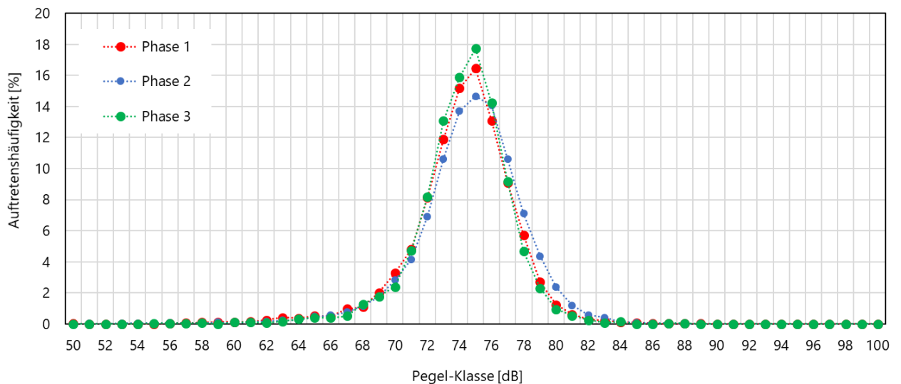
Abbildung 22: Phasenaufgeschlüsselte Pegelverteilung der PW-Ereignisse am Messpunkt 2.
