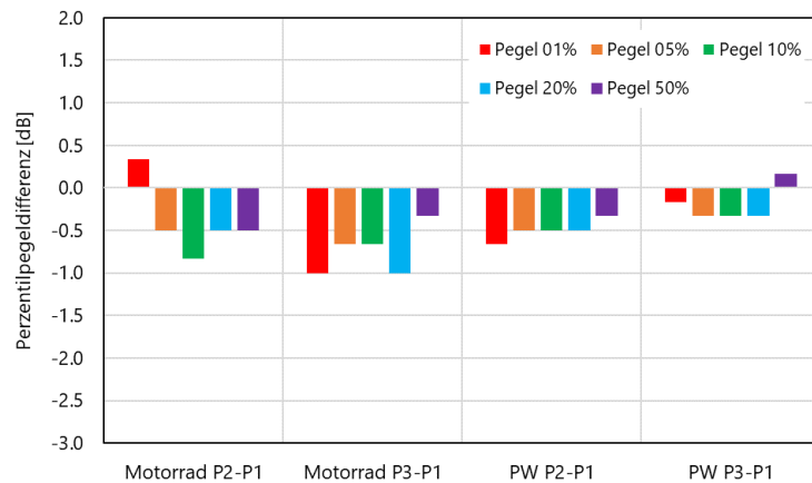
Abbildung 26: Perzentilpegeldifferenzen (1, 5, 10, 20, 50%) am Messpunkt 2 für die beiden Kategorien Motorräder und PW. P2-P1 steht für Phase 2 minus Phase 1, P3-P1 ist Phase 3 minus Phase1.
