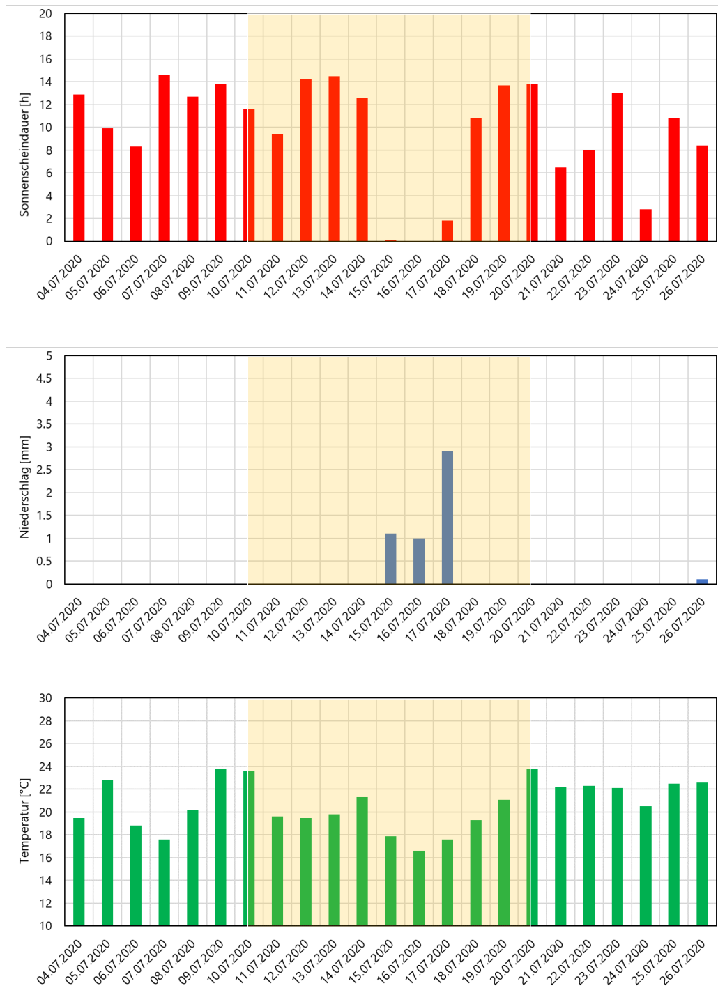
Abbildung 3: Auf jeweils 24 h bezogene Sonnenscheindauer (oben), Niederschlagsmenge (mitte) und Lufttemperatur (unten) gemäss Daten von MeteoSchweiz für die Station Basel-Binningen. Gelb unterlegt ist die Periode mit eingeschaltetem Display.
