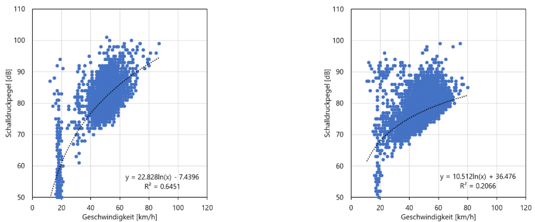
Abbildung 30: X-Y Darstellung der Geschwindigkeits-Schalldruckpegel-Paare am Messpunkt 3 für die Motorräder (links) und PW (rechts).
