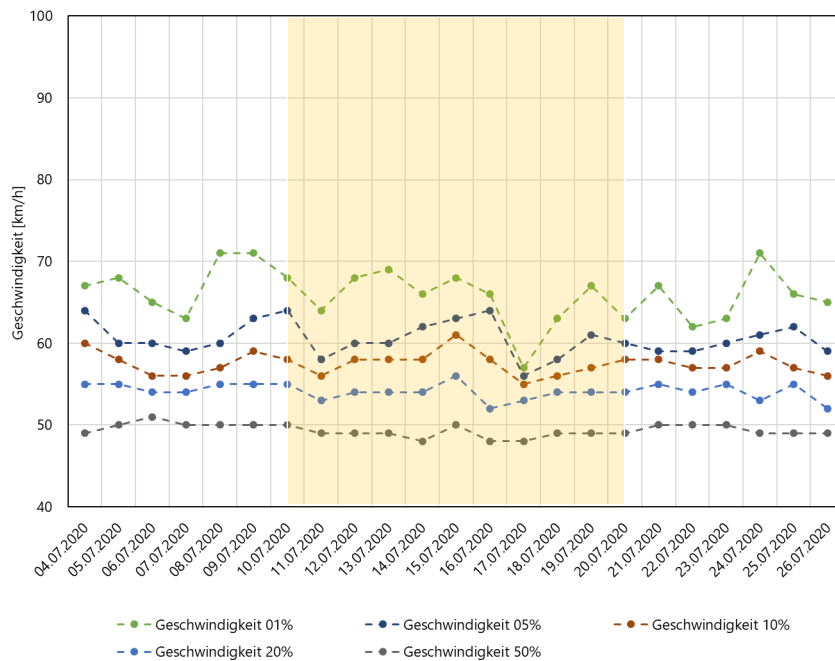
Abbildung 11: Tageweise ausgewertete Geschwindigkeitsperzentilwerte für die Motorrad-Ereignisse am Messpunkt 3. Gelb unterlegt ist die Periode mit eingeschaltetem Display.
