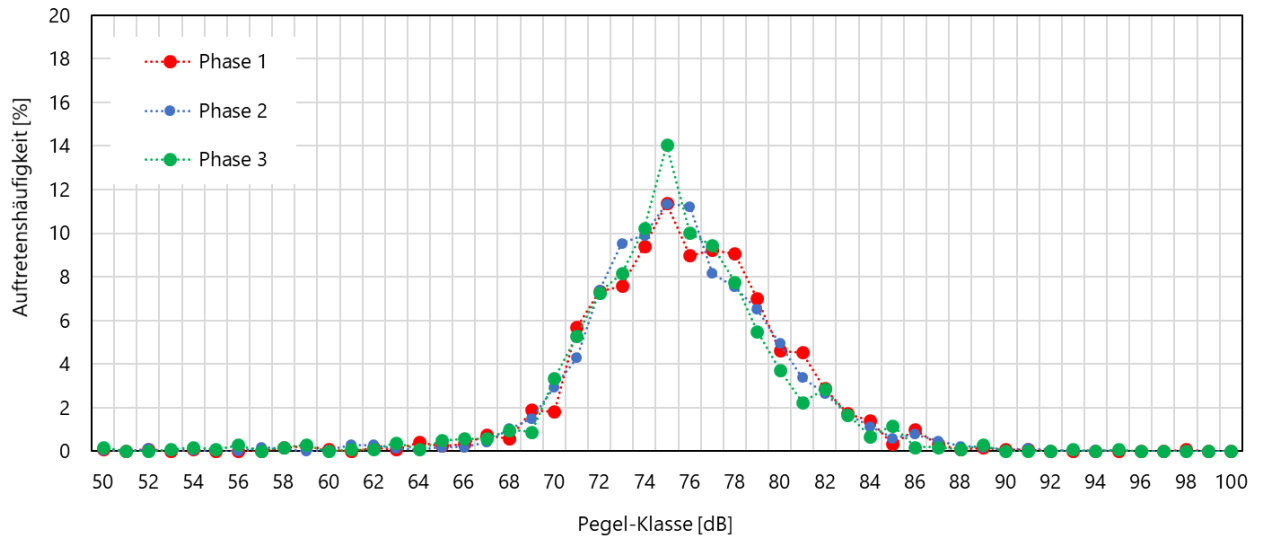
Abbildung 21: Phasenaufgeschlüsselte Pegelverteilung der Motorradereignisse am Messpunkt 2.
