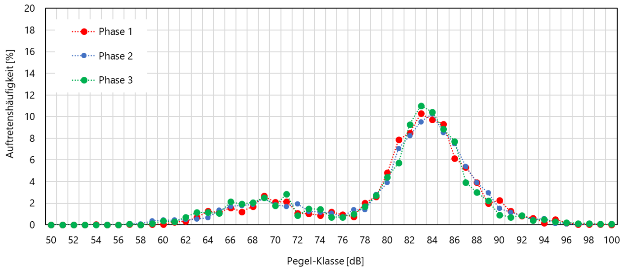
Abbildung 19: Phasenaufgeschlüsselte Pegelverteilung der Motorradereignisse am Messpunkt 1.
