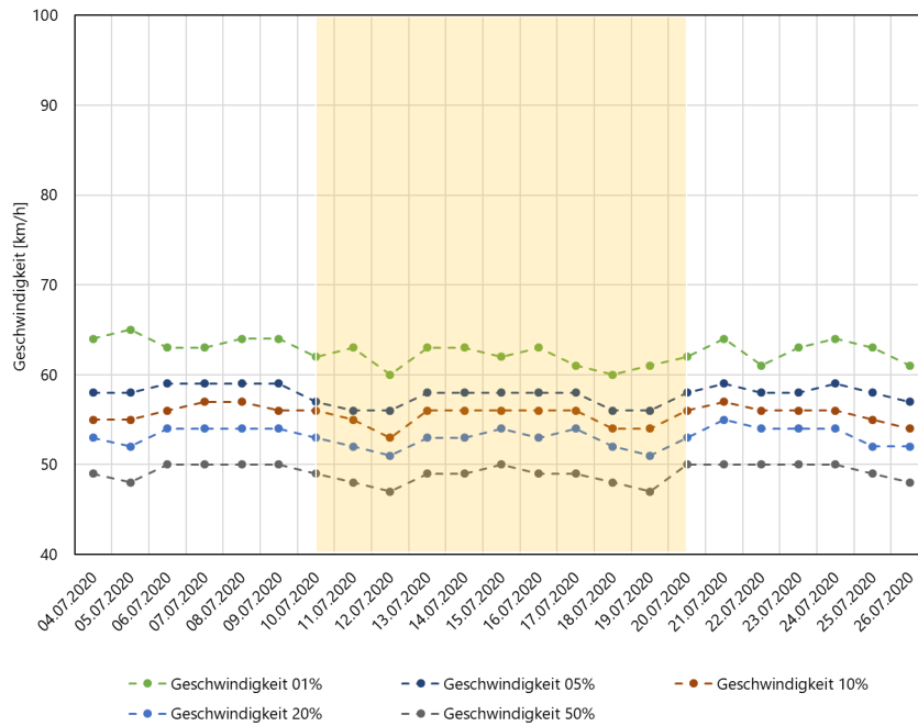
Abbildung 17: Tageweise ausgewertete Geschwindigkeitsperzentilwerte für die PW-Ereignisse am Messpunkt 3. Gelb unterlegt ist die Periode mit eingeschaltetem Display.
