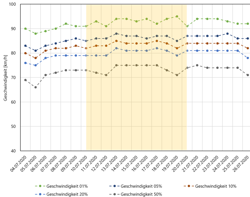
Abbildung 13: Tageweise ausgewertete Geschwindigkeitsperzentilwerte für die PW-Ereignisse am Messpunkt 1. Gelb unterlegt ist die Periode mit eingeschaltetem Display.
