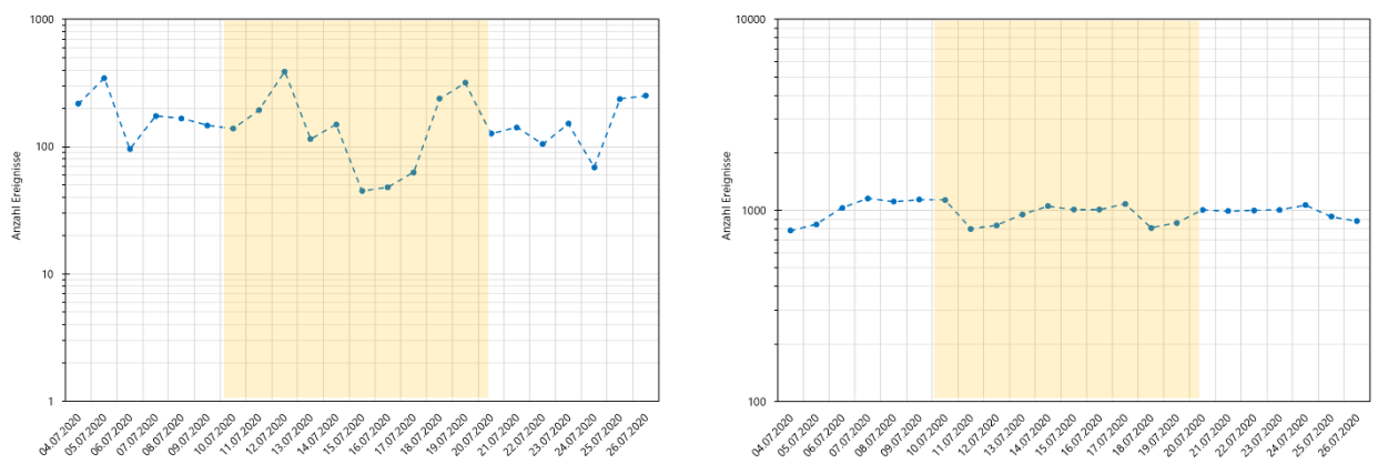
Abbildung 6: Erfasste Tages-Fahrzeugmengen am Messpunkt 3 (links: Motorräder, rechts: Personenwagen).
