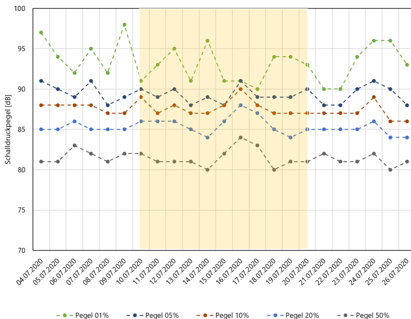
Abbildung 12: Tageweise ausgewertete Schalldruckpegelperzentilwerte für die Motorrad-Ereignisse am Messpunkt 3. Gelb unterlegt ist die Periode mit eingeschaltetem Display.
