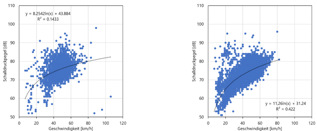
Abbildung 29: X-Y Darstellung der Geschwindigkeits-Schalldruckpegel-Paare am Messpunkt 2 für die Motorräder (links) und PW (rechts).
