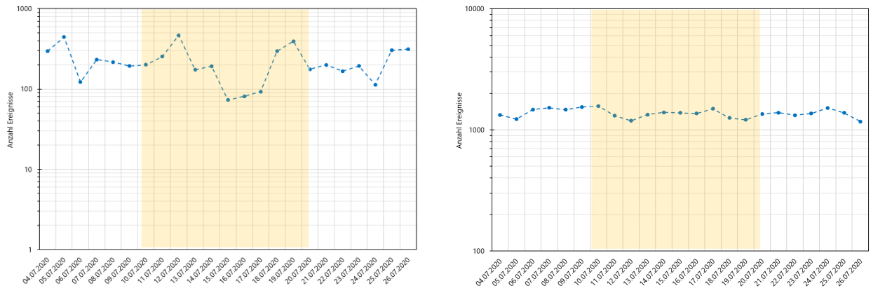
Abbildung 4: Erfasste Tages-Fahrzeugmengen am Messpunkt 1 (links: Motorräder, rechts: Personenwagen).
