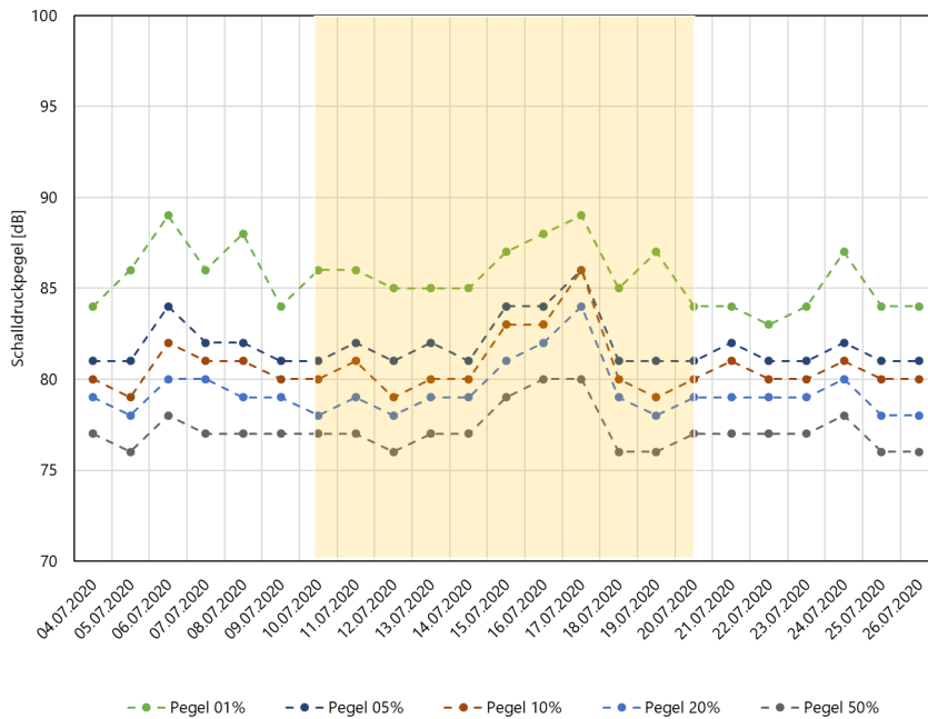
Abbildung 18: Tageweise ausgewertete Schalldruckpegelperzentilwerte für die PW-Ereignisse am Messpunkt 3. Gelb unterlegt ist die Periode mit eingeschaltetem Display.
