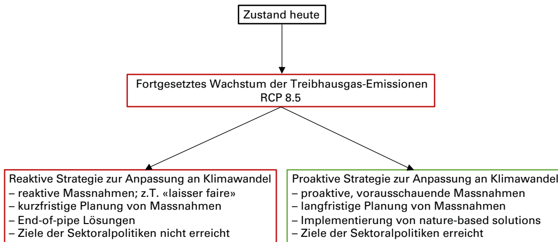
Abb. 2.1: Klimaszenarien, die für die Modellierung bzw. Herleitung der Storylines gewählt wurden.
