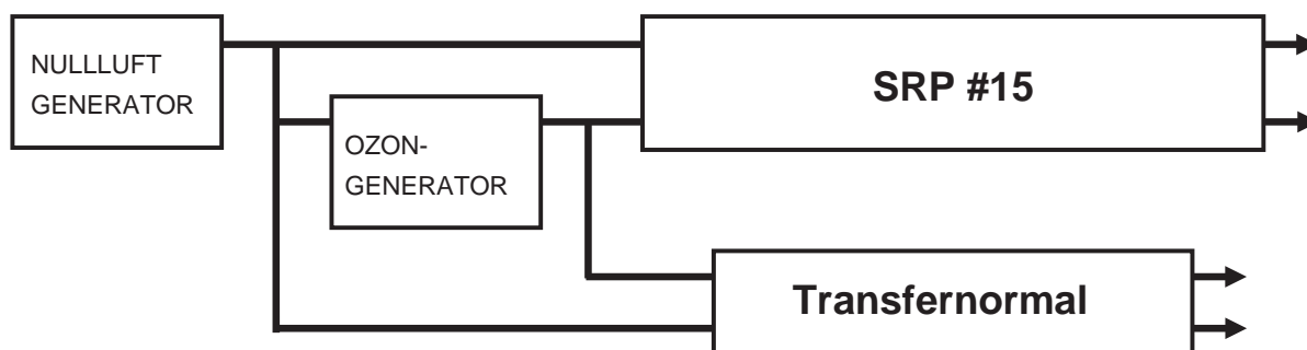
Abb. 4-4: Messanordnung für den Vergleich des Ozon-TransfERNormal mit dem SRP
