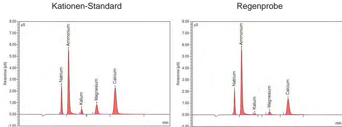
Abb. 3-26: IC-Chromatogramm Kationen-Standard und Regenprobe
