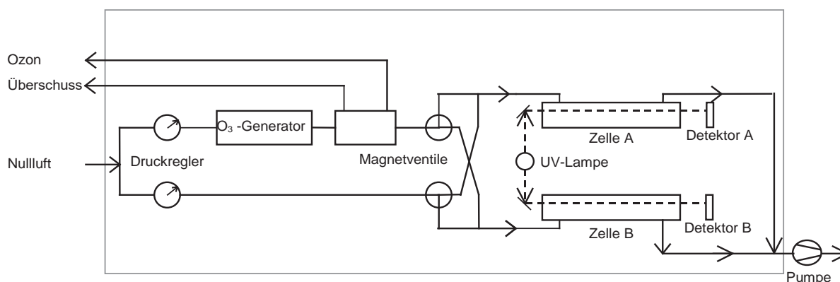
Abb. 4-5: Schematische Darstellung des Thermo 49i-PS
