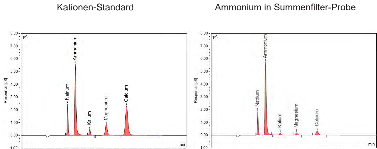
Abb. 3-29: IC- Chromatogramm Kationen - Standard + Summenfilter-Probe
