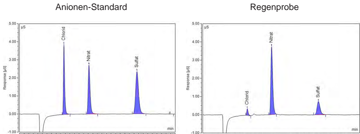
Abb. 3-25: IC-Chromatogramm Anionen-Standard und Regenprobe
