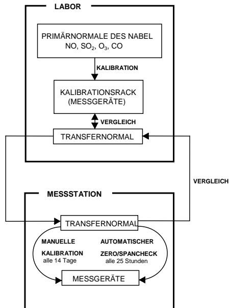
Abb. 4-7: Rückverfolgbarkeit Komponenten CO, NO, O 3 und SO 2
