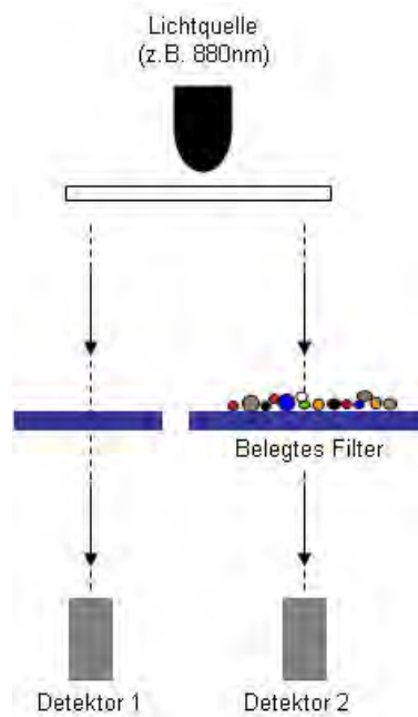
Abb. 3-21: Schematischer Geräteaufbau eines Russmonitor Magese Aethalometer
