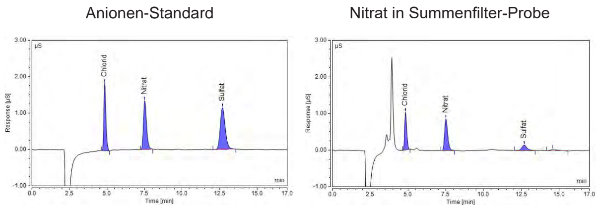
Abb. 3-28: IC Chromatogramm Anionen-Standard und Summenfilter-Probe (Nitrat)
