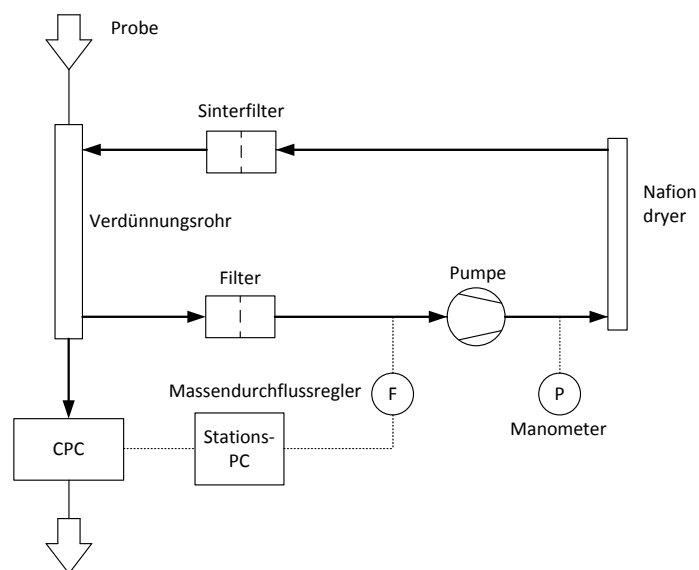
Abb. 3-23: CPC-Verdünnungseinheit
