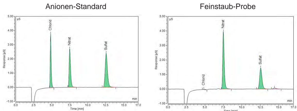
Abb. 3-19: IC-Chromatogramm von Anionen-Standard und Feinstaub-Probe
