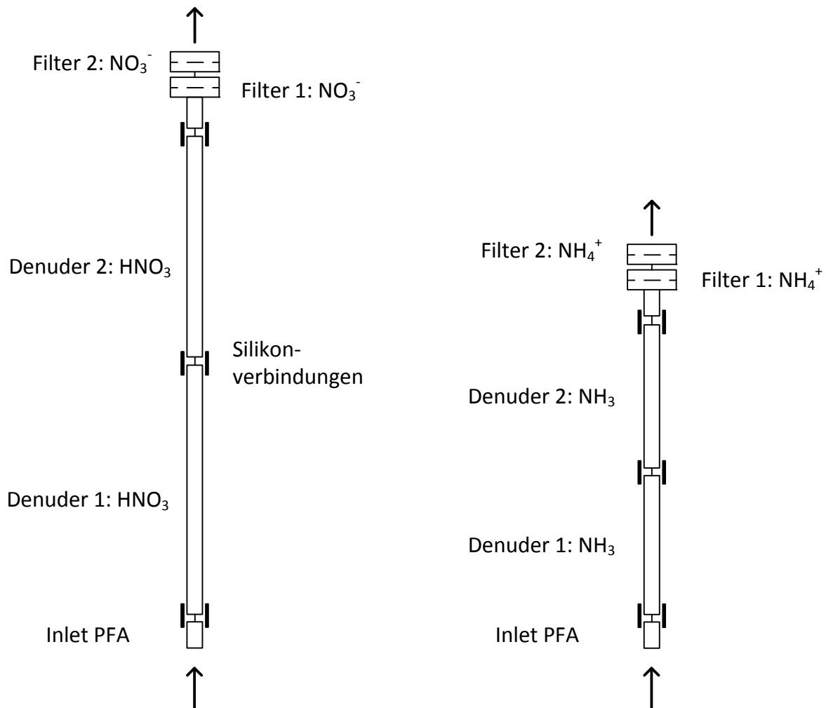
Abb. 3-30: Probetrains zur getrennten Bestimmung von \text{HNO}_3 , \text{NO}_3^- und \text{NH}_3 , \text{NH}_4^+
