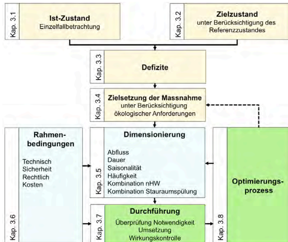
Abb. 3.1: Vorgehen für Planung und Umsetzung von kHW. Durchgezogene Pfeile stellen die Planung eines ersten kHW und den Optimierungsprozess weiterer kHW dar. Die gestrichelte Linie stellt eine im Einzelfall mögliche Anpassung der Zielsetzung durch den Optimierungsprozess dar.
