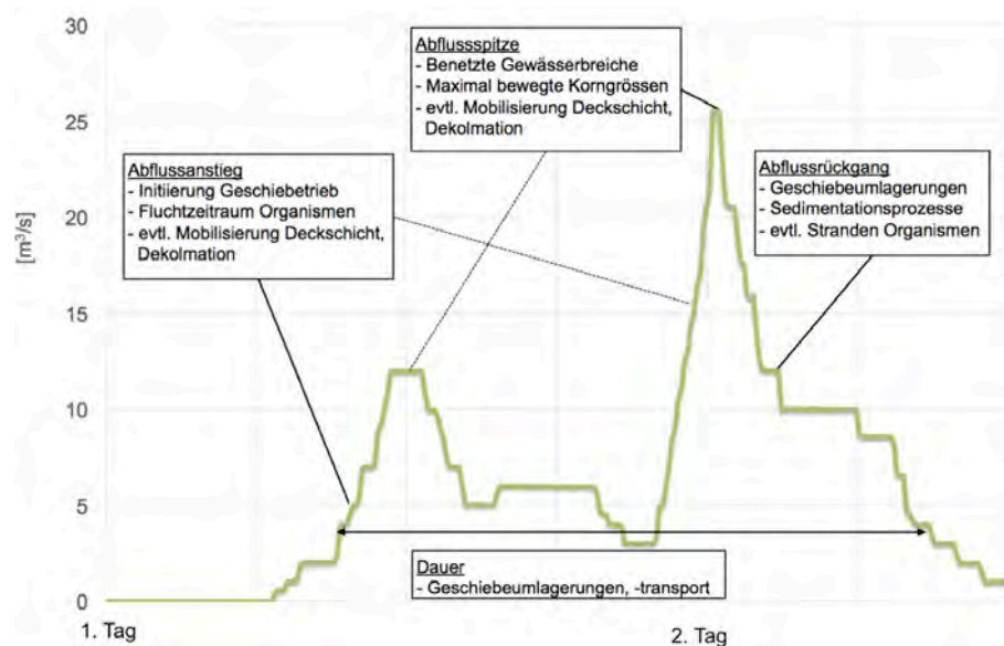
Abb. 3.4: Fiktives Hydrogramm mit möglichen Steuerphasen.
