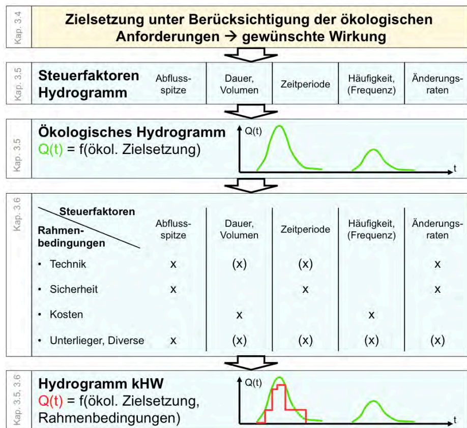
Abb. 3.3: Etappenweises Vorgehen zur Bestimmung des Hydrogramms des kHW. x: Einfluss auf Steuerfaktor; (x): bedingter Einfluss auf Steuerfaktor.
