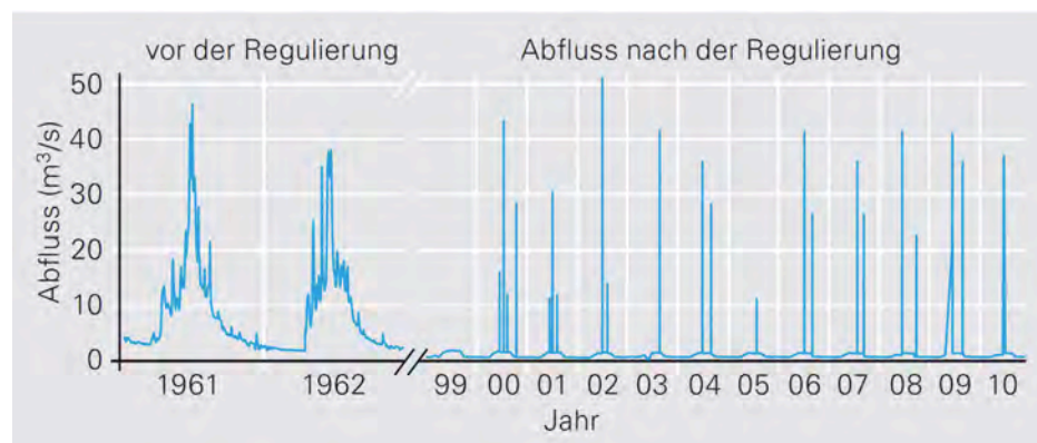
Abb. 3.2: Nachahmung des ursprünglichen Abflussregimes (pre-regulation) am Beispiel Spöl seit 2000 (post-regulation). Quelle: Döring (2012).
