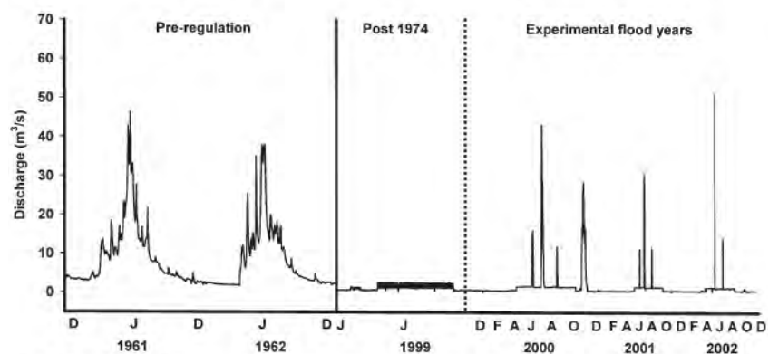
Abb. 2: Abflussverhalten Spöl (Robinson et al., 2013).
