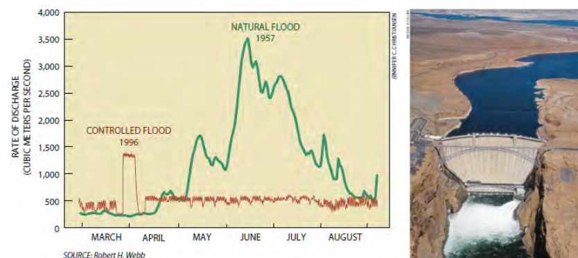
Abb. 3.6: Beispiel Abflussbegrenzung durch Auslassorgane (Collier et al., 1997).
