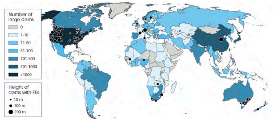
Abb. 2.4: Durchgeführte large-scale flow experiments . FEs = Flow Experiments (Quelle: Olden 2014).
