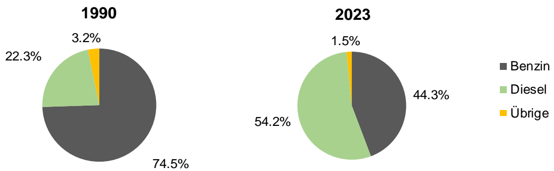
Abbildung 4: Prozentuale Verteilung der CO 2 -Emissionen aus Treibstoffen auf die Energieträger Benzin, Diesel und Übrige (Flugpetrol Inlandflüge und Erdgastreibstoffe) in den Jahren 1990 und 2023.
