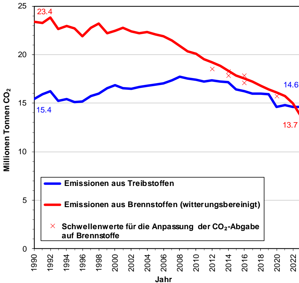
Abbildung 2: Entwicklung der CO 2 -Emissionen aus Brenn- und Treibstoffen (Zeitreihe 1990–2023). Die CO 2 -Emissionen aus Brennstoffen (rot) sind witterungsbereinigt. Die roten Kreuze zeigen die Schwellenwerte, bei deren Überschreitung der Abgabesatz der CO 2 -Abgabe auf Brennstoffe automatisch erhöht wurde. Zurzeit sieht die Gesetzgebung keine weitere Erhöhung der CO 2 -Abgabe vor. Auf den Treibstoffen wird keine CO 2 -Abgabe erhoben, jedoch müssen die Treibstoffimporteure die verursachten CO 2 -Emissionen (blau) teilweise kompensieren.
