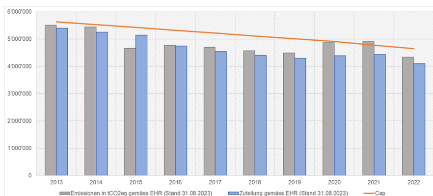
Abbildung 1: Gegenüberstellung der effektiven Emissionen in t CO 2 eq, der kostenlosen Zuteilung an Emissionsrechten und dem Cap
