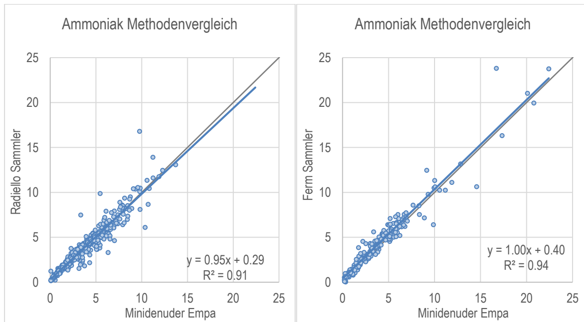
Abb. 54 \text{NH}_3 -Konzentration von Passivsammlern im Vergleich mit Minidenern Oben links: Radiello Sammler und Minidener (Referenzverfahren, Quelle: NABEL), 526 Datenpaare Oben rechts: Ferm Sammler und Minidener (Quelle: NABEL), 309 Datenpaare, Einheit: \mu\text{g m}^{-3}
