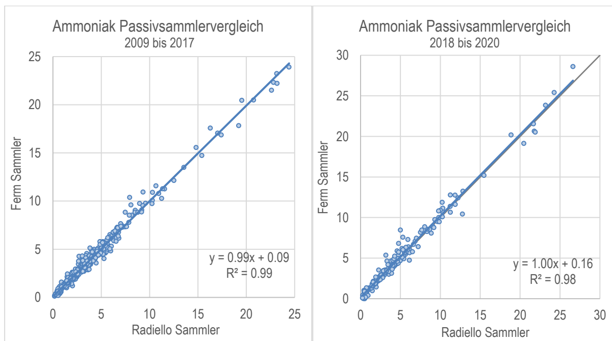
Abb. 55 Radiello- und Ferm-Passivsammler für Ammoniak im Vergleich 2 Passivsammlertypen der FUB: links 2009 bis 2017 (427 Datenpaare), rechts 2018 bis 2020 (205 Datenpaare) Einheit: \mu\text{g m}^{-3}
