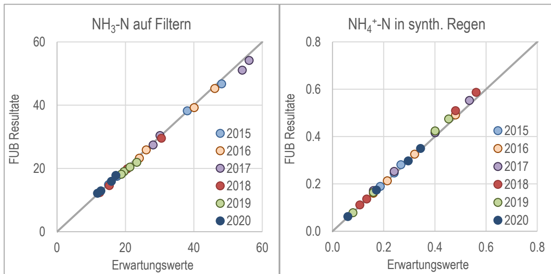
Abb.53 Ringversuchsergebnisse der FUB, verglichen mit den erwarteten Konzentrationen. Links: Ammoniak auf imprägnierten Filtern, Einheit: \mu\text{g N pro Filter} Rechts: Ammonium in Niederschlag, Einheit: \mu\text{g N l}^{-1}
