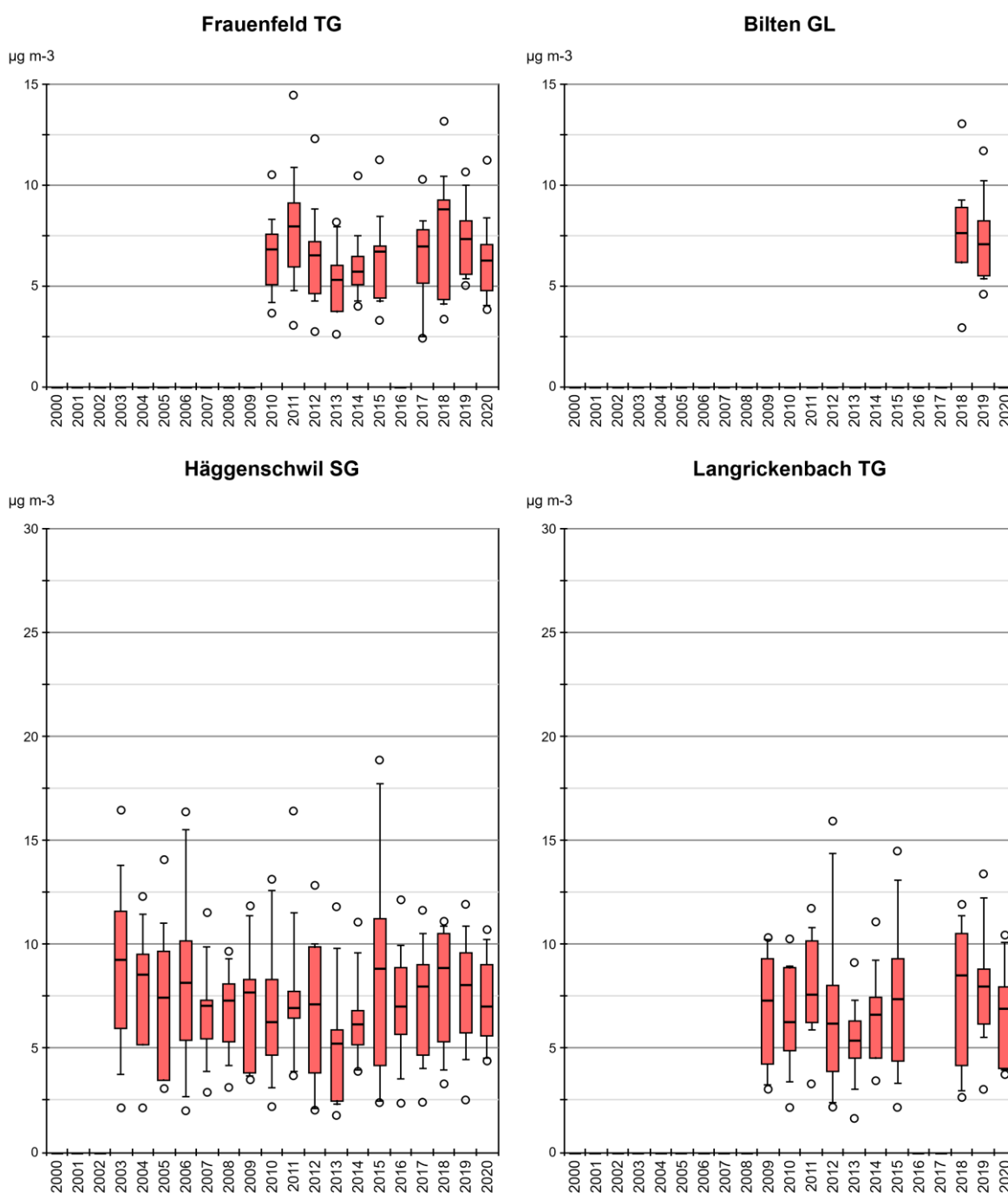
Abb. 30 Ammoniakkonzentration von FRFE, NRB, HÄG, LANG Monatsmittelwerte von Frauenfeld (TG), Biltlen (GL), Häggenschwil (SG), Langgrickenbach (TG) als Boxplots dargestellt.
