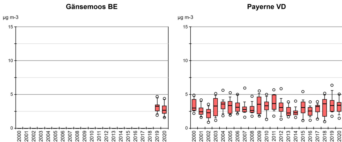
Abb.18 Ammoniakkonzentration von GMO und PAY Monatsmittelwerte von Gänsemoos (BE), Payerne (VD) als Boxplots dargestellt.
