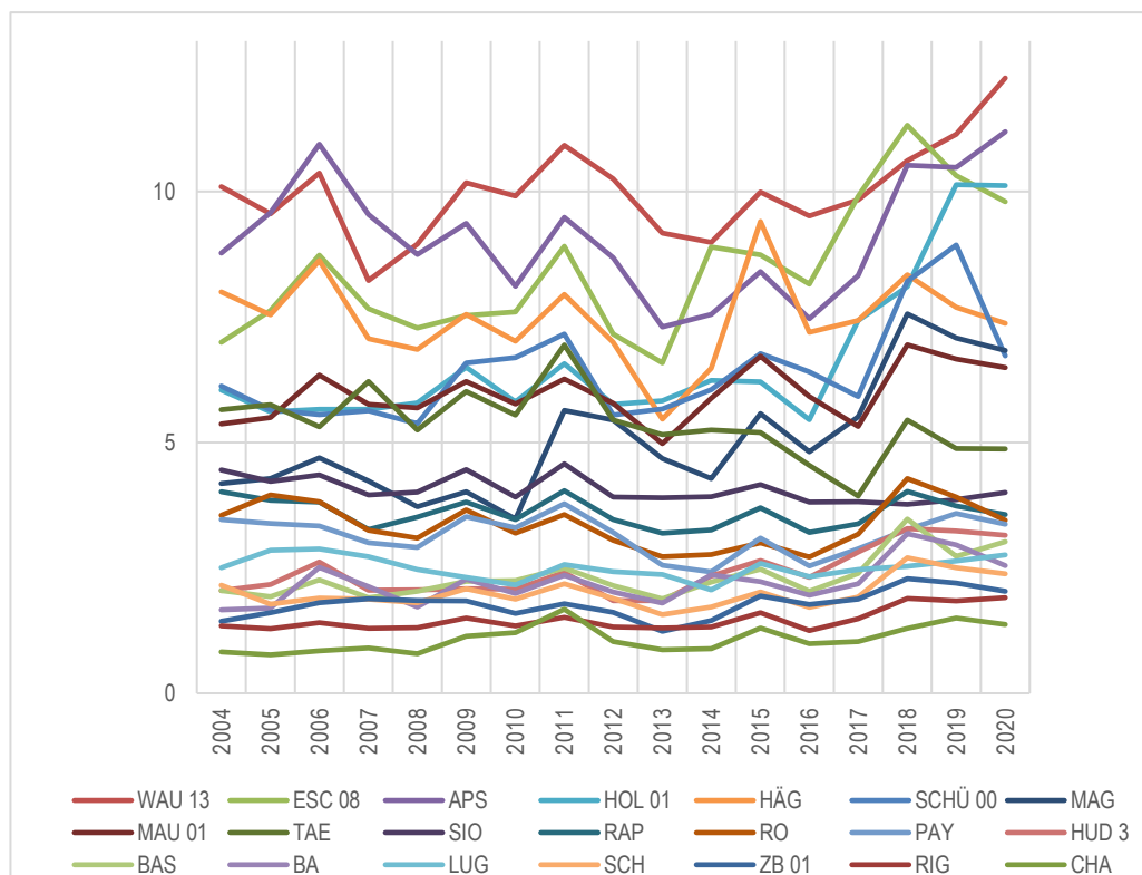
Abb. 5 Standorte mindestens seit 2004, Jahresmittelwerte im Verlauf Jahresmittelwerte der Ammoniakkonzentrationen aller 21 Standorte an denen seit 2004 gemessen wird. Einheit: \mu\text{g m}^{-3}
