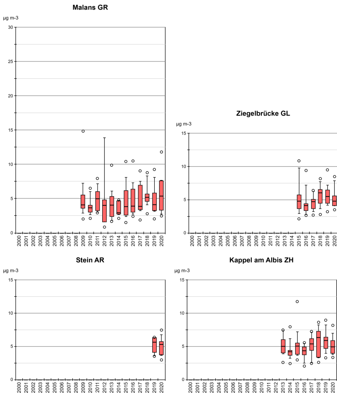
Abb. 24 Ammoniakkonzentration von NMS, BSZ, SSH, KAP Monatsmittelwerte von Malans (GR), Ziegelbrücke (GL), Stein (AR), Kappel am Albis (ZH) als Boxplots dargestellt.
