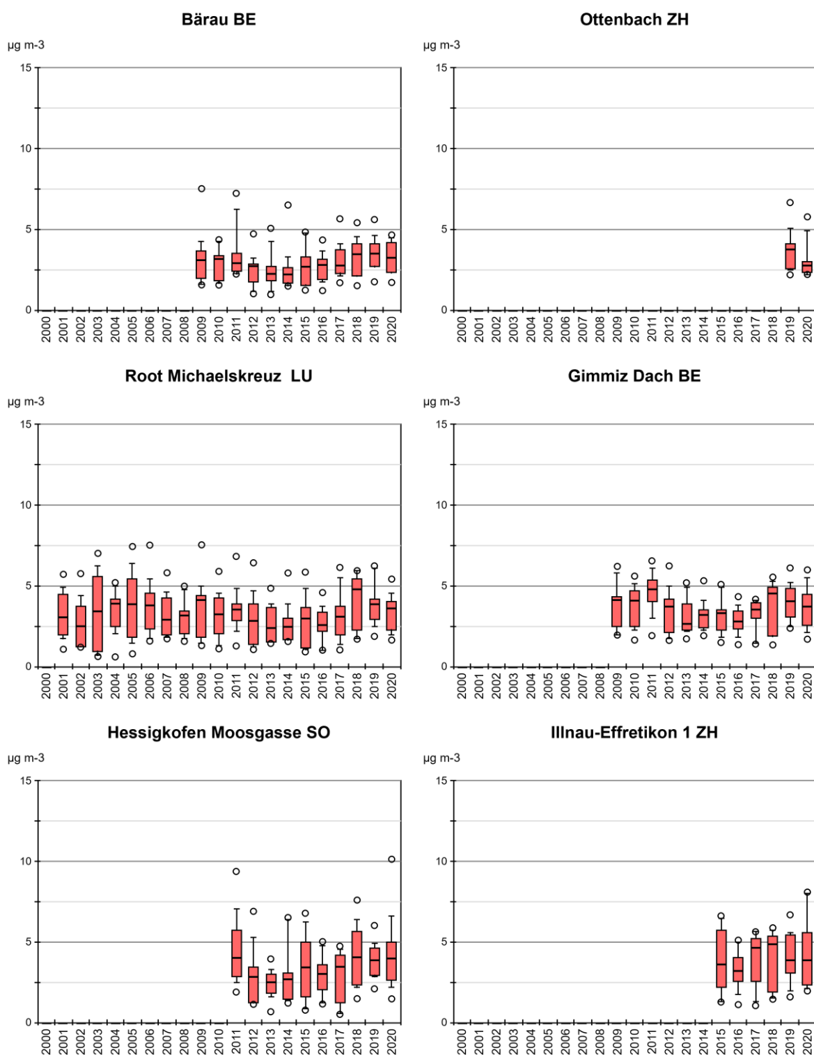
Abb. 19 Ammoniakkonzentration von IEB, OBI, RO, WTG1, HEMO, ILN 01 Monatsmittelwerte von Bärâu (BE), Ottenbach (ZH), Root Michaelskreuz (LU), Gimmiz Dach (BE), Hessigkofen Moosgasse (SO), Illnau-Effretikon 1 (ZH) als Boxplots dargestellt.
