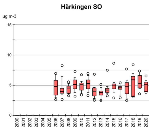
Abb. 37 Ammoniakkonzentration von HAE Monatsmittelwerte von Härkingen (SO) als Boxplots dargestellt.
