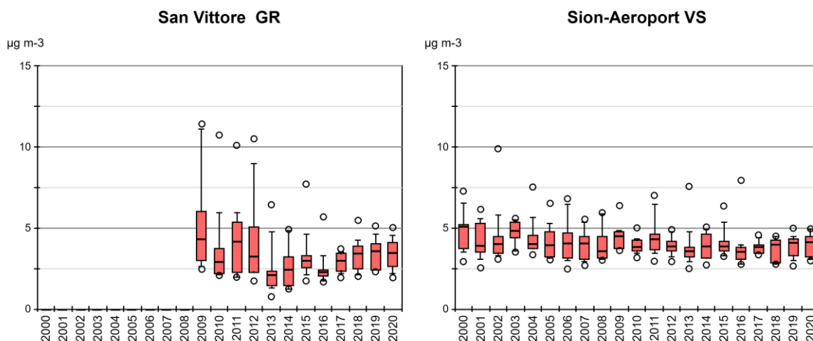
Abb. 36 Ammoniakkonzentration von NV4 und SIO Monatsmittelwerte von San Vittore (GR) und Sion-Aeroport (VS) als Boxplots dargestellt.
