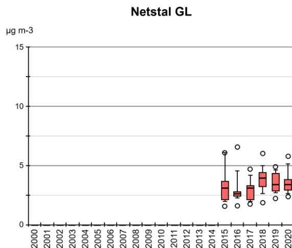
Abb. 34 Ammoniakkonzentration von WIG Monatsmittelwerte von Netstal (GL) als Boxplots dargestellt.
