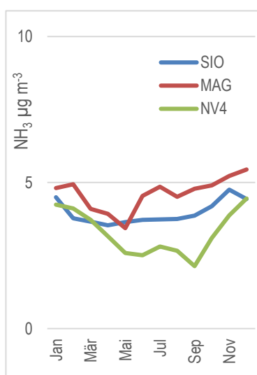
Abb. 45 Jahresgänge der \text{NH}_3 -Konzentration an Standorten mit „untypischem“ Verlauf Mediane der Monatsmittel 2004–2020 (SIO, MAG), 2009–2020 (NV4) Atypischer Jahresgang mit höheren Werten im Winter als im Sommer
