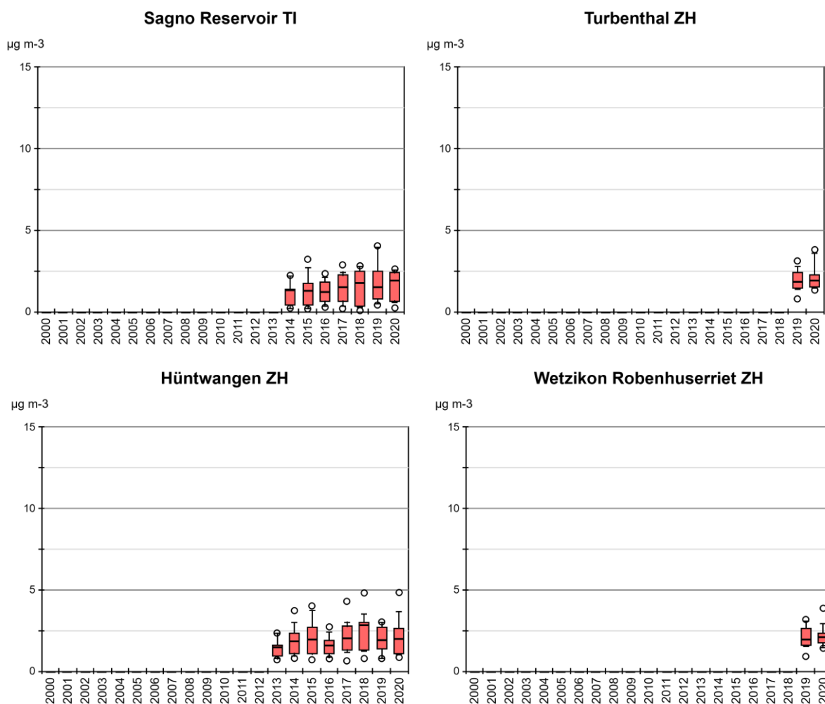
Abb. 15 Ammoniakkonzentration von SARE, TAB, RAF, ROB Monatsmittelwerte von Sagno Reservoir (TI), Turbenthal (ZH), Hüntwangen (ZH), Wetzikon Robenhuserriet (ZH) als Boxplots dargestellt.
