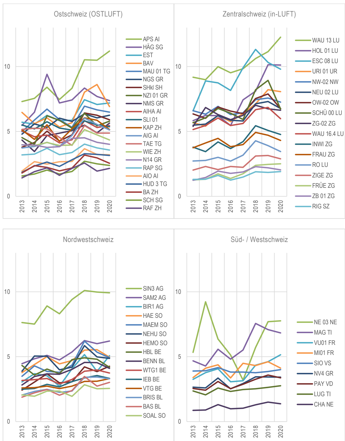
Abb. 8 Standorte seit 2013, Jahresmittelwerte im Verlauf Jahresmittelwerte der Ammoniakkonzentrationen aller 63 Standorte an denen seit 2013 gemessen wird, aufgeteilt nach geografischen Regionen. Einheit: \mu\text{g m}^{-3}
