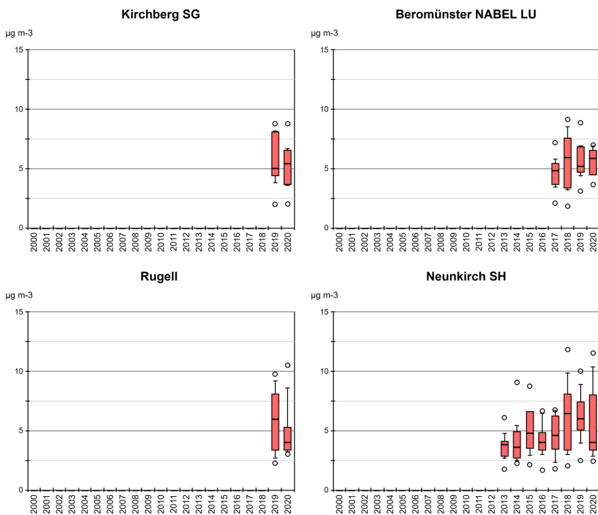
Abb. 25 Ammoniakkonzentration von KIT, BRM, RRI, SHkl Monatsmittelwerte von Kirchberg (SG), Beromünster NABEL (LU), Rugell (FL), Neunkirch (SH) als Boxplots dargestellt.
