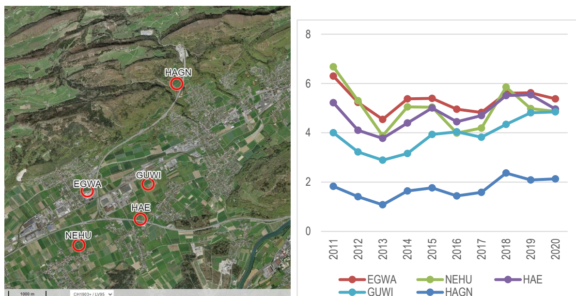
Abb. 49 Luftbild (links) und \text{NH}_3 -Konzentrationen (rechts) der Standorte bei Egerkingen (SO) Verlauf der Jahresmittelwerte, Einheit: \mu\text{g m}^{-3} EGWA liegt direkt zwischen Strasse und Einkaufszentrum; GUWI und NEHU inmitten von Feldern, HAGN am Jurahang in der Nähe des Waldes. Luftbild: geodata © swisstopo
