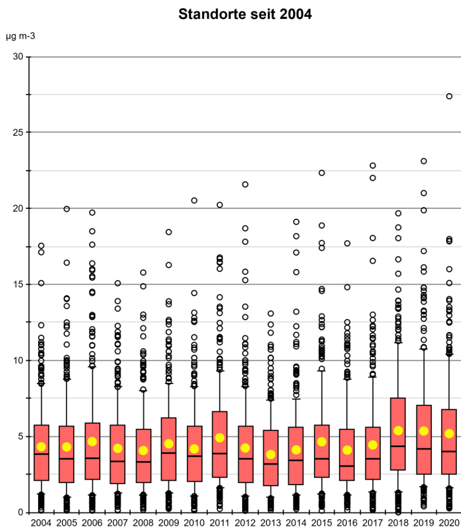
Abb. 4 Monatliche Konzentrationen der Standorte mindestens seit 2004, Boxplots Die Ammoniak-Konzentrationen der 21 Standorte, an denen während 17 Jahren gemessen wurde. Datengrundlage sind Monatsmittelwerte.
