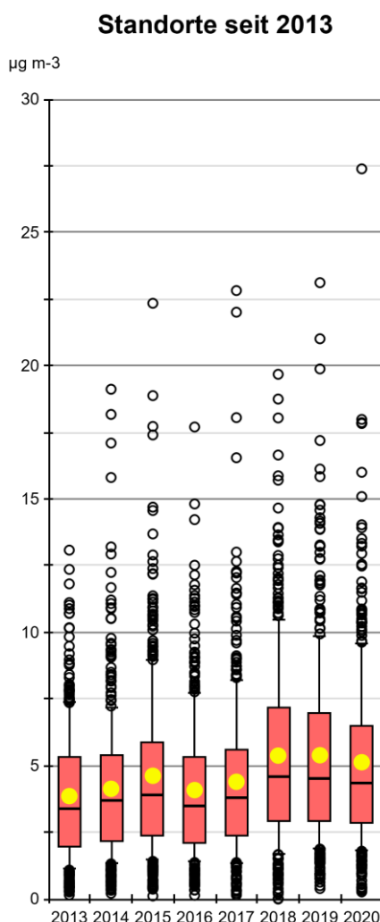
Abb. 9 Standorte mindestens seit 2013, monatliche Konzentrationen als Boxplots Die Ammoniak-Konzentrationen der 63 Standorte, bei denen während 8 Jahren gemessen wurde. Die jährlichen Boxplots fassen die Monatsmittelwerte zusammen. 3
