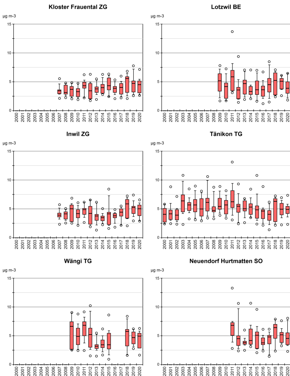
Abb. 21 Ammoniakkonzentration von FRAU, HBL, INWI, TAE, WAEN, NEHU Monatsmittelwerte von Kloster Frauental (ZG), Lotzwil (BE), Inwil (ZG), Tänikon (TG), Wängi (TG), Neuendorf Hurtmatten (SO) als Boxplots dargestellt.
