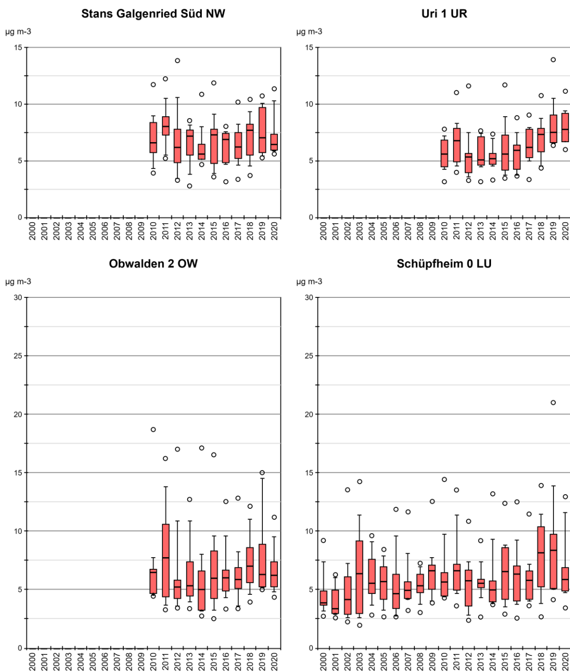
Abb. 29 Ammoniakkonzentration von NW-02, OW-02, URI 01, SCHÜ 00 Monatsmittelwerte von Stans Galgenried Süd (NW), Obwalden 2 (OW), Uri 1 (UR), Schüpheim 0 (LU) als Boxplots dargestellt.
