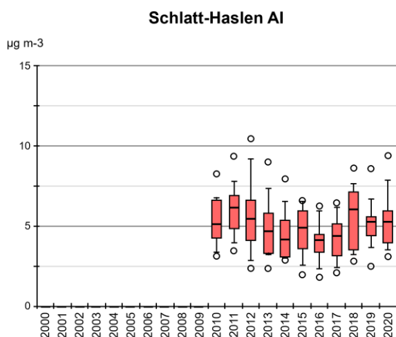
Abb. 23 Ammoniakkonzentration von AIHA, AIG Monatsmittelwerte von Schlatt-Haslen und Gonten (AI), als Boxplots dargestellt.
