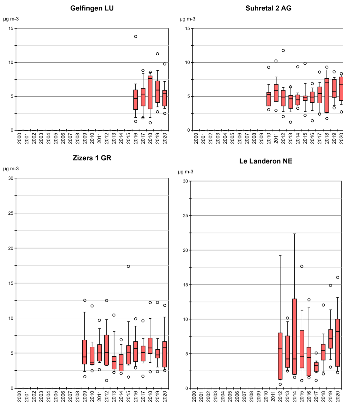
Abb. 26 Ammoniakkonzentration von GEF, SAM2, NZI 01, NE 03 Monatsmittelwerte von Gelfingen (LU), Suhretal 2 (AG), Zizers 1 (GR), Le Landeron (NE) als Boxplots dargestellt.
