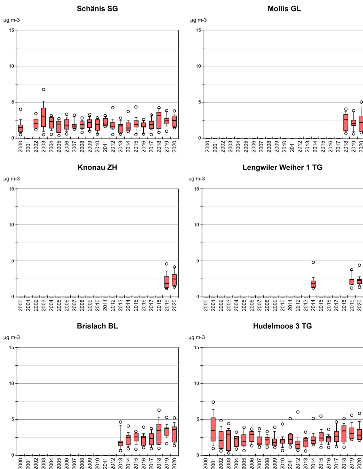
Abb. 16 Ammoniakkonzentration von SCH, WBM, AEG, LEN 1, BRIS, HUD 3 Monatsmittelwerte von Schänis (SG), Mollis (GL), Knonau (ZH), Lengwiler Weiher 1 (TG), Brislach (BL), Hudelmoos 3 (TG) Is Boxplots dargestellt.
