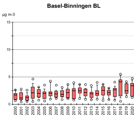
Abb. 38 Ammoniakkonzentration von BAS Monatsmittelwerte von Basel-Binningen (BL) als Boxplots dargestellt.
