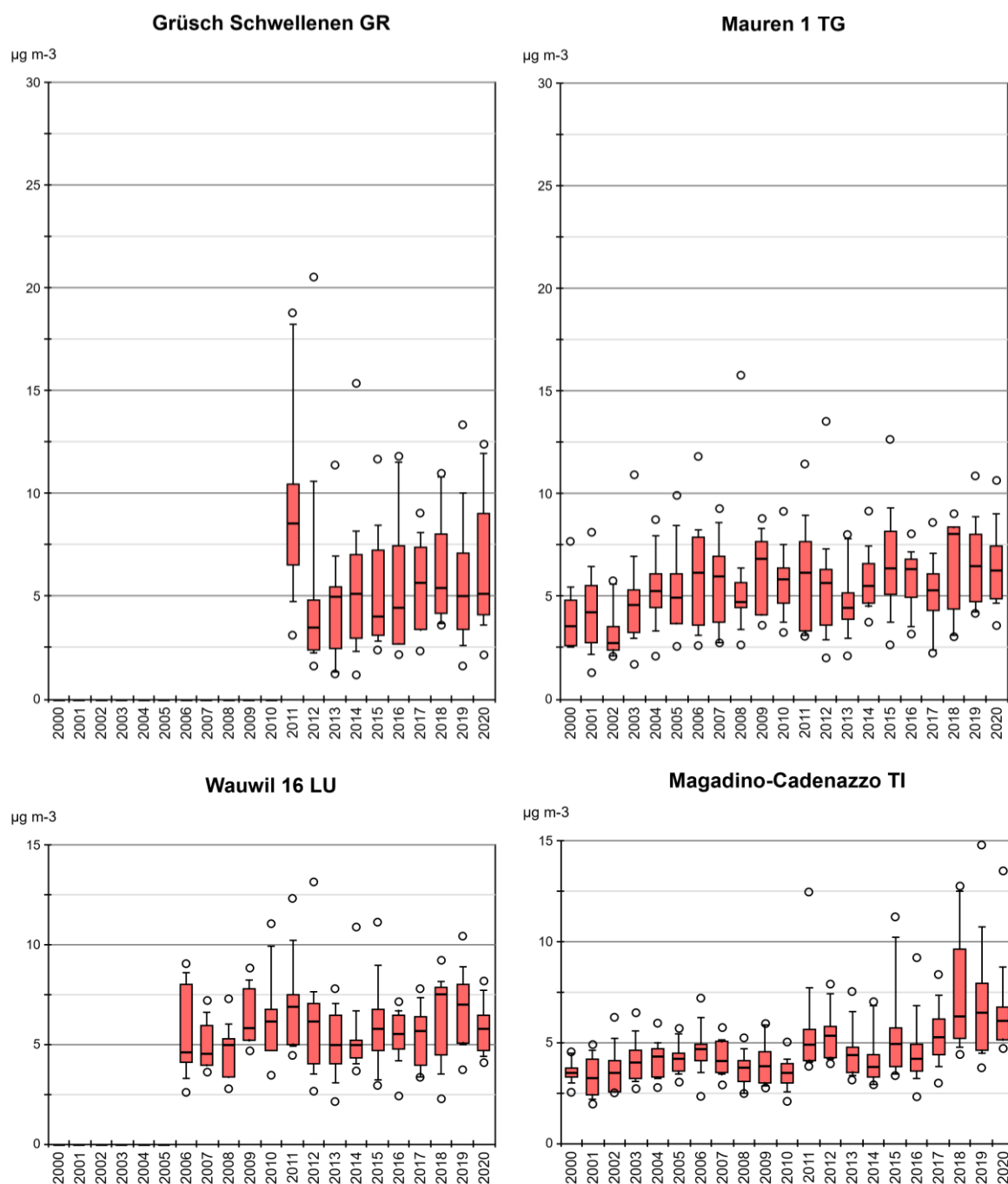
Abb. 27 Ammoniakkonzentration von NGS, WAU 16.4, MAU 01, MAG Monatsmittelwerte von Le Landeron (NE), Grüşch Schwellenen (GR), Wauwil 16 (LU), Mauren 1 (TG), Magadino-Cadenazzo (TI) als Boxplots dargestellt.
