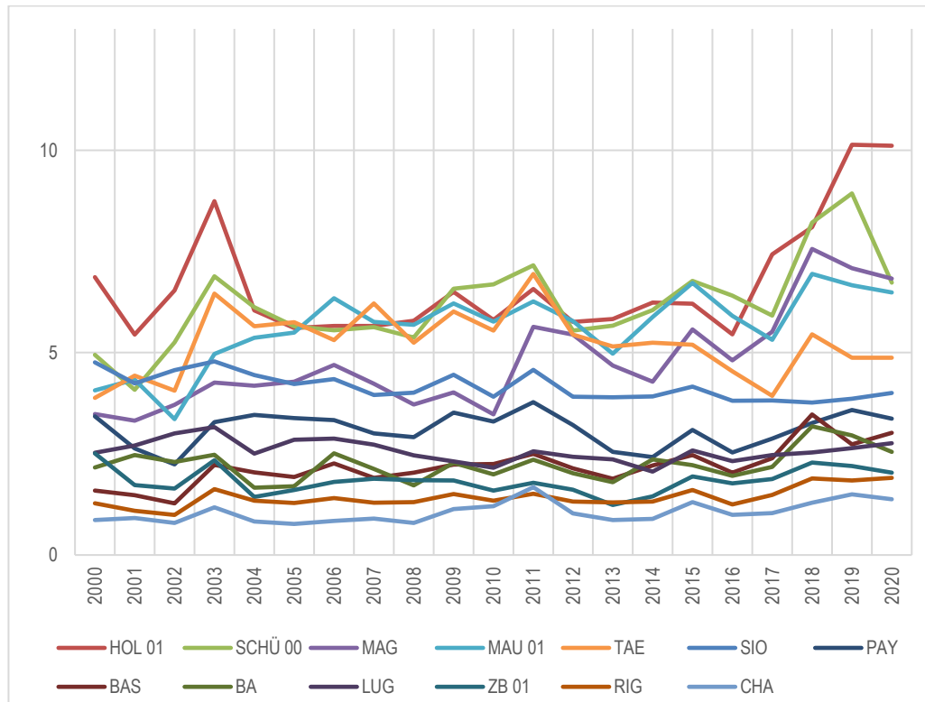
Abb. 3 Standorte seit 2000, Jahresmittelwerte im Verlauf Jahresmittelwerte der Ammoniakkonzentrationen aller 13 Standorte an denen seit 2000 gemessen wird. Einheit: \mu\text{g m}^{-3}
