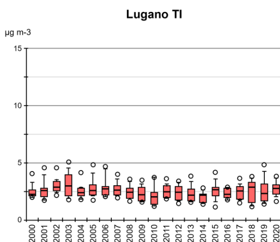
Abb. 39 Ammoniakkonzentration von LUG Monatsmittelwerte von Lugano (TI) als Boxplots dargestellt.
