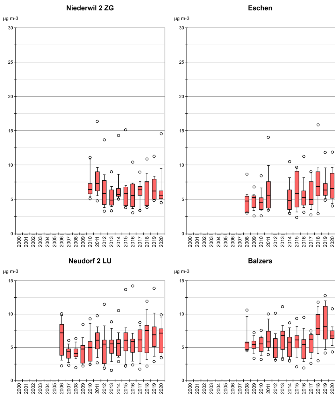
Abb. 28 Ammoniakkonzentration von ZG-02, NEU 02, EST, BAV Monatsmittelwerte von Niederwil 2 (ZG), Neudorf 2 (LU), Eschen und Balzers (FL) als Boxplots dargestellt.
