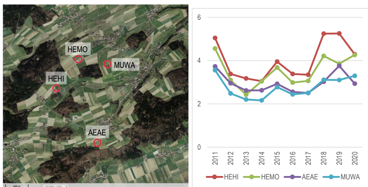
Abb. 47 Luftbild (links) und \text{NH}_3 -Konzentrationen (rechts) der Standorte bei Hessikofen (SO) Verlauf der Jahresmittelwerte, Einheit: \mu\text{g m}^{-3} Alle 4 Standorte befinden sich in Gebieten mit Feld und Ackerwirtschaft. Luftbild: geodata © swisstopo
