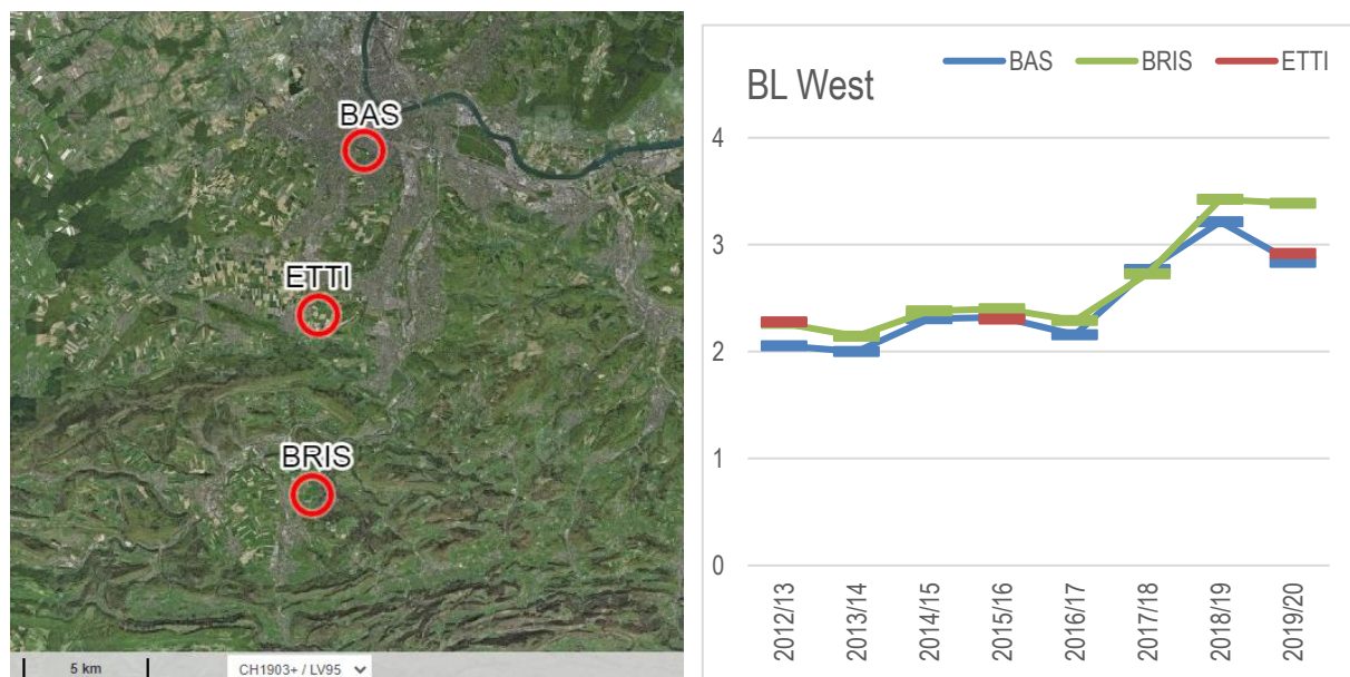
Abb. 52 Luftbild (links) und \text{NH}_3 -Konzentrationen (rechts) der Standorte in Basel Land West Verlauf der Jahresmittelwerte, Einheit: \mu\text{g m}^{-3} . Luftbild: geodata © swisstopo
