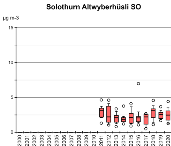
Abb. 40 Ammoniakkonzentration von SOAL Monatsmittelwerte von Solothurn Altwyberhüsli (SO) als Boxplots dargestellt.
