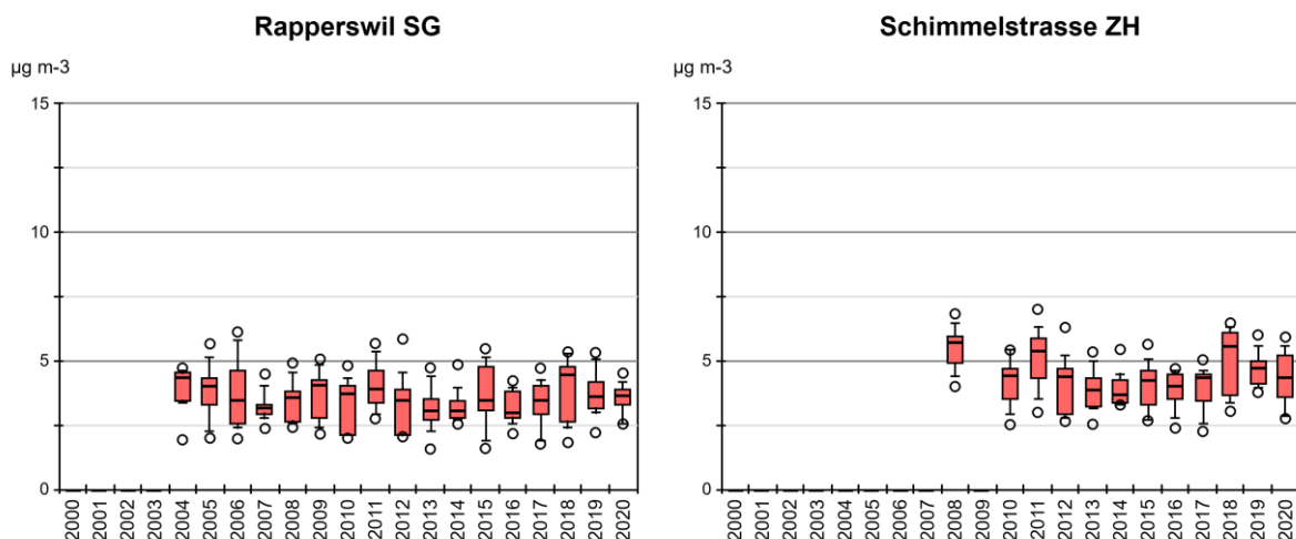
Abb. 41 Ammoniakkonzentration von RAP und WIE Monatsmittelwerte von Rapperswil (SG) und Schimmelstrasse (ZH) als Boxplots dargestellt.
