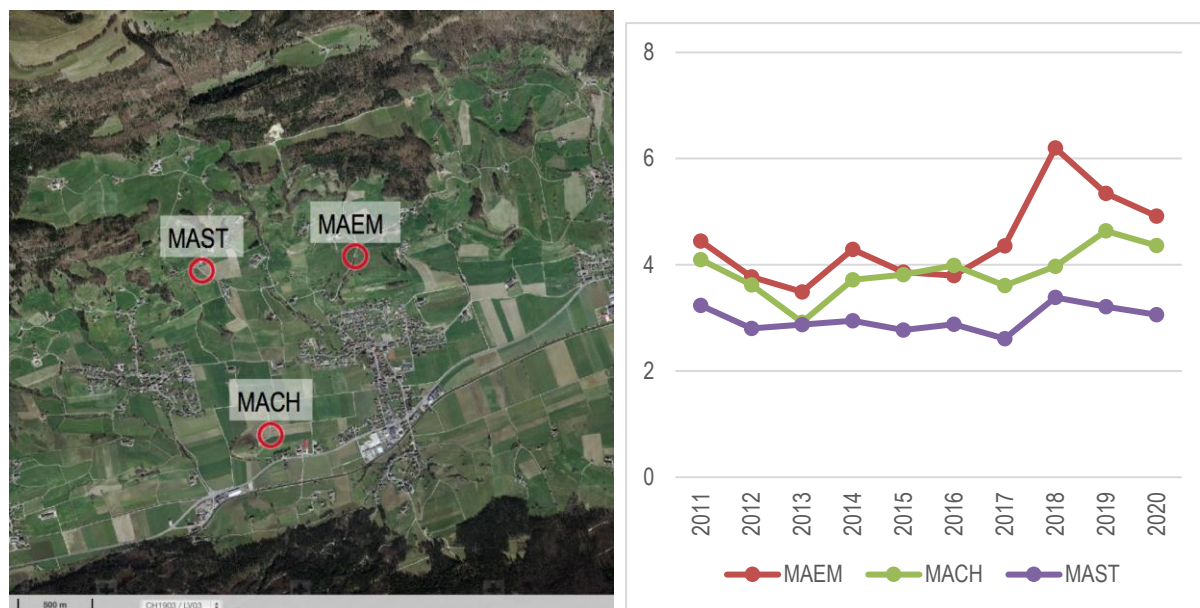
Abb. 48 Luftbild (links) und \text{NH}_3 -Konzentrationen (rechts) der Standorte bei Matzendorf (SO) Verlauf der Jahresmittelwerte, Einheit: \mu\text{g m}^{-3} Alle 3 Standorte befinden sich in Gebieten mit Feld und Ackerwirtschaft. Luftbild: geodata © swisstopo
