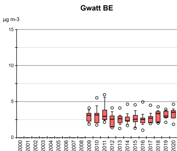
Abb.17 Ammoniakkonzentration von VTG Monatsmittelwerte von Gwatt (BE) als Boxplots dargestellt.
