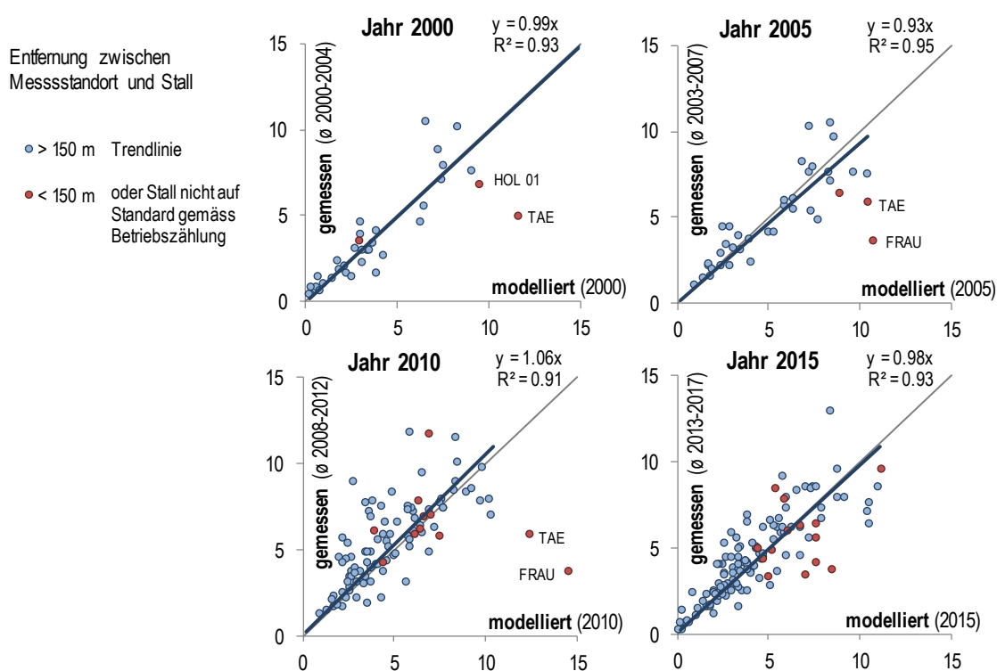
Abb. 11 Vergleich modellierter mit gemessenen \text{NH}_3 -Konzentrationen, Jahre 2000 resp. 2000–2004, 2005 resp. 2003–2007, 2010 resp. 2008–2012 und 2015 resp. 2013–2017 Die Trendlinien beziehen sich nur auf Standorte > 150 m entfernt von landwirtschaftlichen Betrieben (blaue Punkte). Einheit: \mu\text{g m}^{-3}
