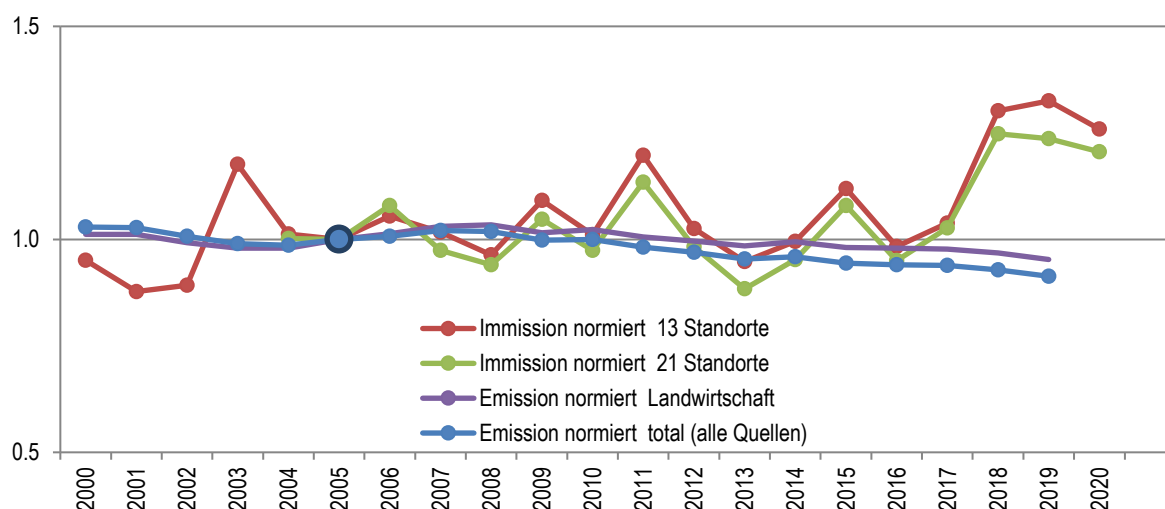
Abb. 10 Vergleich der Entwicklung von Emissionen und Immissionen, alle normiert auf das Jahr 2005. Die Emissionen (Summe aller Quellengruppen sowie Quelle Landwirtschaft) und die Mittelwerte der Immissionen der 13 bzw. 21 Standorte wurden auf das Bezugsjahr 2005 normiert.
