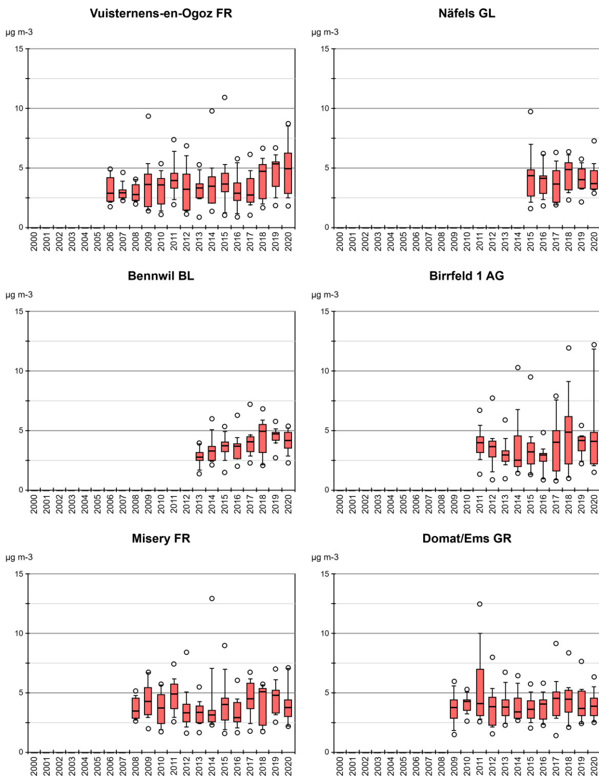
Abb. 20 Ammoniakkonzentration von VU01, DEB, BENN, BIR1, MI01, N14 Monatsmittelwerte von Vuisternens-en-Ogoz (FR), Näfels (GL), Bennwil (BL), Birrfeld 1 (AG), Misery (FR), Domat/Ems (GR) als Boxplots dargestellt.
