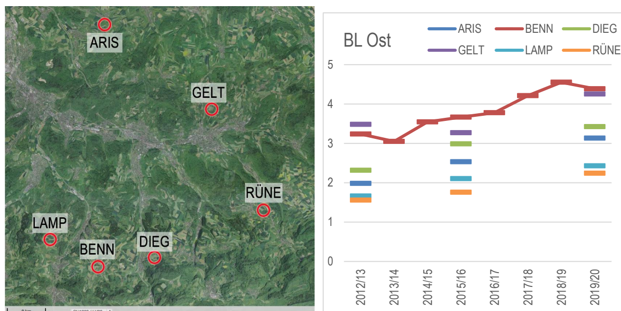
Abb. 51 Luftbild (links) und \text{NH}_3 -Konzentrationen (rechts) der Standorte in Basel Land Ost Verlauf der Jahresmittelwerte, Einheit: \mu\text{g m}^{-3} . Luftbild: geodata © swisstopo
