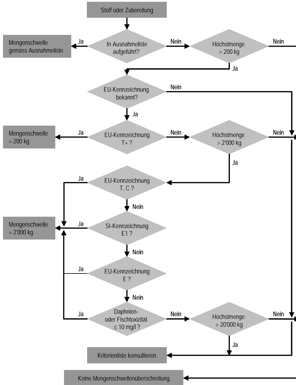
Abb. 3 > Fließschema für Stoffe und Zubereitungen (für Mengenschwellen bis 2000 kg)
