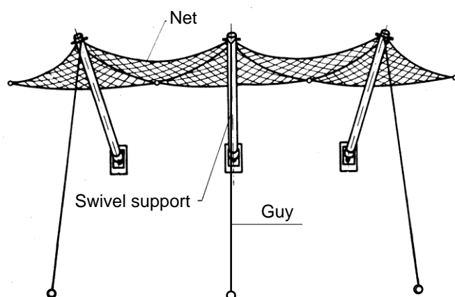
Fig. 3 > Snow net.
