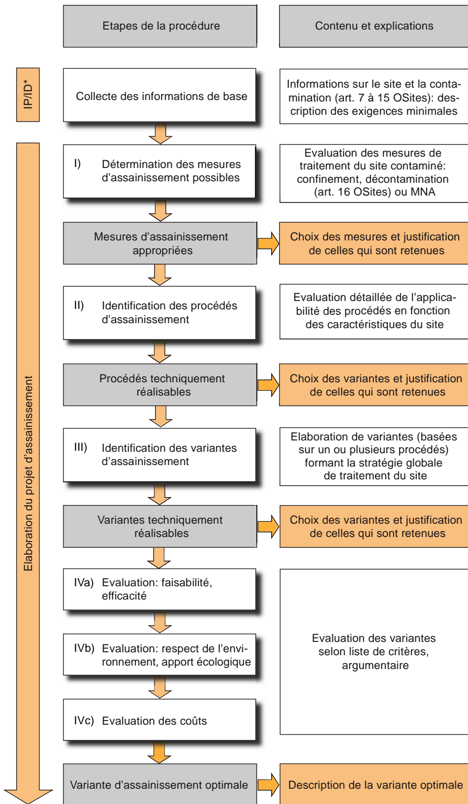
Fig. 2 > Déroulement de la procédure d'identification et d'évaluation des variantes d'assainissement
