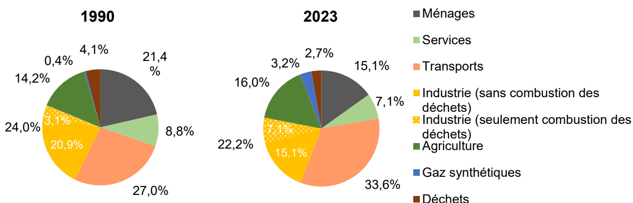
Figure 8 : Émissions de gaz à effet de serre (sans bilan des gaz à effet de serre lié à l'utilisation des terres) de la Suisse selon la loi sur le CO 2 et l'Accord de Paris, par secteur en vertu de l'ordonnance sur le CO 2 , en 1990 et en 2023 (cf. tableau 9 pour le détail de la composition des secteurs).
