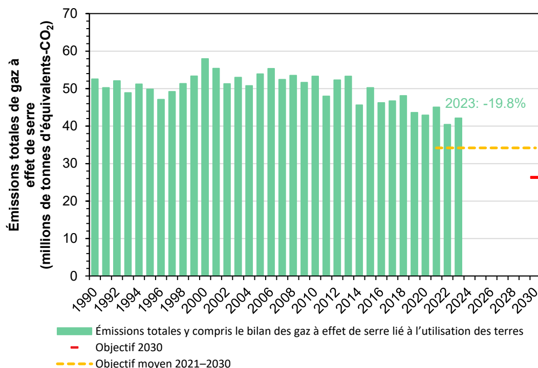
Figure 5 : Évolution des émissions totales de gaz à effet de serre de la Suisse selon la loi sur le CO 2 et l'Accord de Paris (y compris le bilan des gaz à effet de serre lié à l'utilisation des terres). Est également indiquée la réduction en pourcentage par rapport à 1990 pour l'année la plus récente. La ligne rouge indique la valeur cible pour l'année 2030 (d'au moins moins 50 % par rapport aux émissions totales de gaz à effet de serre en 1990). En outre, la Suisse s'est engagée à réduire ses émissions d'au moins 35 % en moyenne entre 2021 et 2030 par rapport à 1990 (ligne orange en pointillés). Les attestations internationales, qui sont également pris en compte pour l'examen des objectifs, ne sont pas représentés ici.
