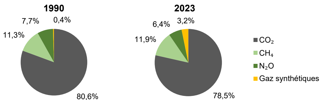
Figure 7 : Émissions de gaz à effet de serre (sans bilan des gaz à effet de serre lié à l'utilisation des terres) de la Suisse selon la loi sur le CO 2 et l'Accord de Paris, par gaz, en 1990 et en 2023.
