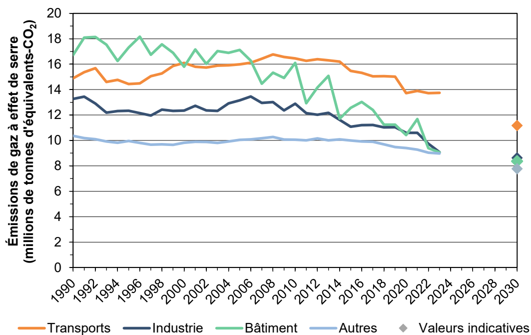
Figure 6 : Évolution des émissions de gaz à effet de serre dans les secteurs visés par l’ordonnance sur le CO 2 . Sont également indiquées les valeurs indicatives pour l’année 2030 (voir chapitre 1.6). Au total, les émissions des secteurs des transports, de l’industrie et du bâtiment, ainsi que les autres sources, ont diminué de 26,1 % entre 1990 et 2023 par rapport à 1990.
