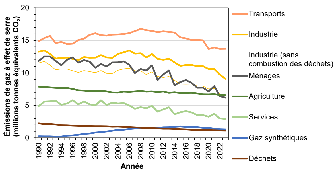
Figure 9 : Évolution des émissions de gaz à effet de serre (sans bilan des gaz à effet de serre lié à l'utilisation des terres) de la Suisse selon la loi sur le CO 2 et l'Accord de Paris, par secteur en vertu de l'ordonnance sur le CO 2 , au cours de la période 1990–2023 (cf. tableau 9 pour le détail de la composition des secteurs).
