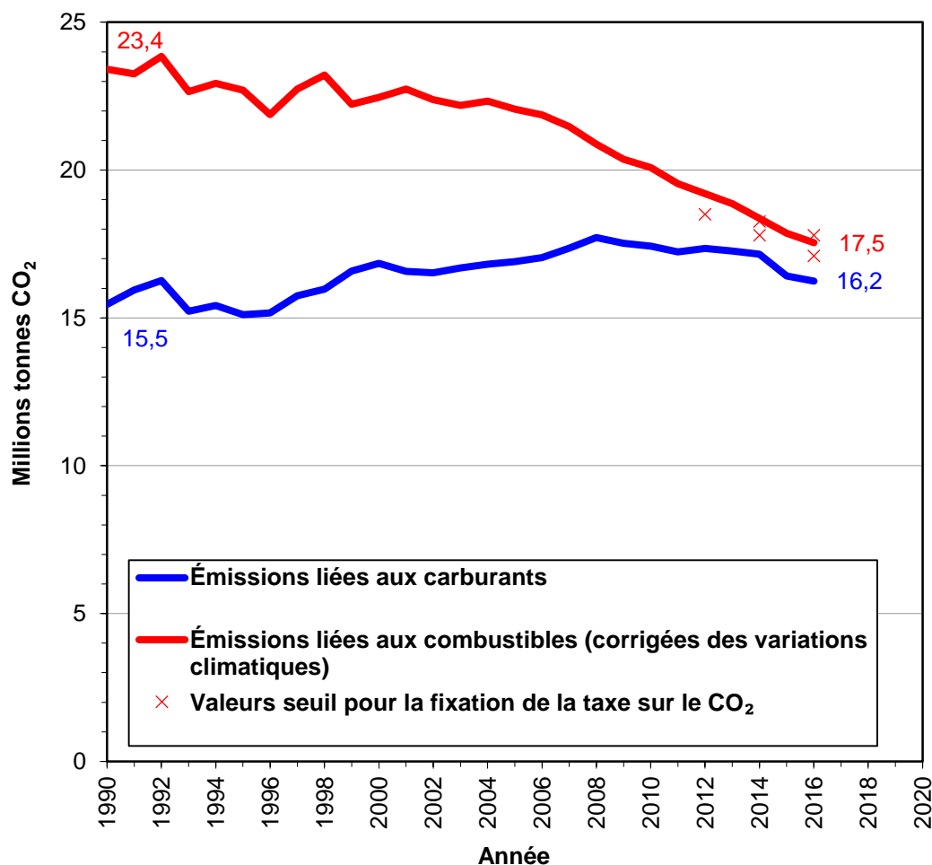
Figure 2 : Série temporelle (1990–2016) des émissions de CO 2 énergétiques, en millions de tonnes de CO 2 . En bleu : émissions effectives de CO 2 liées aux carburants. En rouge : émissions de CO 2 liées aux combustibles prises en compte après correction climatique pour déterminer le montant de la taxe sur le CO 2 . Les croix rouges correspondent aux valeurs seuil déterminantes pour la hausse du montant de cette taxe (cf. tableau 1).
