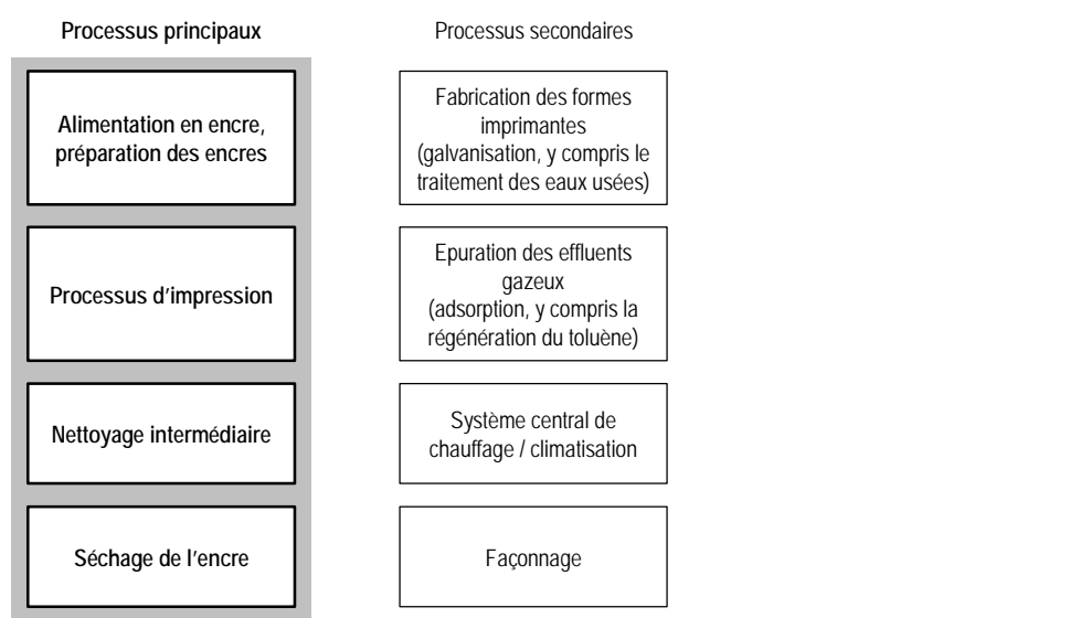
Fig. 1 > Processus principaux et secondaires dans les installations d'héliogravure d'édition
