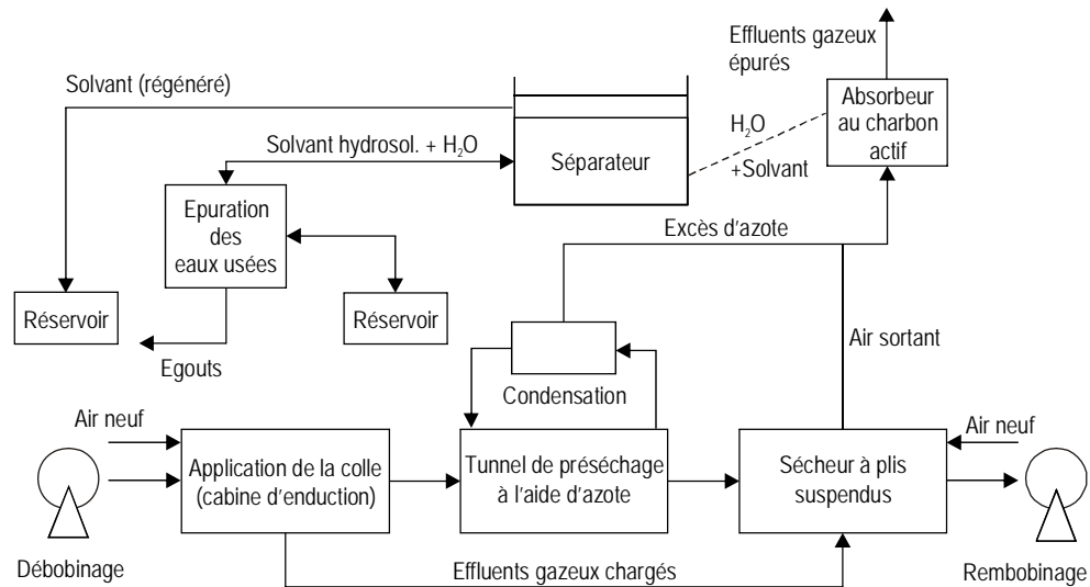
Fig. 4 > Fabrication de rubans adhésifs avec des colles à solvants et épuration des effluents gazeux
