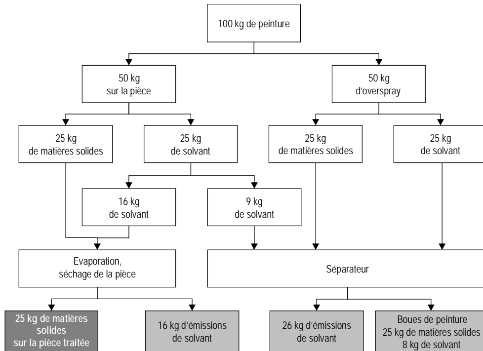
Fig. 8 &gt; Flux de substances lors de l'application par pulvérisation selon une technique conventionnelle
