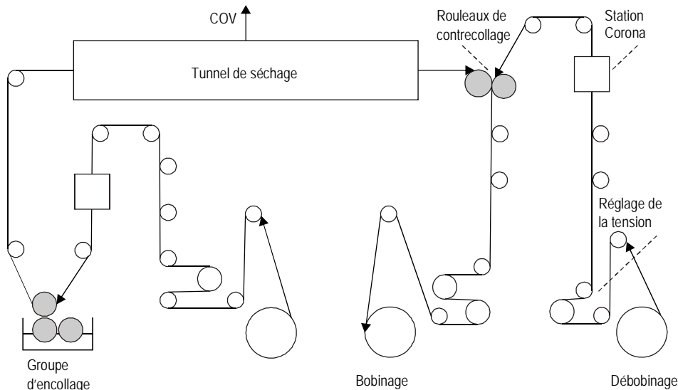
Fig. 12 > Procédé de contrecollage à sec avec des colles à solvants
