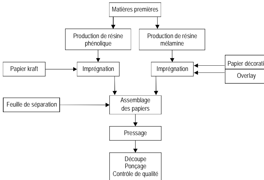
Fig. 14 > Le procédé d'imprégnation
