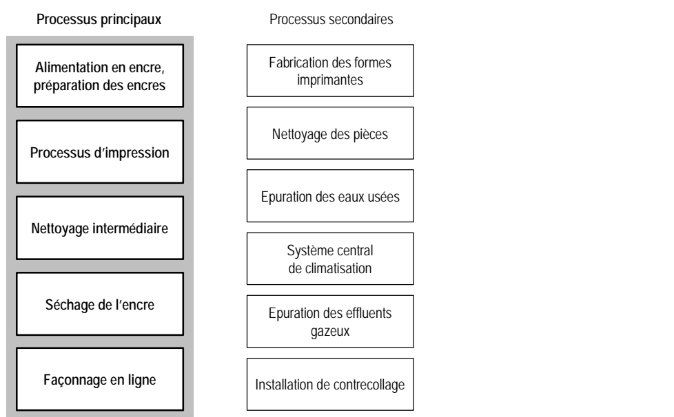
Fig. 2 > Processus principaux et secondaires dans les installations d'impression d'emballages
