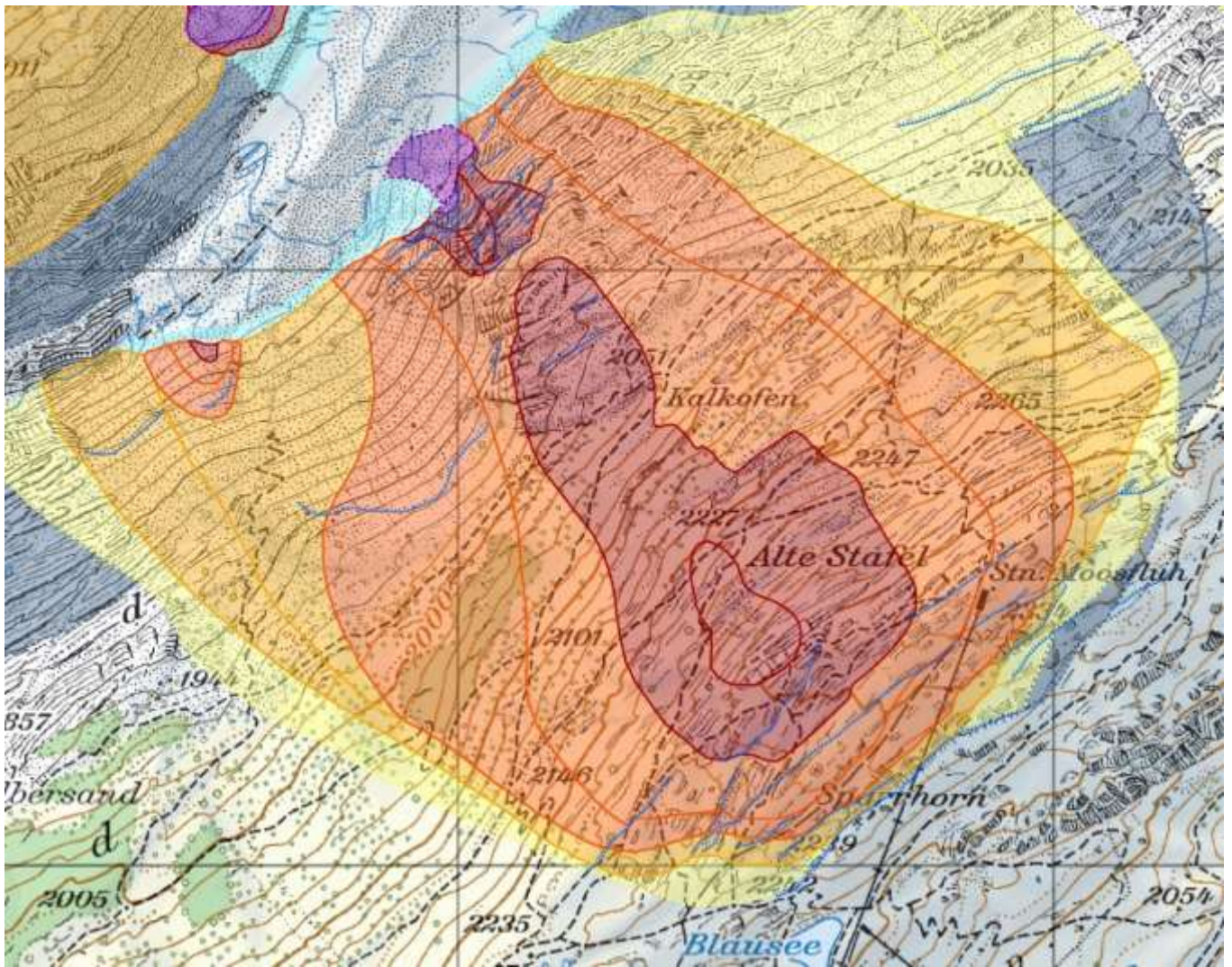
Carte du glissement de terrain de Moosfluh (selon radar INSAR OFEV). Sources: données provenant de radars satellites de 2015 et études de terrain réalisées par l'OFEV.
