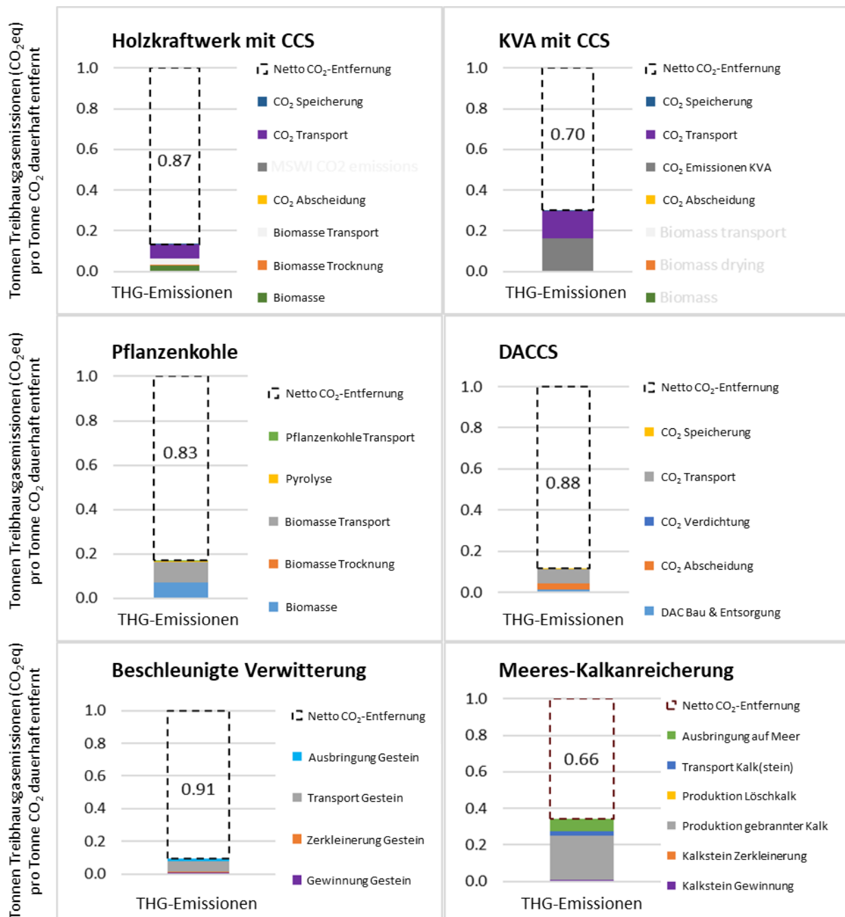
Abbildung 2.1: Lebenszyklus-Treibhausgasemissionen verschiedener CDR-Methoden, berechnet mit einer „realistisch-optimistischen“ Parametereinstellung aus heutiger Sicht der Schweiz. KVA: Kehrlichtverbrennungsanlage; DAC(CS): Direkte Abscheidung (und Speicherung) von Kohlendioxid aus der Luft; THG: Treibhausgas. Alle Methoden gehen von einer Anwendung in der Schweiz aus, mit Ausnahme von Meeres-Kalkanreicherung («Ocean Liming», Norwegen). Biogener Kohlenstoffanteil im Siedlungsabfall: 52%; alle THG-Emissionen im Zusammenhang mit CO 2 -Transport und -Speicherung werden diesem biogenen Kohlenstoffanteil und damit der CDR-Dienstleistung zugerechnet. CO 2 -Abscheidungs-raten: 90% im Holz-kraftwerk, 85% in der KVA. Fichtenholz wird als Biomasse für die Biokohleproduktion und die Holzverbrennung verwendet. Geologische CO 2 -Speicherung in Island für DACCS, Holzverbrennung und MSWI mit CCS angenommen. Transport des CO 2 über eine 4000 km lange Pipeline; CO 2 -Speichertiefe: 3000 m. DAC wird mit Schweizer Netzstrom und Abwärme betrieben. Anlageninterne Wärme- und Stromversorgung für die CO 2 -Abtrennung in den Holzverbrennungs- und KVA-Anlagen. Transport von Biomasse und Gestein im Bereich von rund 100 km. Hochtemperaturwärmeversorgung für die Brennkalkproduktion aus einer Erdgasverbrennung. Spezifische CO 2 -Aufnahme durch verstärkte Gesteinsverwitterung: 0.35 t CO 2 /t Gesteinsmaterial. Die gestrichelt umrahmten Balkenteile über jedem farbigen Balken stellen die Netto-CO 2 -Entfernungsraten dar, d.h. den Anteil des dauerhaft entfernten Brutto-CO 2 , der nicht durch THG-Emissionen aus den CDR-Produktsystemen kompensiert wird.
