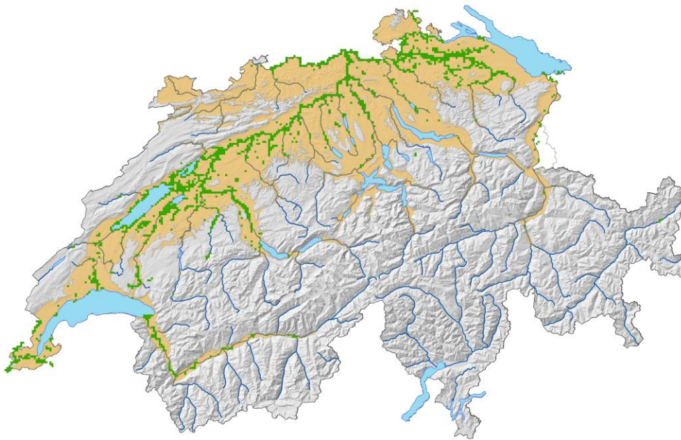
Abb. 27 > Aktuelle (grün) und potentielle (gelb) Verbreitungsgebiete des Bibers
