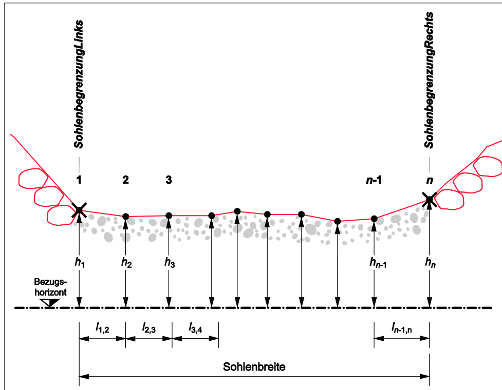
Abb. 45 Ermittlung der mittleren Sohlenlage.
