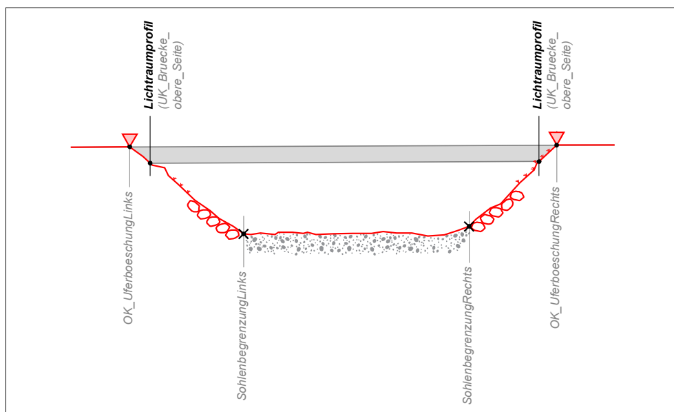
Abb. 22 Lichtraumprofil bei einfachen Brücken.
