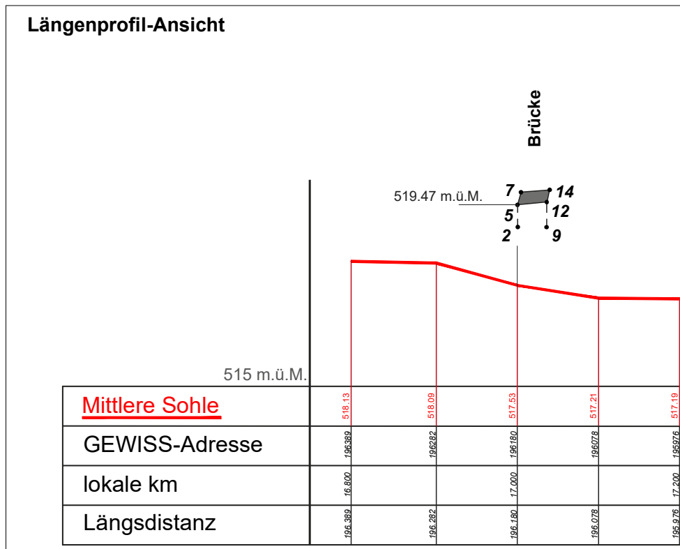
Abb. 40 Darstellung der Brücke im Längenprofil.
