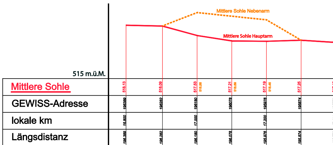
Abb. 47 Längenprofil im Bereich eines Nebenarms.
