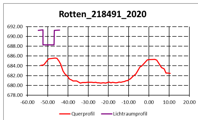
Abb. 37 Beispiel Brückenschnitt, Diagramm des Querprofiles GEWISS_Adr. 218487
