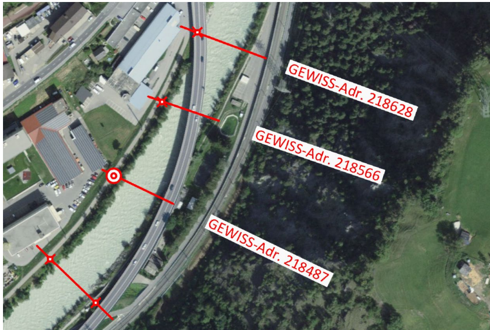
Abb. 33 Beispiel Brückenschnitt, Situation
