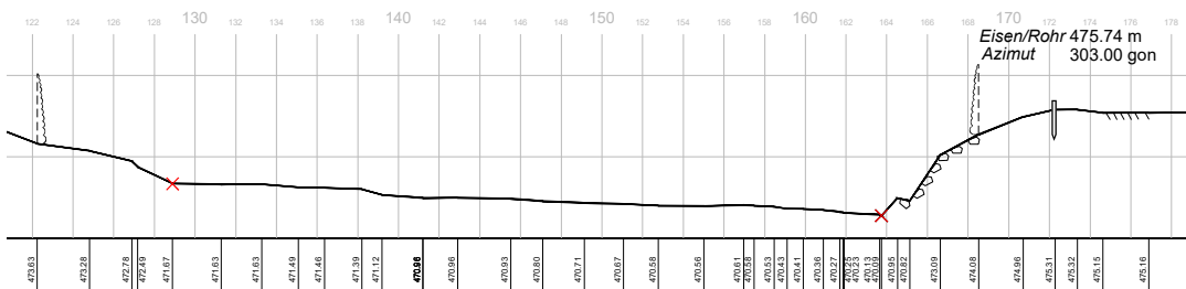
Abb. 14 Sohlenbegrenzung falls der Kolk am Prallhang liegt und der Uferschutz bis in den Kolk hinunter reicht.
