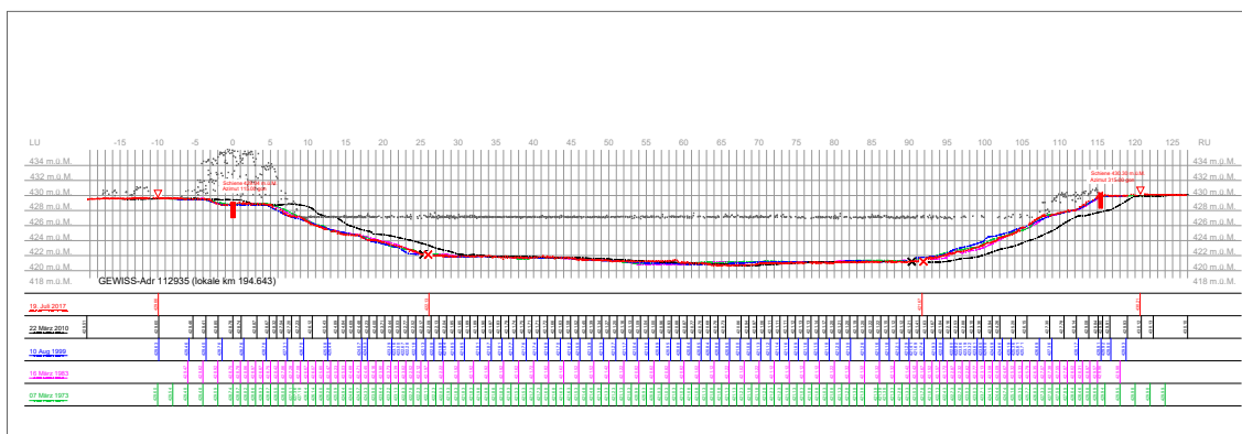
Abb. 58 Querprofil aus der klassifizierten Punktwolke.
