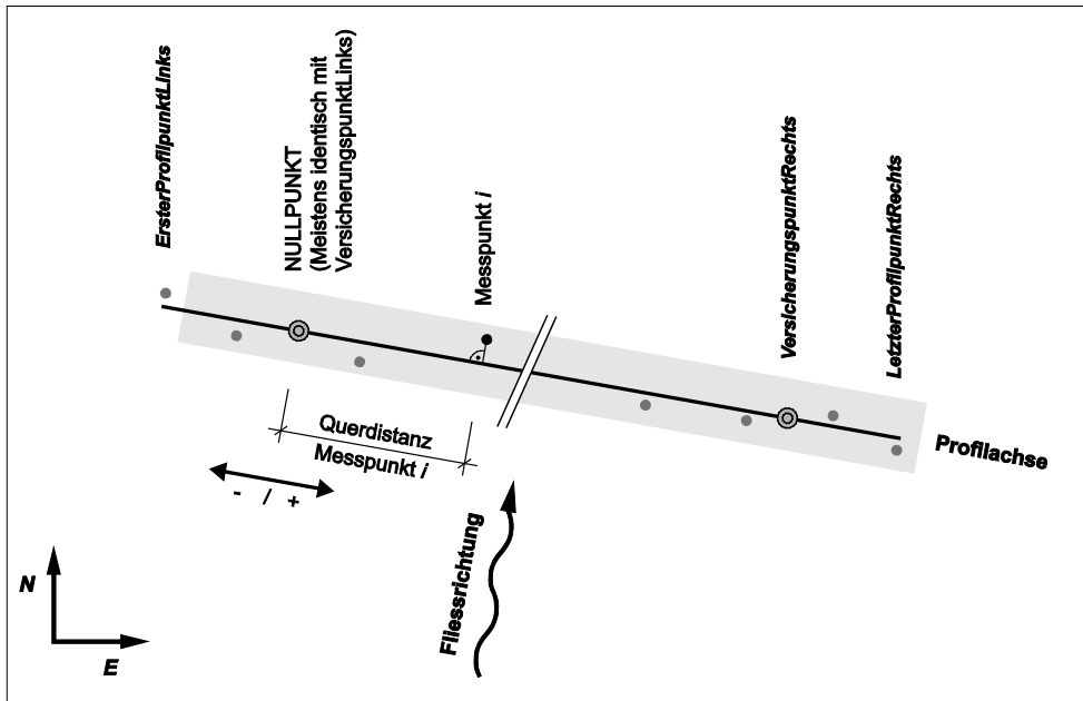
Abb. 12 Definition der berechneten Querdistanz.
