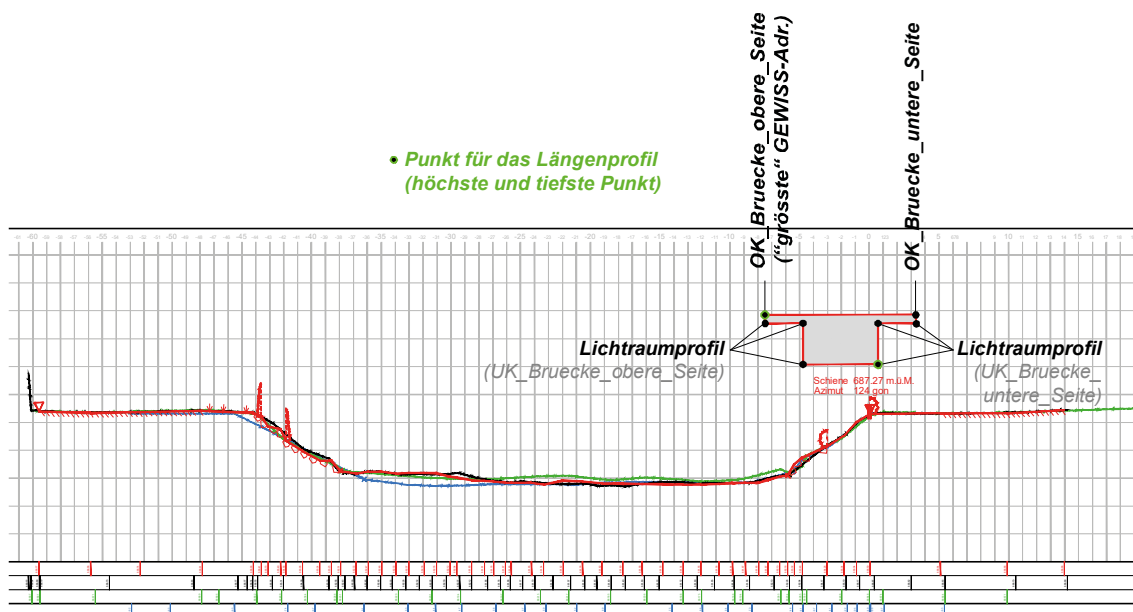
Abb. 34 Beispiel Brückenschnitt, Querprofil GEWISS_Adr. 218628
