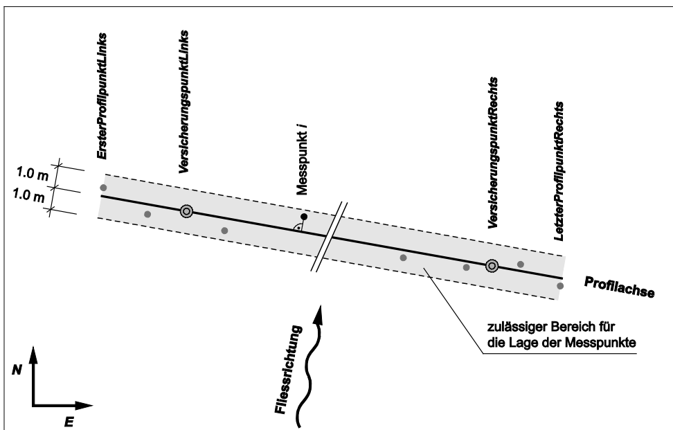
Abb. 11 Zulässiger Bereich für die Lage der Messpunkte.
