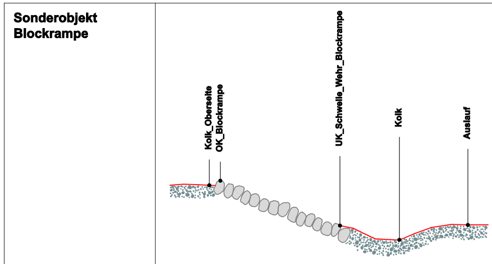
Abb. 7 Sonderobjekte bei Blockrampen.
