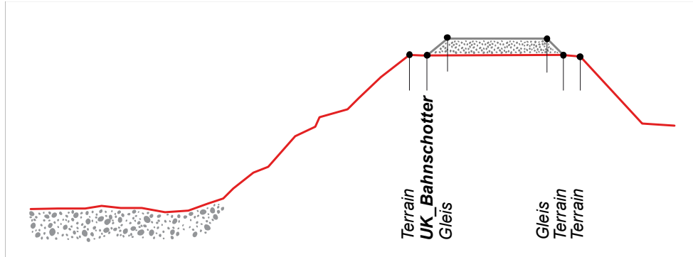
Abb. 43 Verwendung des Attributswerts „UK_Bahnschotter“ zur Kennzeichnung der Begrenzung zwischen einem Bahndamm und dem aufliegenden Bahnschotter.
