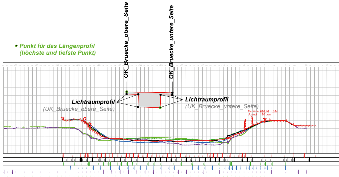
Abb. 35 Beispiel Brückenschnitt, Querprofil GEWISS_Adr. 218566
