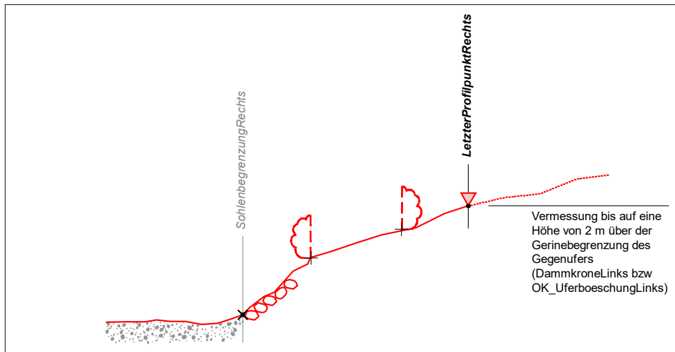
Abb. 20 Gerinnebegrenzung bei ansteigendem Umgelände.
