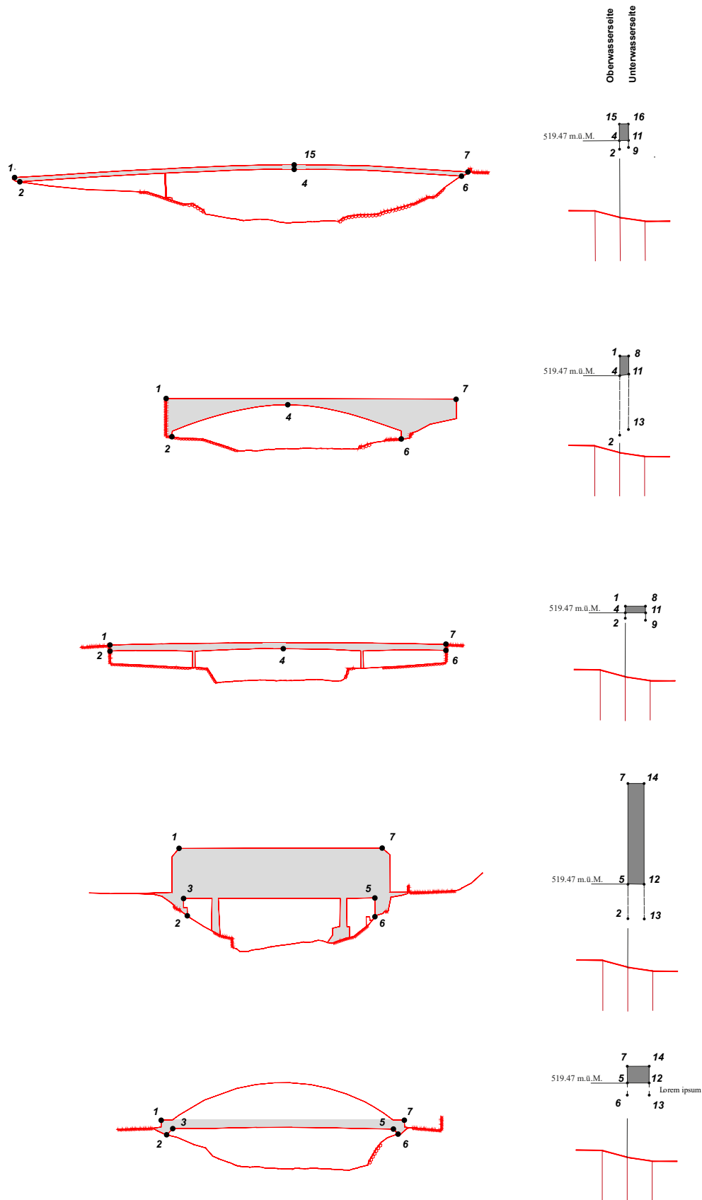
Abb. 41 Beispiele der Darstellung der Brücke im Querprofilplan (links) und im Längsprofilplan (rechts).
