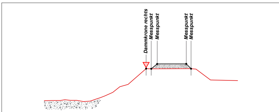
Abb. 21 Punktrolle zur Definition des durchlässigen Bahnschotters.
