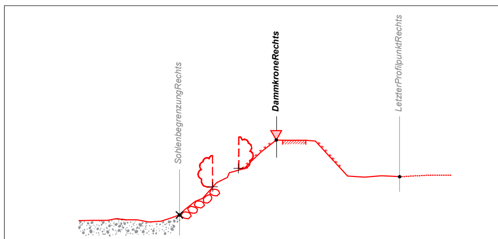
Abb. 19 Gerinnebegrenzung bei vorhandenem Hochwasserdamm.
