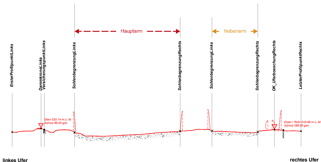
Abb. 17 Definition der Sohlenbegrenzungspunkte für den Haupt- und den Nebenarm in einem geteilten Gerinne (GEWISS_Adresse 196180 aus Abb. 16).
