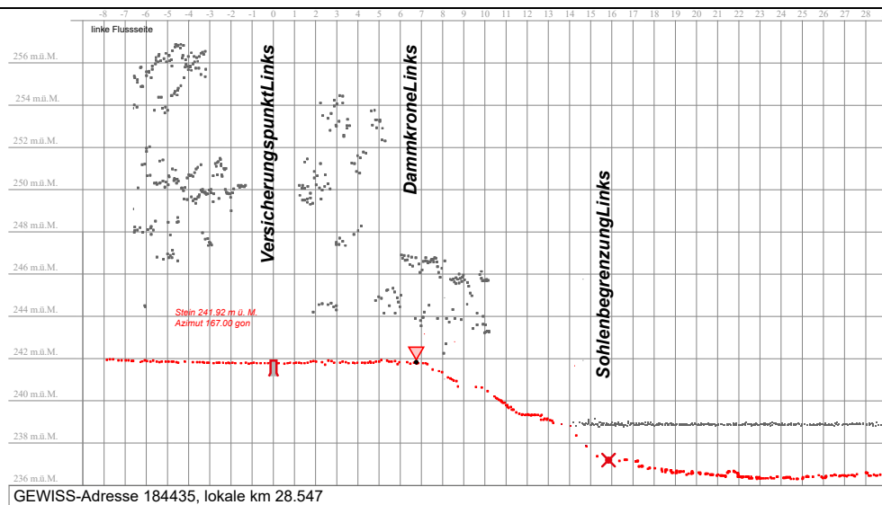
Abb. 51 Definition der Sohlen- und Gerinnebegrenzung im Querprofil.
