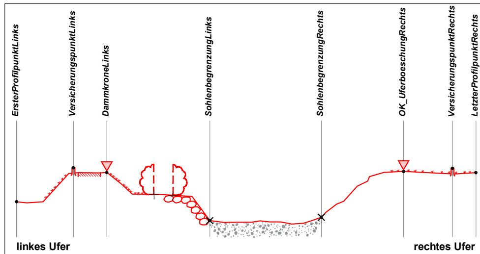
Abb. 13 Beispiel für unterschiedliche Punktrollen.
