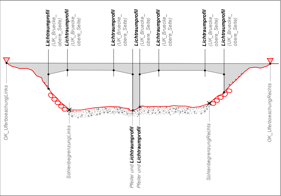
Abb. 24 Lichtraumprofil bei Brücken mit Pfeilern.
