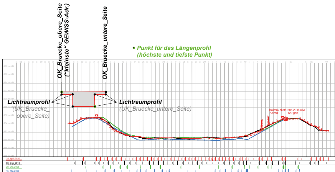
Abb. 36 Beispiel Brückenschnitt, Querprofil GEWISS_Adr. 218487
