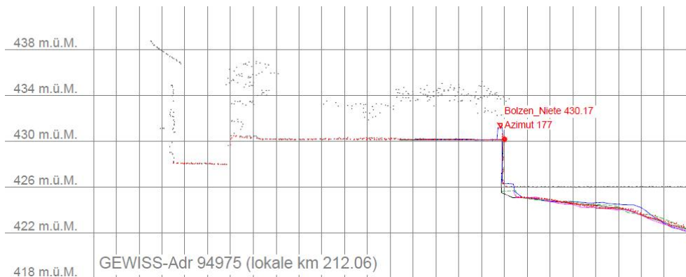
Abb. 52 Definition der Gerinnebegrenzung bei Vorhandensein einer Ufermauer
