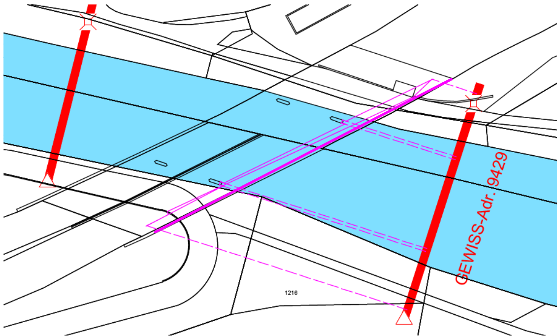
Abb. 27 Beispiel 1 Lichtraumprofil, Situation
