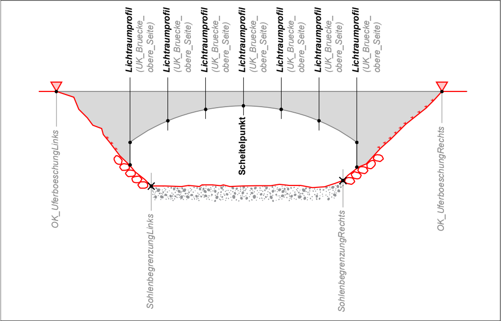
Abb. 23 Lichtraumprofil bei Bogenbrücken.
