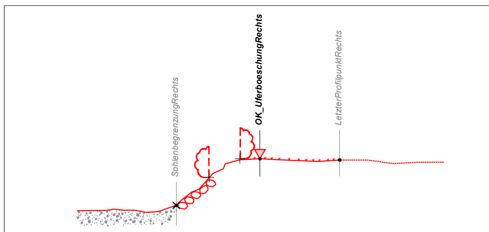
Abb. 18 Gerinnebegrenzung ohne Hochwasserdamm.
