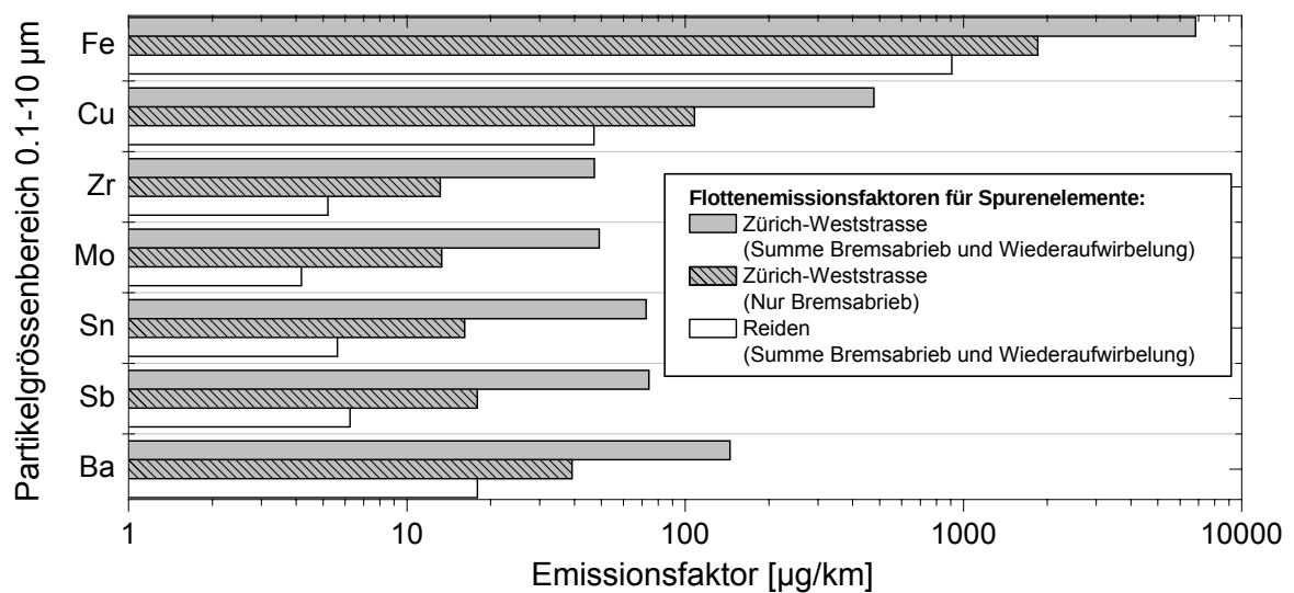
Fig. 1.8: Totale Flottenemissionsfaktoren (Partikelgrößenbereich 0.1 - 10 \mu\text{m} ) für Zürich-Weststrasse (10% SMW) und Reiden (15% SMW), für bremsabriebsbezogene Spurenelemente. Den Werten für Zürich-Weststrasse liegen experimentelle Daten von Februar/März 2007 zugrunde (9 Tage, nur Zeitabschnitte ohne Niederschlag), für Reiden von Oktober 2007 (4 Tage, nur Zeitabschnitte ohne Niederschlag).
