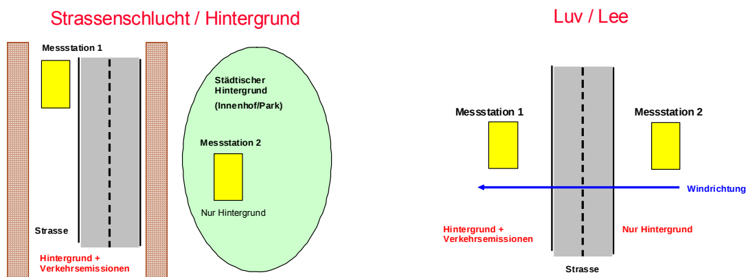
Fig. 1.1: Schematische Darstellung des Strassenrand-Hintergrund-Konzepts (links) und des Lee-Luv-Konzepts (rechts). Die Probenahmehöhe betrug 4.5 m über Boden, basierend auf experimentellen Voraussetzungen (optimierte Ansaugleitungen, freie Anströmbarkeit und Vandalensicherheit).
