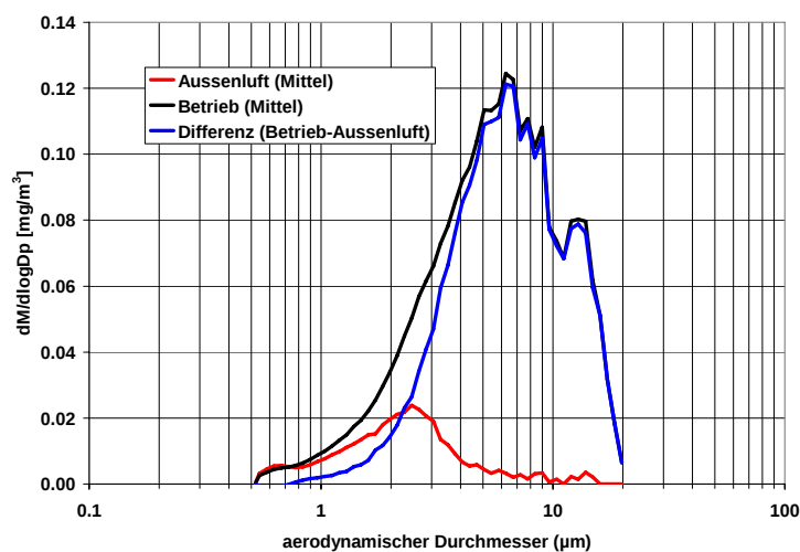
Fig 1.10: Typische Partikelgrössenverteilung im Messbereich 0.5-20 \mu\text{m} aus einem Experiment mit einem Verkehrslastsimulator während einer Versuchsperiode mit dominierendem Strassenabrieb (Aufwirbelung vernachlässigbar). Verglichen mit der Umgebungsluft ist die Grössenverteilung klar Richtung Grobfraktion verschoben.
