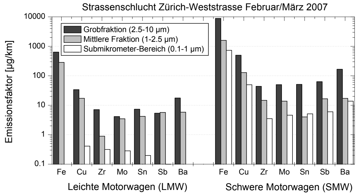
Fig. 1.7: Emissionsfaktoren (EF) für leichte (LMW) und schwere (SMW) Motorfahrzeuge für Zürich-Weststrasse (Strassenschlucht). Der Berechnung lagen 209 Stundenwerte zugrunde ( \sim 9 Tage, \Delta\text{NO}_x > 20 \mu\text{g m}^{-3} , nur Zeitabschnitte ohne Niederschlag). Für Zn wurden keine Emissionsfaktoren berechnet, da dieses Element auch durch nicht verkehrsbedingte Quellen stark beeinflusst war.
