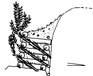
Kastenkonstruktion doppelwandig
