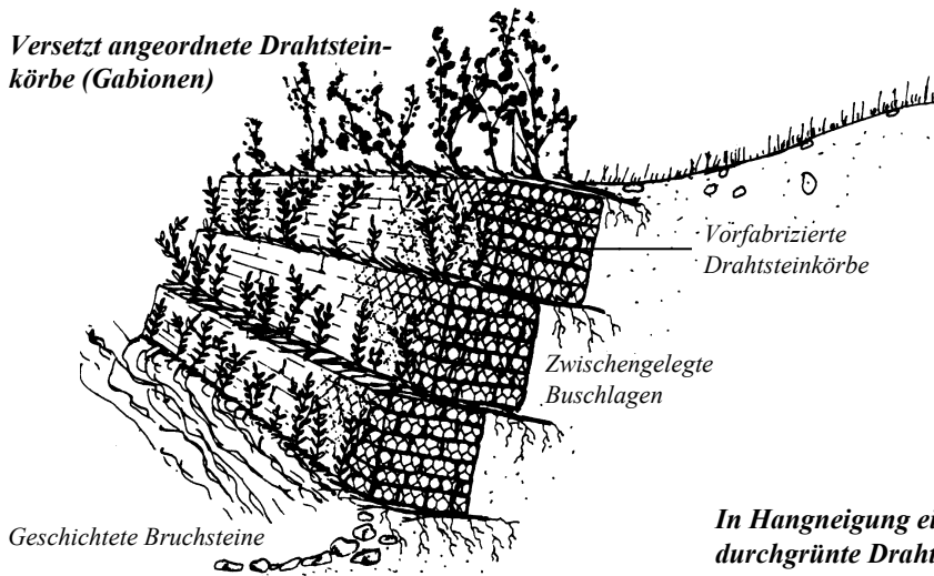
Dem Geländeverlauf angepasster, durchgrünter Drahtsteinkorb
