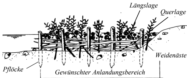
Fertiger Gitterbuschbau im Querschnitt mit eingesteckten Weidenästen
