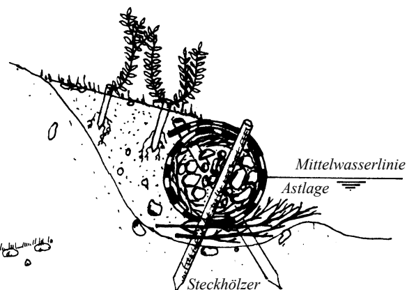
Eingebaute Geotextiluferfaschine mit nachfolgenden Weidensteckhölzern
