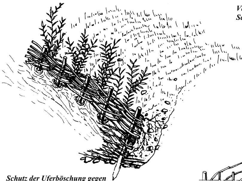
Schutz der Uferböschung gegen Auswaschung durch Flechtzaun und Astlagen
