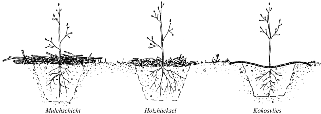
Pionierpflanzung mit Mulch, Holzhäcksel und Kokosvlies
