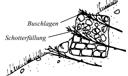
Terrassenartig eingebauter, durchgrünter Drahtsteinkorb
