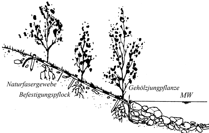
Böschungsschutzmatte bei Gehölzjungpflanzungen
