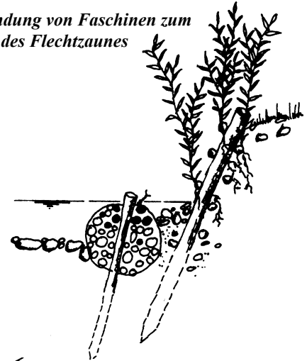
Bau eines Flechtzaunes
