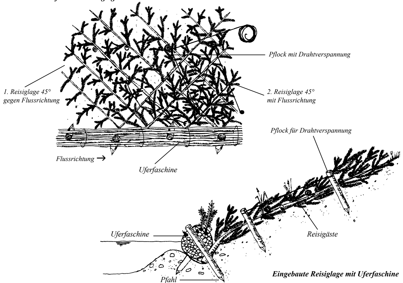
Eine im Bau befindliche Reisiglage
