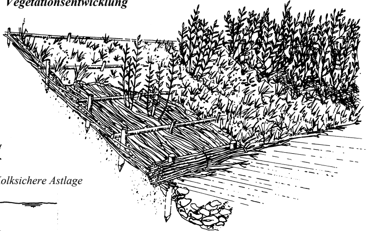
Ansicht der Spreitlage mit fortschreitender Vegetationsentwicklung
