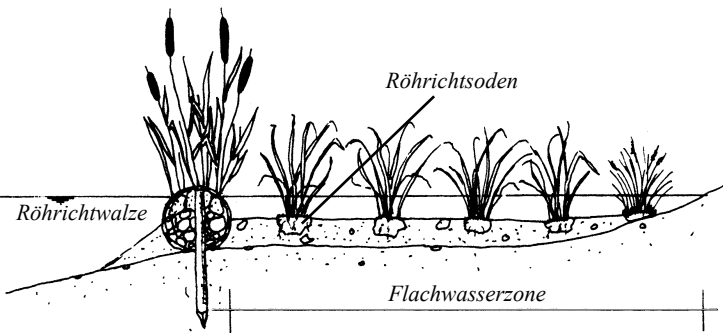
Röhrichtwalze mit nachfolgender, geotextilgesicherter Ballenpflanzung
