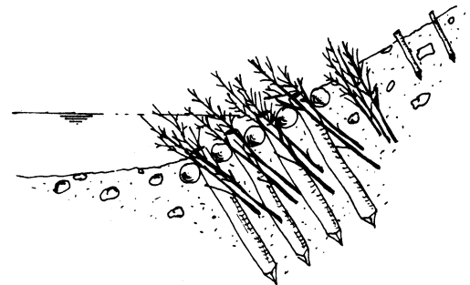
Querschnitt der flach eingebauten Holzkrainerwand
