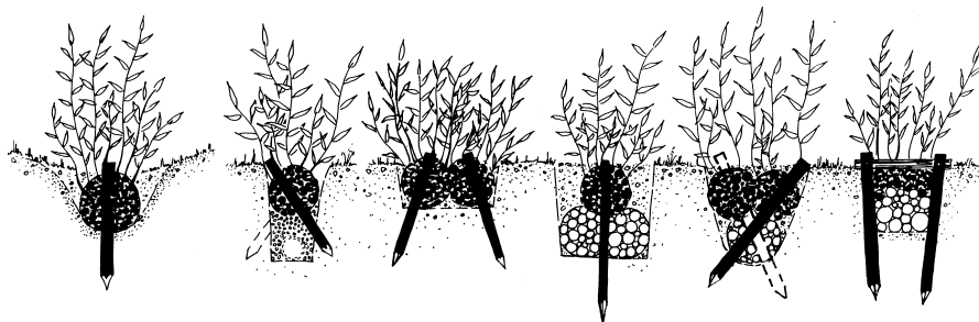
Verschiedene Arten von lebenden Faschinen zur Entwässerung
