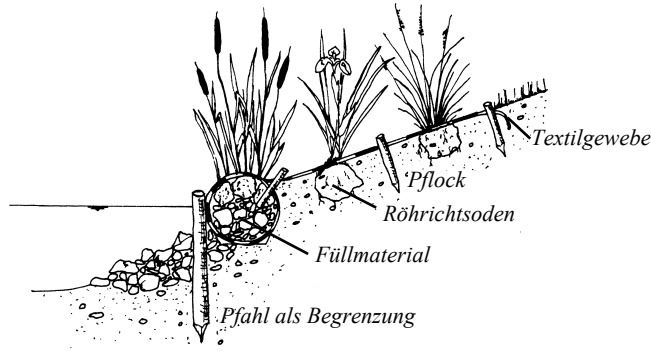
Röhrichtwalze mit nachfolgender, geotextilgesicherter Ballenpflanzung
