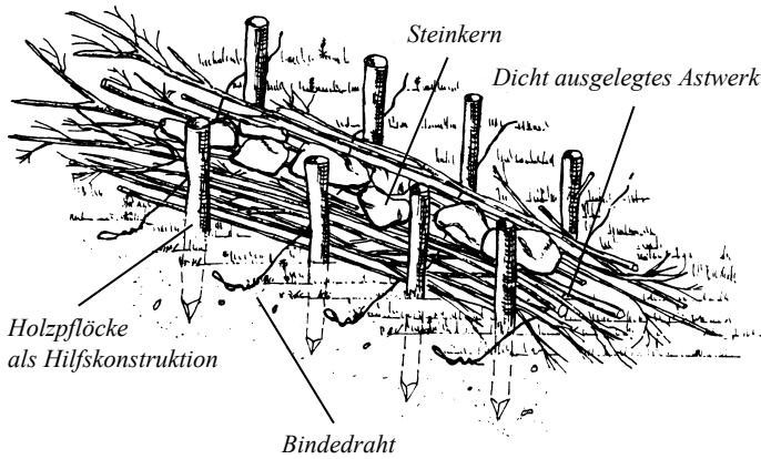
Herstellung einer Senkfaschine zwischen einem Hilfgürtel
