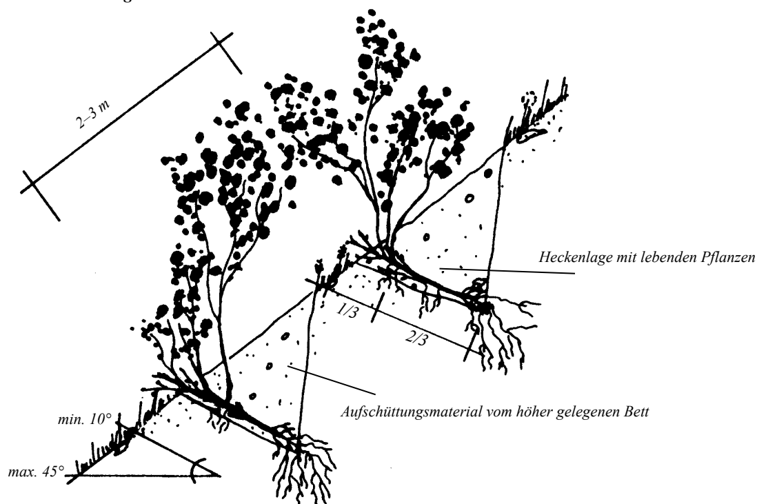
Heckenlage in der Anschnittböschung ca. 60 cm
