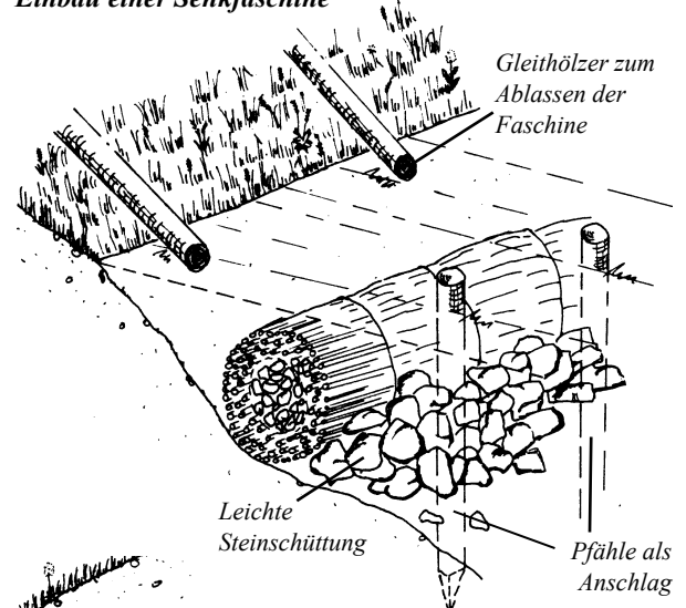
Einbau einer Senkfaschine
