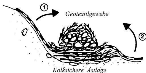
Sackartig eingebaute Röhrriechtwalze mit flexibler Vorderkante
