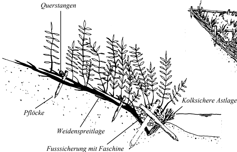
Ansicht der Spreitlage mit fortschreitender Vegetationsentwicklung
