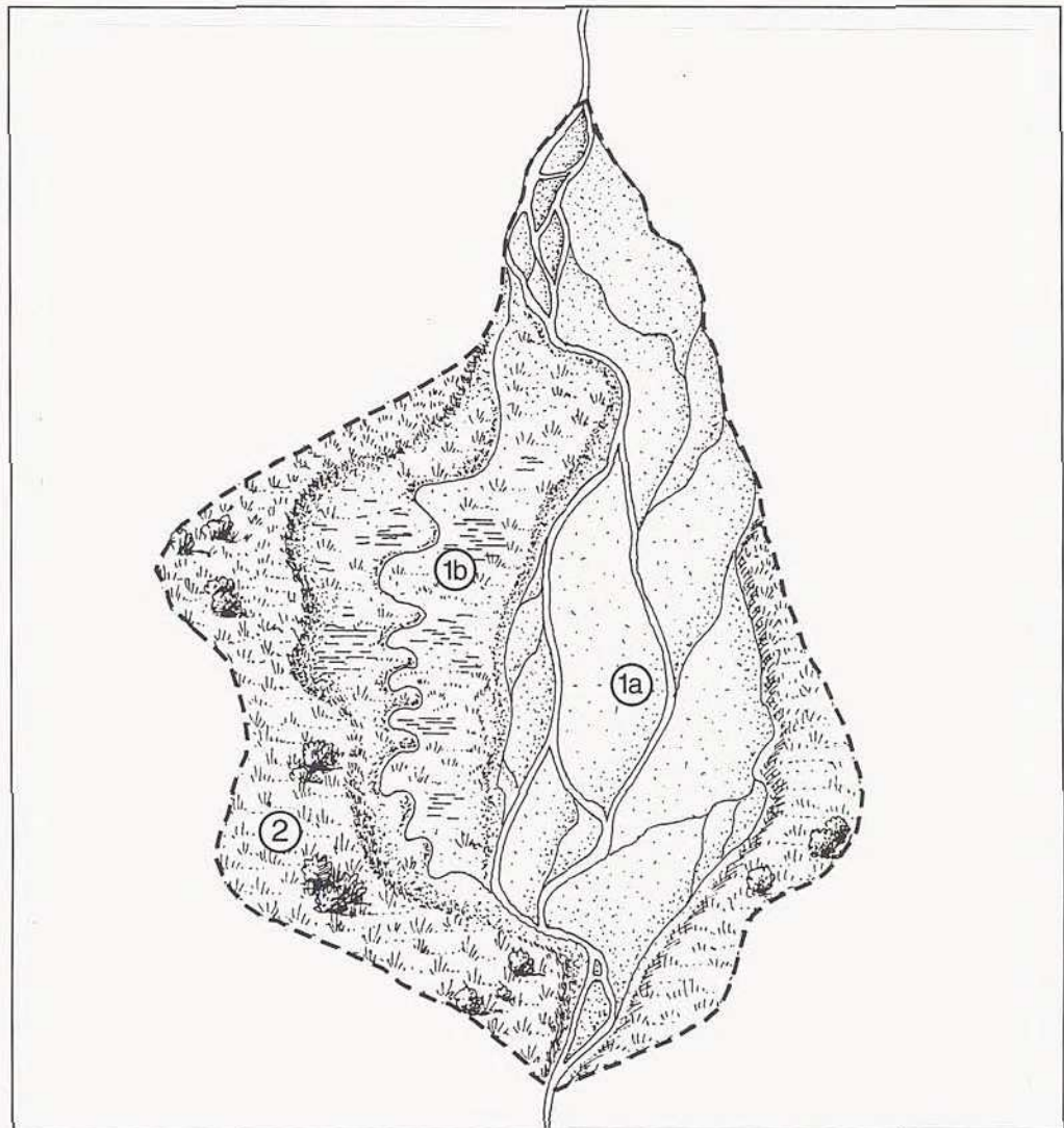
Abbildung 12: Glazifluviale Bereiche: aktuell aktiv (1a), aktuell inaktiv (1b), relik (2)
