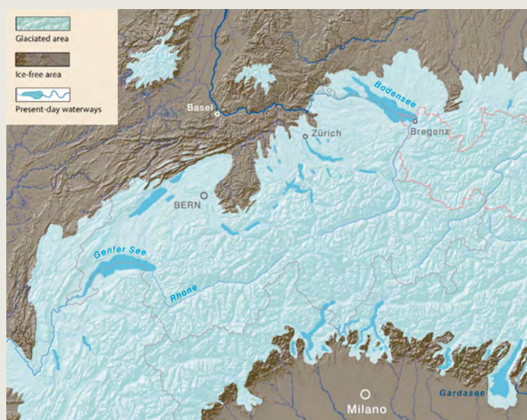
Figure 89: Reconstruction of the maximum glacial extent during the high point of the last ice-age (26 – 20 thousand years ago). Figure adapted from the publication Geologische Bundesanstalt (Hrsg.) (2013): Der Alpenraum zum Höhepunkt der letzten Eiszeit – Posterkarte. Geologische Bundesanstalt, Wien.
