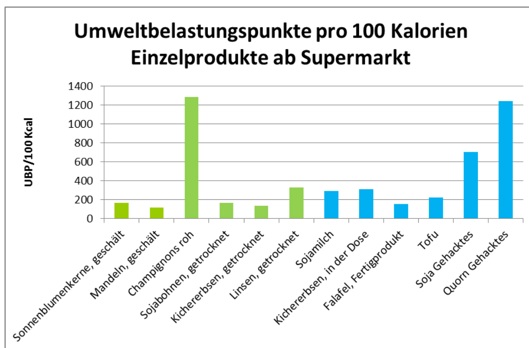
Fig. 4.24: Umweltbelastungspunkte der distribuierten Einzelprodukte (grün) und verarbeiteten Einzelprodukte (hellblau) ab Supermarkt pro Energiegehalt (Kalorien).
