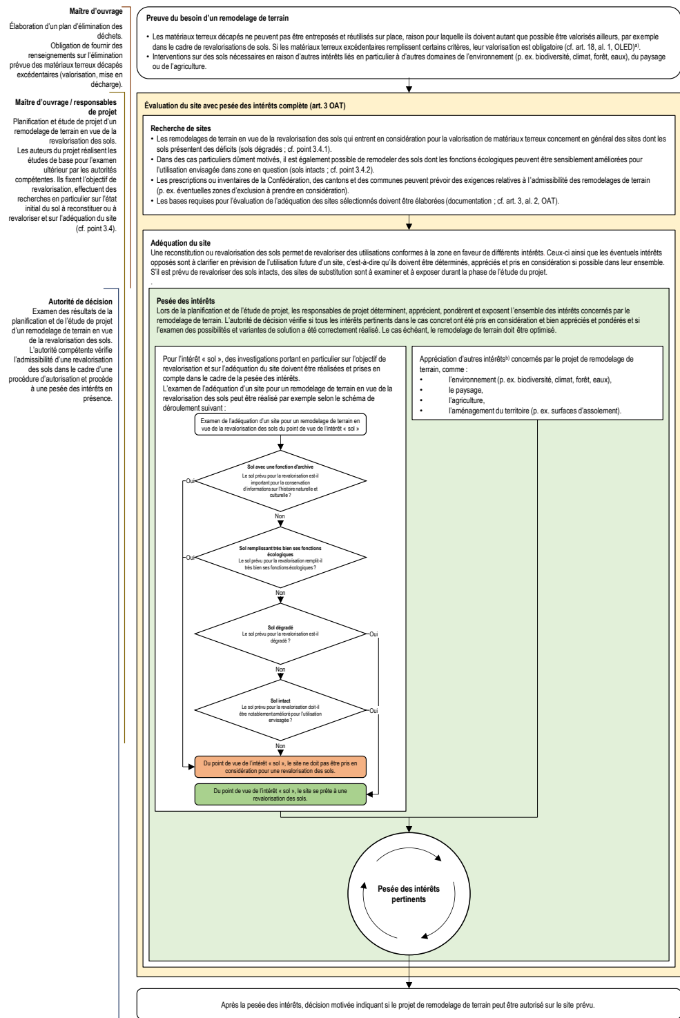
Figure 2 Schéma de la procédure d'évaluation de sites avec pesée des intérêts complète (art. 3 OAT) dans le cadre d'un remodelage de terrain en vue de la revalorisation des sols
