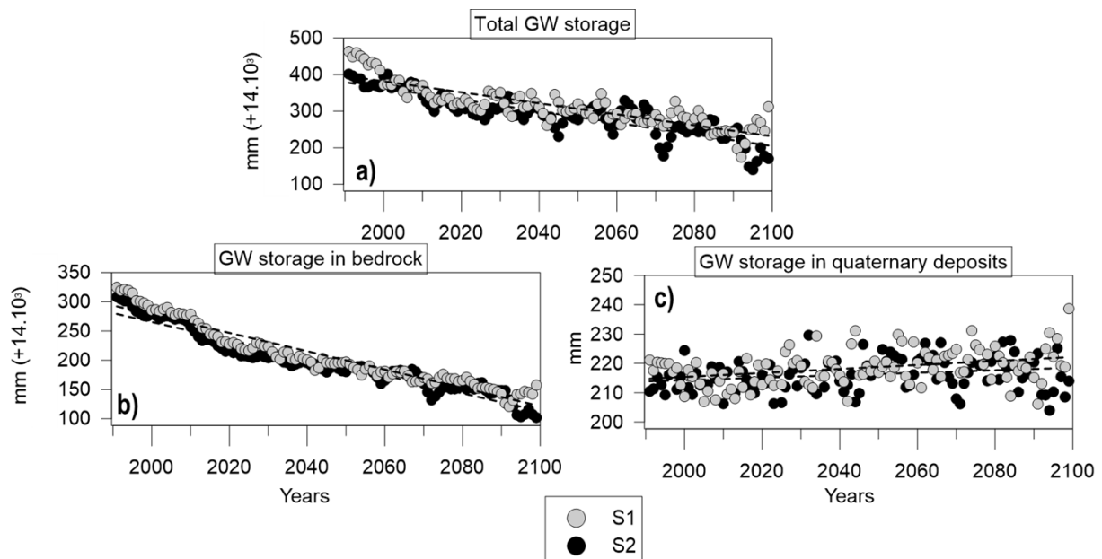
Figure 9. Moyennes annuelles du stockage d'eau souterrain total (a), du stockage dans le socle rocheux peu perméable (b) et du stockage dans les dépôts meubles Quaternaires perméables (c) (Arnoux et al. en prep.).
