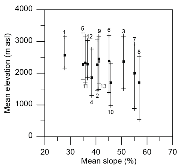
Figure 3 : Altitude (moyenne, minimum et maximum) et pente moyenne des bassins versants (Arnoux et al. 2020a).
