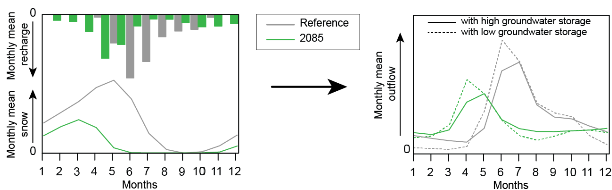
Figure 14. Schéma conceptuel de l'évolution du débit des cours d'eau dans le futur avec une forte augmentation des températures et une diminution des précipitations estivales mettant en évidence le rôle tampon des eaux souterraines (Arnoux et al. 2020a).
