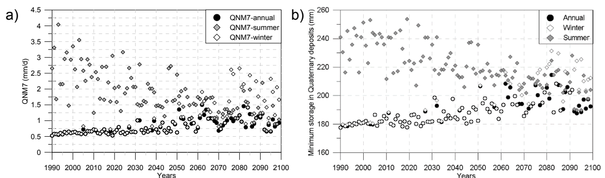
Figure 11 : Débit minimale (a) ou stockage minimale de l'eau souterraine dans les dépôts quaternaires (b) sur sept jours consécutifs par an, à la fin d'été (août-septembre) et à la fin d'hiver (avril-mai) pour S2 (Arnoux et al. en prep.).
