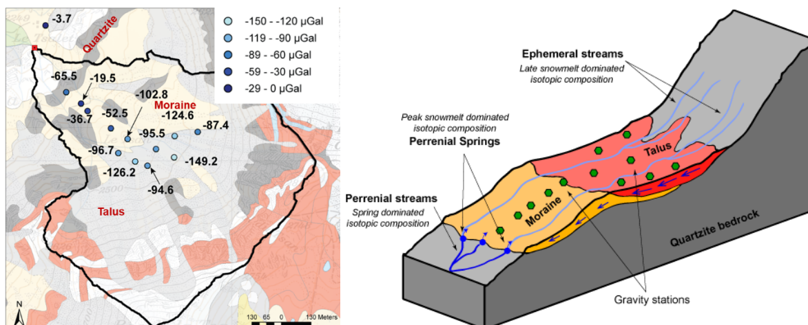
Figure 7. Résultats de l'étude gravimétrique (gauche) ; Changement de la force de gravité entre fin de la période de fonte neige (Juillet) et fin de période de récession estivale (Octobre). Modèle conceptuel du fonctionnement hydrogéologique du sous bassin étudié (droite) ; voir Arnoux et al. 2020b pour plus de détails
