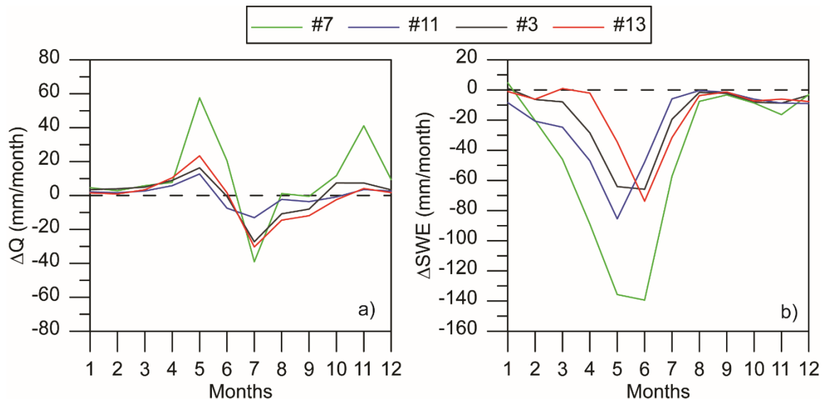
Figure 4 : (a) Changement des débits mensuels moyens mesurés et (b) de la quantité de neige modélisée exprimée en lame d'eau (SWE), entre la période de 30 années de 1988-2017 et 1968-1999 pour quatre bassins alpins. La quantité de neige a été modélisée avec le modèle de neige inclus dans HBV-light à partir de données fournies par le SLF sur 3 ans et des données climatiques historiques (Arnoux et al. 2020a).
