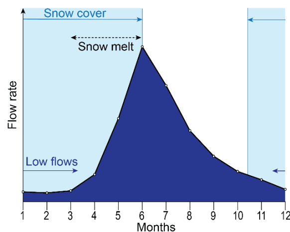
Figure 1. Illustration du hydrographe moyen mensuel typique des bassins versants alpins dominés par la fonte de neige, exemple du bassin Goneri-Oberwald (droite).
