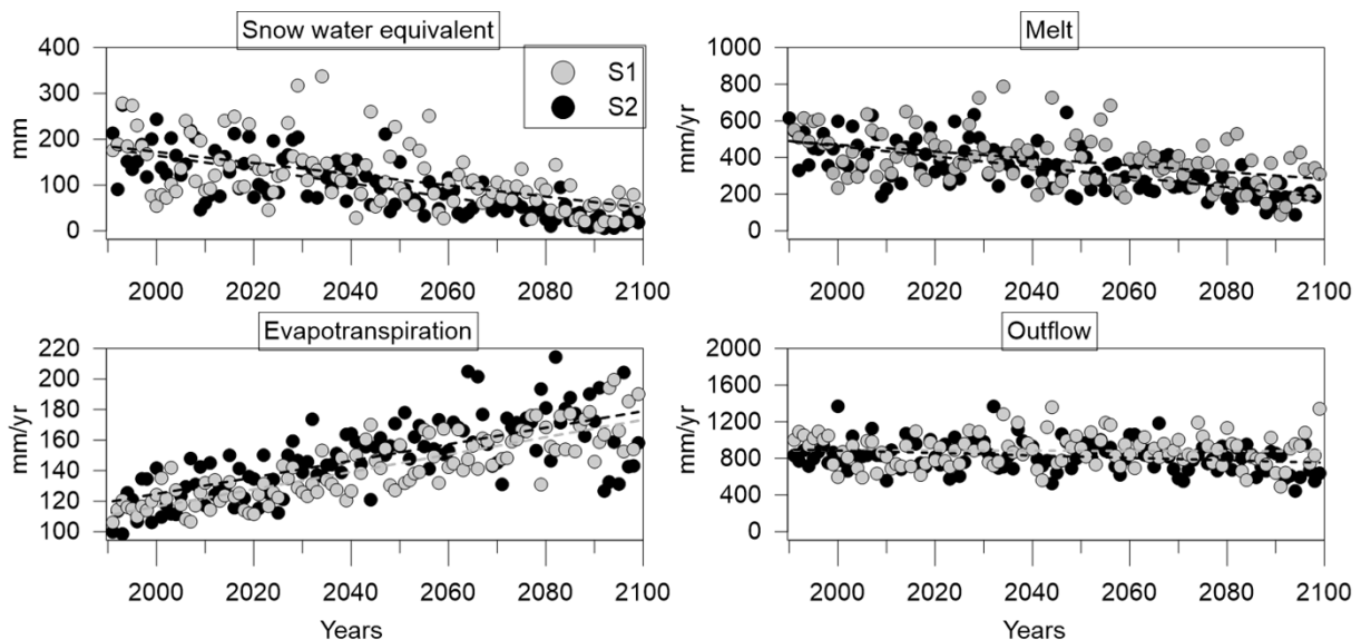
Figure 8 : Moyennes annuels de l'équivalent en eau de la neige (SWE), de la fonte, de l'évapotranspiration (ET), du débit à l'exutoire du bassin dans le bassin de recherche (Réchy) pour deux scénarios climatiques (voir Tableau 2) (Arnoux et al. en prep.).
