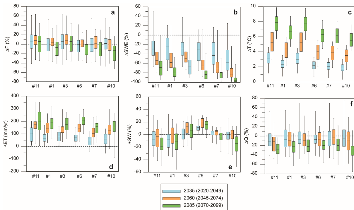
Figure 12 : Variation des précipitations annuelles moyennes (a), de l'équivalent en eau de la neige (b), de la température (c), de l'évapotranspiration (d), du stockage des eaux souterraines (e), du débit (f) pour les bassins versants n° 11, n° 1, n° 3, n° 6, n° 7 et n° 10 pour les 3 périodes futures : 2035 (2020-2049) en bleu, 2060 (2045-2074) en orange et 2085 (2070-2099) en vert, par rapport à la période de référence (1982-2011) pour le scénario S2 (Arnoux et al. 2020a).
