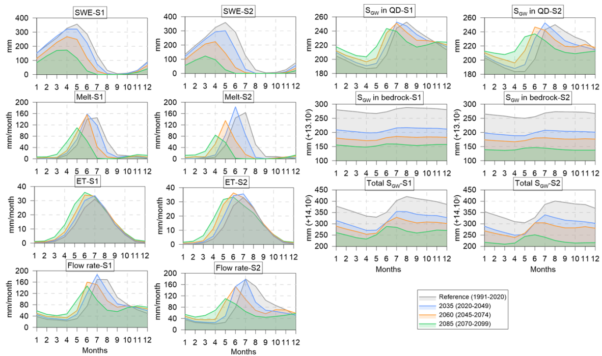
Figure 10. Evolutions saisonnières selon les deux scénarios RCP 8.5, S1 and S2 pour le bassin de recherche (Réchy). Moyennes saisonnières de l'équivalent en eau de la neige (SWE), de la fonte (Melt), de l'évapotranspiration (ET), du débit à l'exutoire du bassin (Flow rate), du stockage souterrain ( S_{GW} ) dans les dépôts Quaternaires perméables (QD), dans le socle rocheux peu perméable (bedrock) et le stockage souterrain total (voir Arnoux et al. en prep. pour plus de détails). Les unités du stockage souterrain représentent la quantité d'eau présente dans les différents réservoirs souterrains normalisée à la taille du bassin versant, ici les variations relatives sont importantes, les valeurs absolues dépendent du volume des couches géologiques et de leur porosité.
