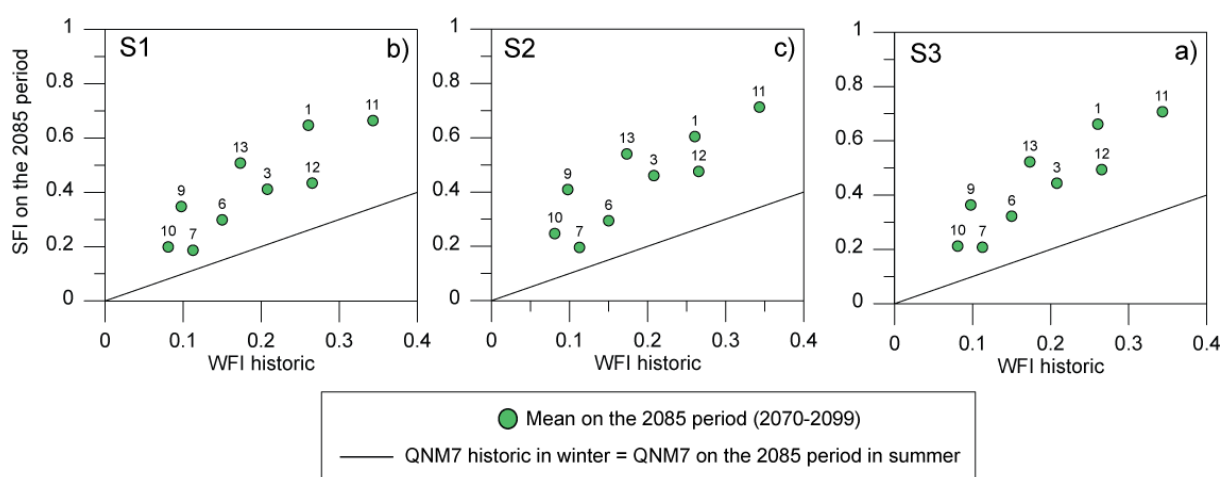
Figure 13. SFI (débit minimal d'été moyen sur sept jours consécutifs divisé pour le débit moyen annuel) pour la période 2085 pour a) S1, b) S2, et c) S3, contre WFI (débit minimal d'hiver moyen sur sept jours consécutifs divisé pour le débit moyen annuel) historique calculé sur les périodes de surveillance des bassins versants (Arnoux et al. 2020a).
