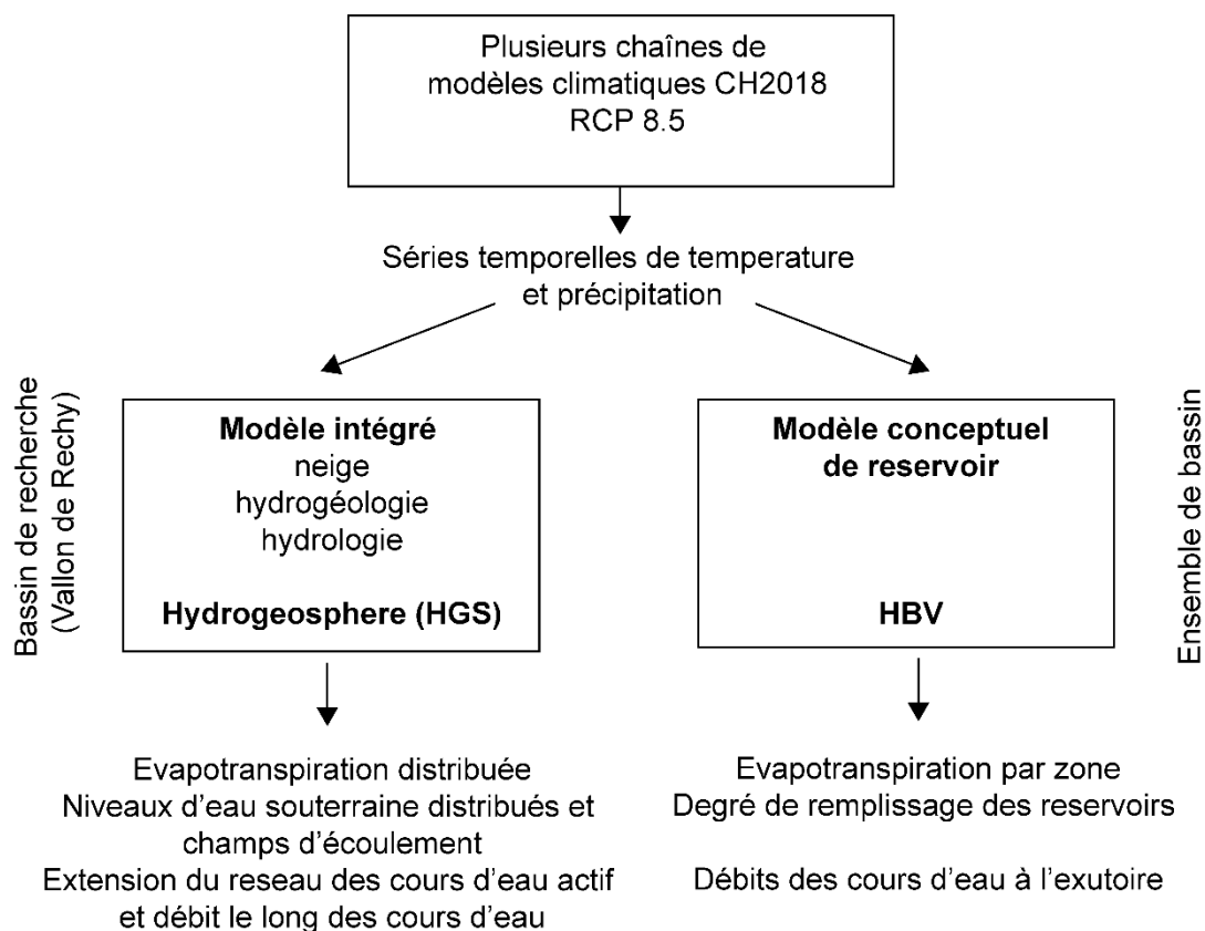
Figure 5 : Vue d'ensemble des approches de modélisation. Des données provenant des modèles climatiques (RCP8.5) ont été intégrés dans des modèles hydrologiques et hydrogéologiques. Pour le bassin de recherche, une modèle intégré (HGS) a été utilisé pour simuler explicitement l'hydrodynamique des différents aquifères et son impact sur l'écoulement de surface. Pour dix bassins, une approche simplifiée a été utilisé sur la base d'un modèle hydrologiques conceptuel à réservoirs (HBV-light).
