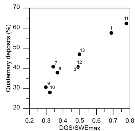
Figure 6. (a) Illustration de l'hydrogéologie simplifiée des milieux alpins, modifiée de Vincent et al. (2019). Relation entre le pourcentage de dépôts quaternaires et (b) un indice pour l'écoulement en hiver (WFI) ou (c) le stockage d'eau souterraine à l'échelle saisonnière (DGS) normalisé par la quantité de neige maximale (SWE max ) pour 13 petits bassins alpins Suisses (Arnoux et al. 2020a pour plus de détails).
