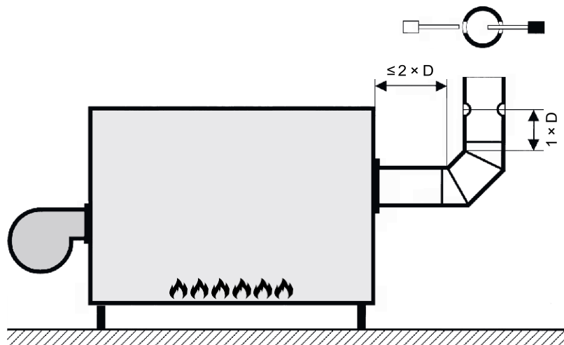
Figure 2: Mesure sur un conduit de fumée rectiligne trop court avant un coude (installations de combustion alimentées à l'huile et au gaz)
