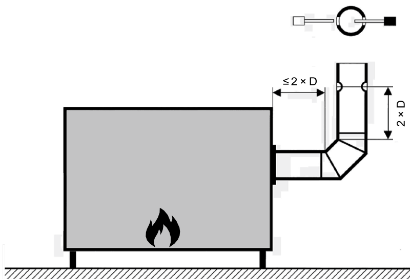
Figure 3: Mesure sur un conduit de fumée rectiligne trop court avant un coude (installations de combustion alimentées au bois)
