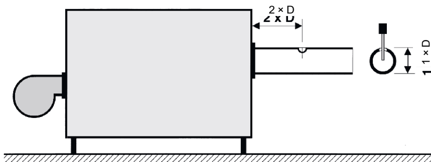
Figure 1: Mesure sur un conduit de fumée rectiligne suffisamment long avant un coude (installations de combustion alimentées à l'huile, au gaz ou au bois)
