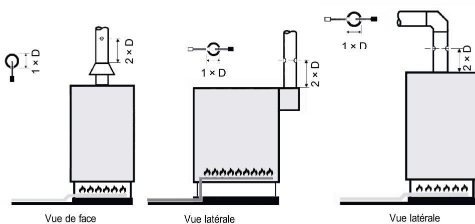
Figure 4: Emplacement de l'orifice de mesure après un générateur de chaleur atmosphérique à gaz doté d'un coupe-tirage
