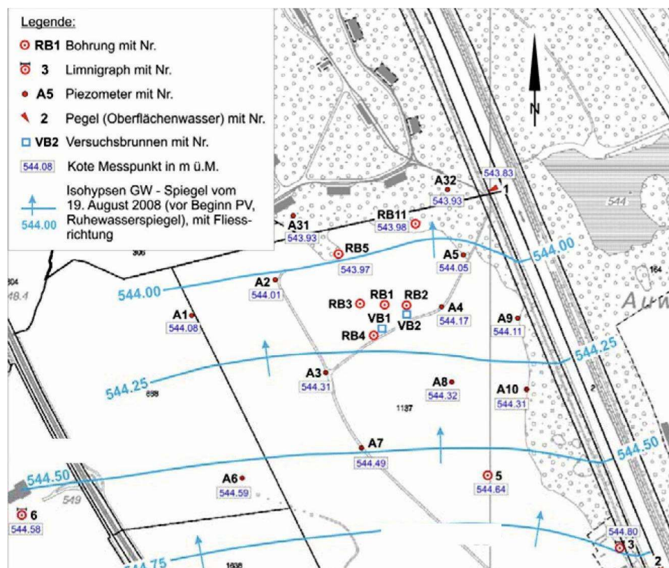
Abbildung 2: Die Veränderung der Grundwasserisohypsen muss für die Projekteingabe dargestellt werden. (Planausschnitt: Kellerhals + Häfeli AG)
