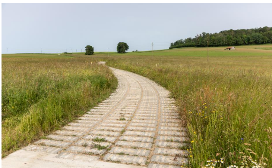
Abbildung 6: Sickerfähige Strasse mit Betonelementen (Foto: LIN'eco)
