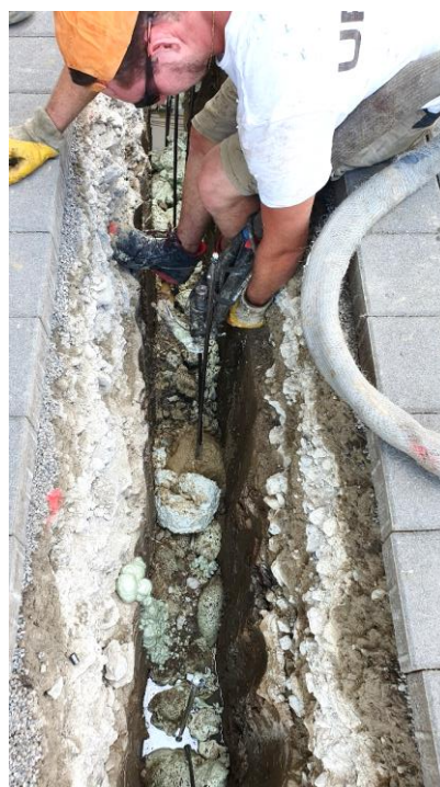
Injektionsarbeiten für 2. Bohrreihe
