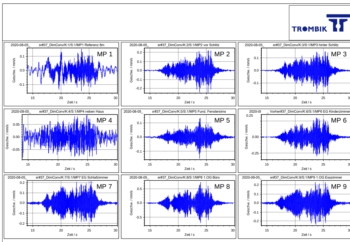
Zeitverlauf MP 1-9, z-Komp. für IC um 14:22 Uhr auf Gleis 2
