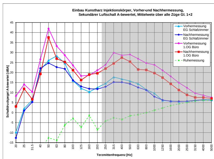
Terzspektren der mittleren Schalldruckpegel Vorher- und Nachhermessung
