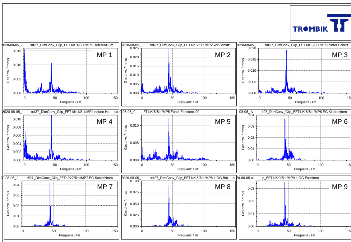
Schmalbandspektren MP 1-9, z-Komp. für IC um 14:22 Uhr auf Gleis 2
