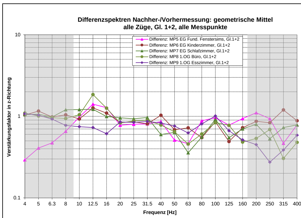
Differenzen der geom. Mittel der Gebäudemesspunkte Nachher- zu Vorhermessung
