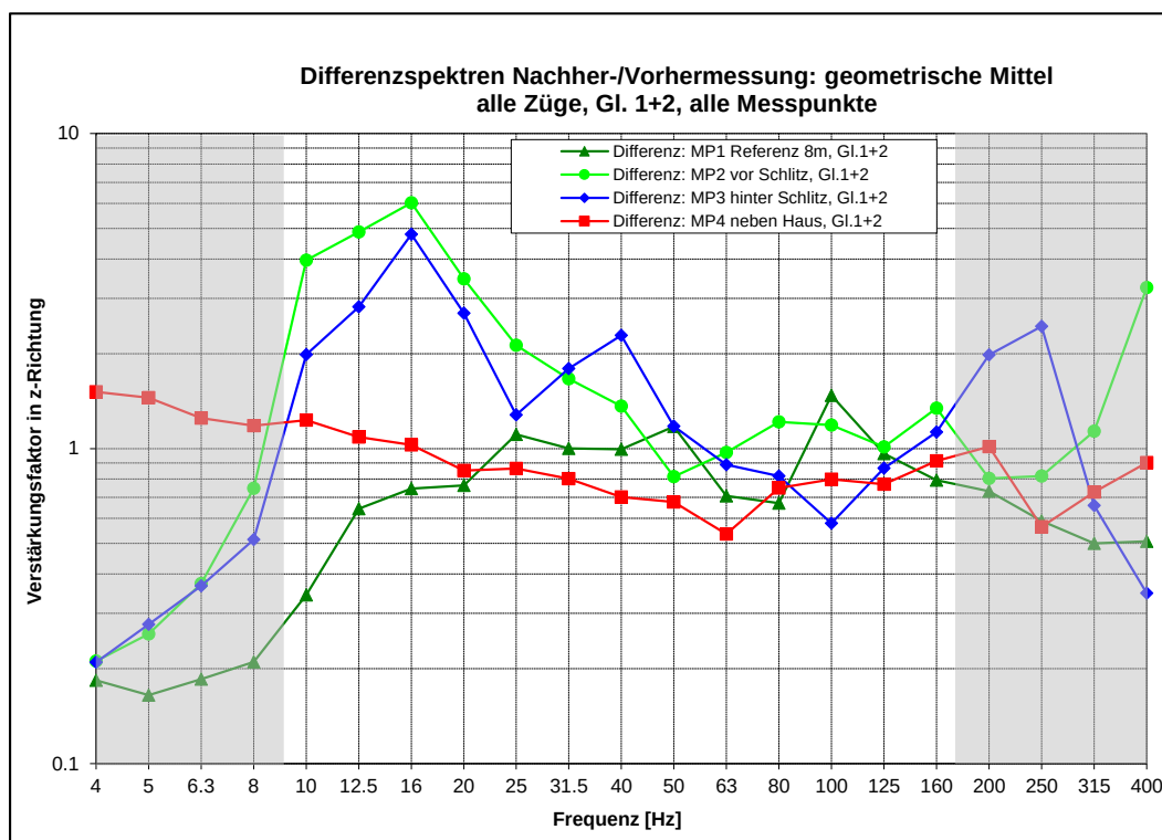
Differenzen der geom. Mittel der Aussenmesspunkte Nachher- zu Vorhermessung
