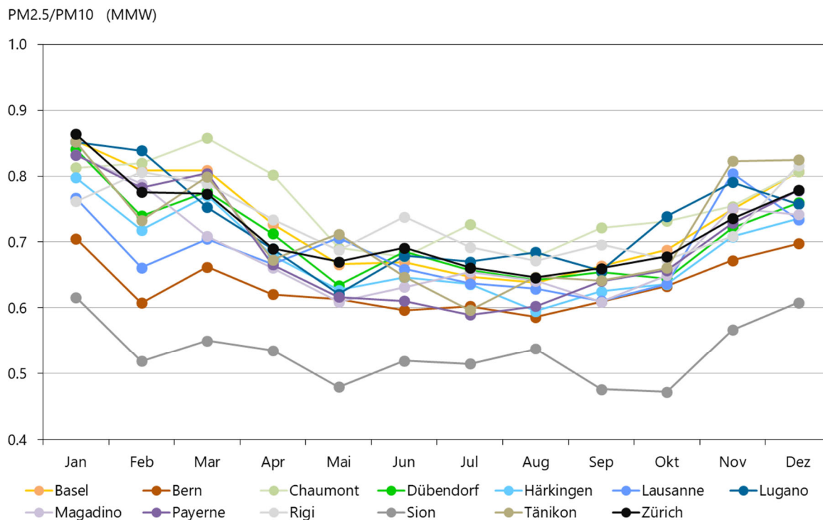
Abb. 8: Durchschnittlicher Jahresverlauf der Monatsmittelwerte der PM2.5/PM10-Verhältnisse in der Zeitperiode 2003- 2021
