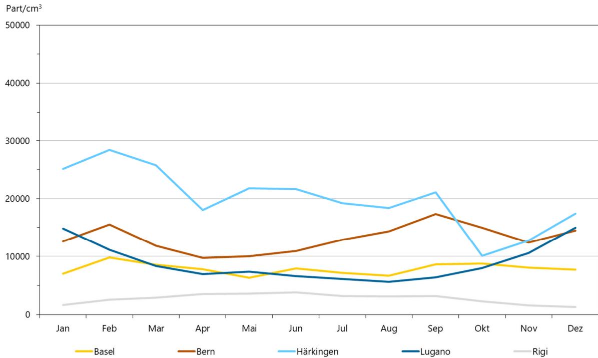
Abb. 13: Jahresverlauf der Monatsmittelwerte der Partikelkonzentration im Jahr 2021
