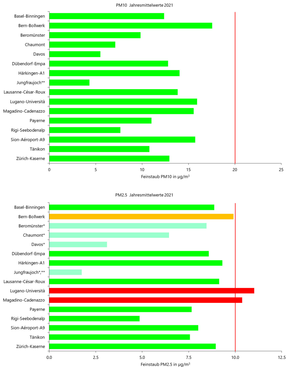
Abb. 2: Vergleich der Jahresmittelwerte 2021 von PM10 (oben) und PM2.5 (unten) mit den Immissionsgrenzwerten (PM10 Grenzwert: 20 µg/m³; PM2.5 Grenzwert: 10 µg/m³).
