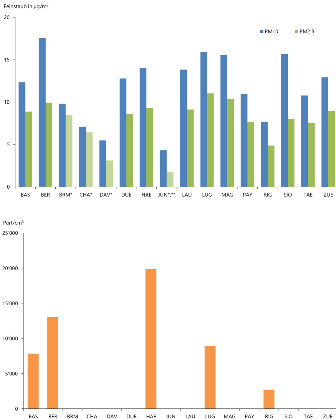
Abb. 1: Übersicht über die Jahresmittelwerte 2021 von PM10 und PM2.5 (oben;) und die Jahresmittelwerte 2021 der Partikelanzahlkonzentrationen (unten).
