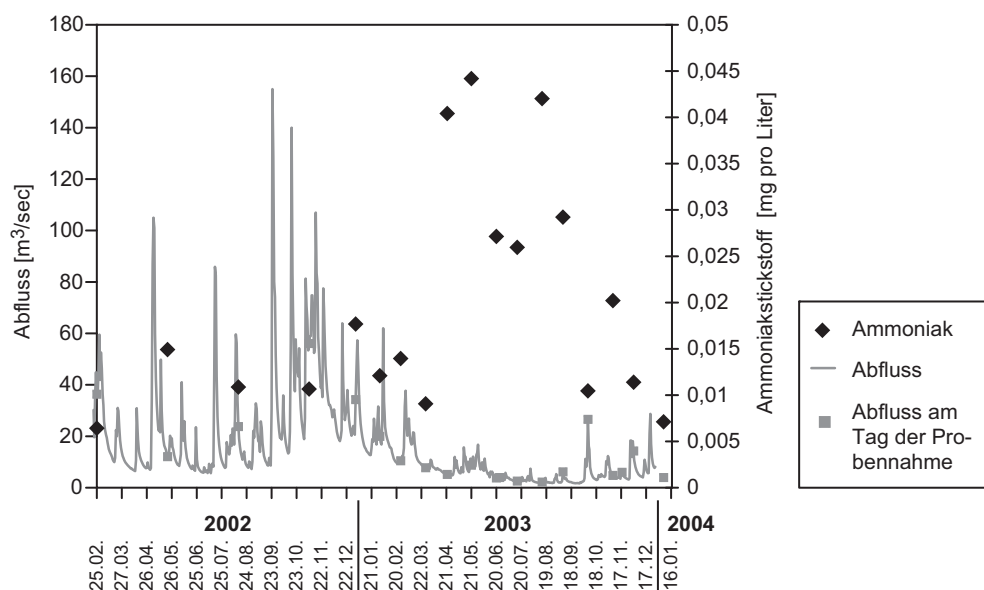
Abb. 4.12: Belastung der Birs am Birskopf mit Ammoniak von Februar 2002 bis Januar 2004. Die im Frühjahr/ Sommer 2003 beobachteten Ammoniak-Konzentrationen liegen in einem Bereich, der Edelfische gefährden kann. Dies gilt insbesondere für deren Laich und die Jungfische. (Daten: AUE-Labor Basel-Stadt)
