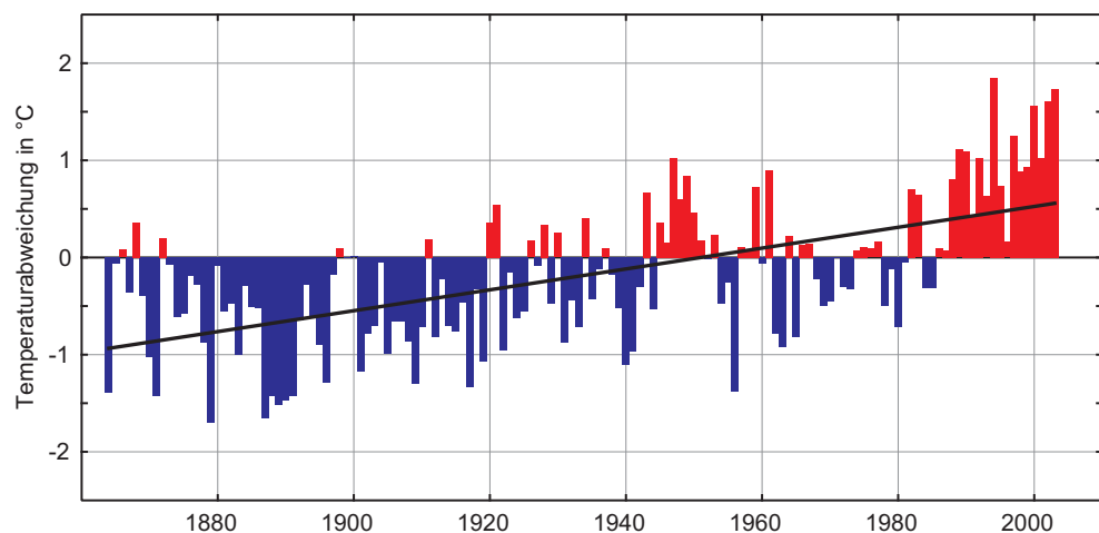
Abb. 1.17: Jährliche Abweichung der Temperatur in der Schweiz von der Jahresnorm 1961–1990. Die zu warmen Jahre sind rot, die zu kalten Jahre blau angegeben. Der lineare Trend der Tempe- ratur zwischen 1864 und 2003 beträgt +1,1\text{ }^{\circ}\text{C} pro 100 Jahre (schwarze Linie). Als Datengrundlage dienten ausschliesslich homogene Temperaturreihen 4,23 .
