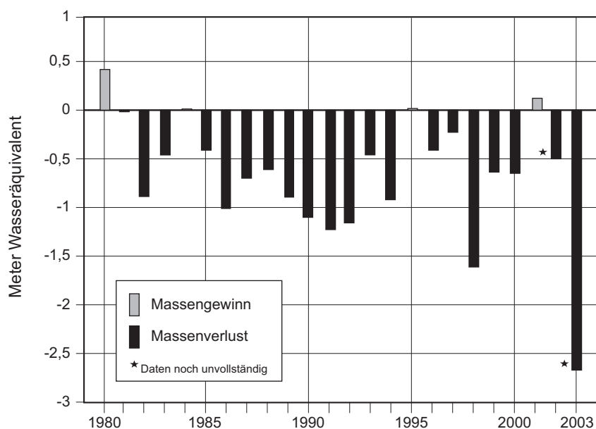
Abb. 2.2: Massenverlust der Alpen- gletscher seit 1980. Die Mittelwerte wurden mit Hilfe der jährlichen Massenbilanz folgender Gletscher berech- net: St Sorlin (F), Sarennes (F), Silvretta (CH), Gries (CH), Sonnblickkees (A), Ver- nagtferner (A), Kesselwand- ferner (A) Hintereisferner (A), Caresèr (I). Datenquelle: Regula Frauenfelder, World Glacier Monitoring Service, Zürich.
