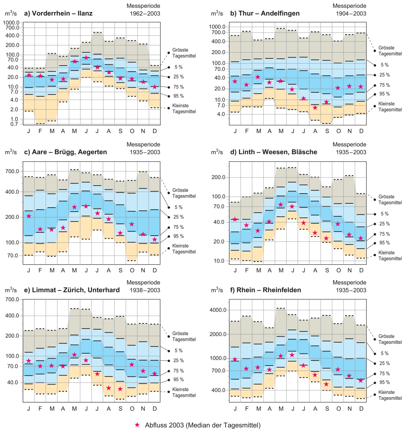
Abb. 3.5: Monatliche Verteilung der Tagesmittel des Abflusses von ausgewählten Flüssen mit Mischregime.
