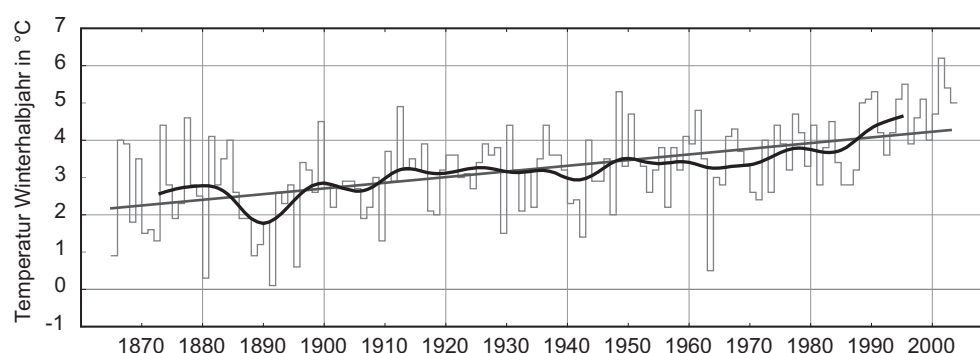
Abb. 1.2: Langjährige Temperatur- entwicklung des Winterhalb- jahres in den Niederungen der Alpennordseite (Mittel der Messstationen Basel, Bern, Genf und Zürich). Angegeben sind die Werte von Jahr zu Jahr, das Mittel über 20 Jahre (Gauss-Tiefpass-Filter) sowie der lineare Trend (graue Trendlinie). Deutlich ist der Sprung in der Erwärmung im Winterhalbjahr 1987/88 zu erkennen. Der lineare Trend der Erwärmung beträgt für die dargestellte Messreihe des Mittellandes +1,5 °C pro 100 Jahre.
