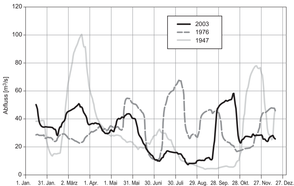
Abb. 3.10: Über 30 Tage gemittelte Abflussganglinie der Station Thur-Andelfingen in den Jahren 1947, 1976 und 2003. Jeder Wert gibt das Abflussmittel über die 14 vorgängigen und 15 nach- folgenden Tage inklusive des betreffenden Tages selbst an. Der 29.2.1976 wurde weggelassen.
