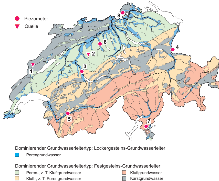
Abb. 5.1.: Hydrogeologische Übersicht der Schweiz und in diesem Bericht erwähnte Fallbeispiele:
