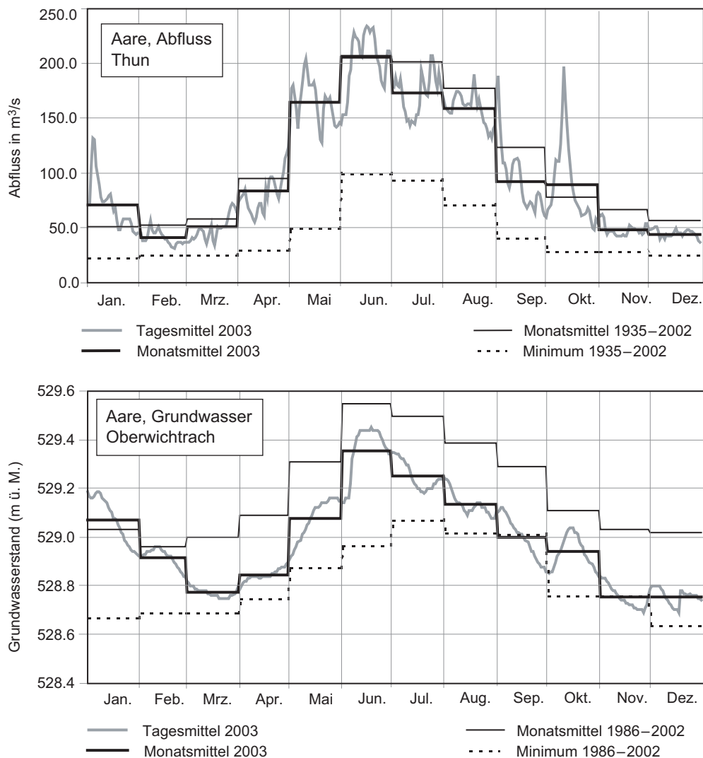
Abb. 5.5: Oben: Abfluss der Aare in Thun BE. Unten: Grundwasserstand in den Aareschottern in Oberwischtrach BE. (beides BWG-Messstationen)
