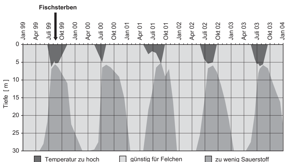
Abb. 4.3: Tiefenprofil des Greifensees im Kanton Zürich von Januar 1999 bis Januar 2004. In den dunkel eingefärbten Tiefen- bereichen ist die Wasser- temperatur für Felchen ent- weder zu hoch, oder es ist zu wenig Sauerstoff vorhanden. Wenn sich beide ungünsti- gen Bereiche überlappen, wird der Lebensraum für die Felchen eng. (Daten: AWEL Kanton Zürich).
