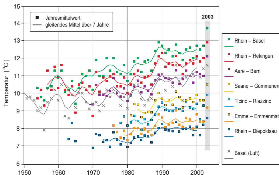
Abb. 4.1: Veränderung der Wassertemperatur an ausgewählten BWG-Messstationen seit 1950. Dargestellt ist zudem der Verlauf der Lufttemperatur in Basel (Daten: MeteoSchweiz).
