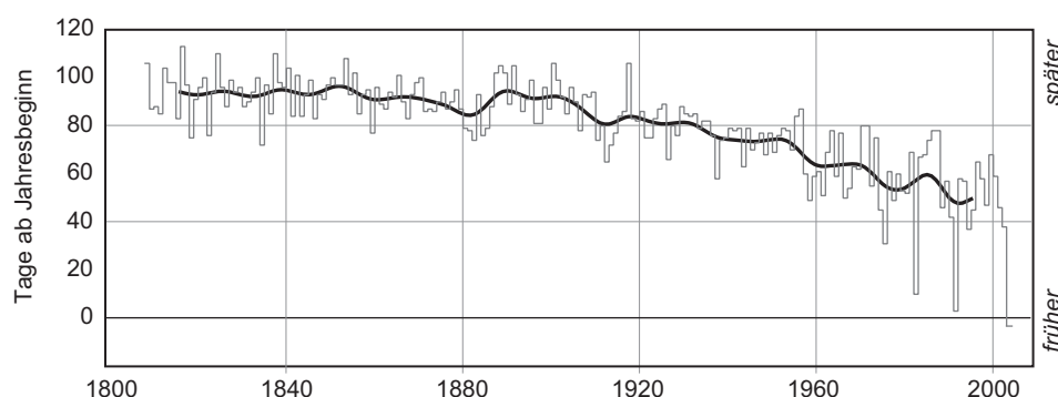
Abb. 1.1: Termin des Blattausbruchs der Rosskastanien in Genf. Gezählt werden die Tage seit Jahresbeginn. Die Messreihe (grau) beginnt 1808. Die schwarze Kurve zeigt die über 20 Jahre gemittelte Entwicklung (Gauss-Tiefpass-Filter). Der bisher späteste Blattausbruch wurde am 23. April 1816, der früheste am 29. Dezember 2002 beobachtet 3 .
