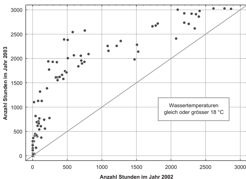
Abb. 4.8: Anzahl Stunden mit Wassertemperaturen über 18 °C an den 114 Mess- stationen (Punkte), aufge- tragen für die Jahre 2002 (X-Achse) und 2003 (Y-Achse). Stationen, bei denen sich zwischen diesen beiden Jahren nichts ver- ändert hat, würden auf die Diagonale (graue Linie) zu liegen kommen.
